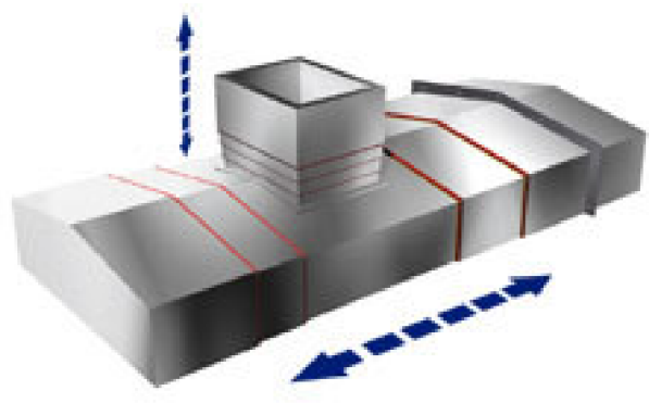
Obr.17 Dvousé kryty [7]
