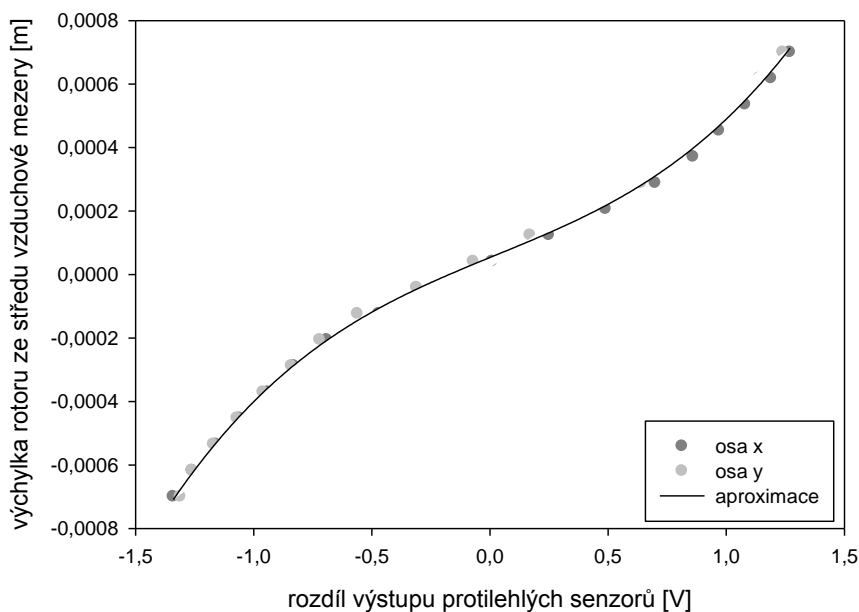
Obrázek 18: Závislost rozdílu výstupu senzorů na poloze rotoru
