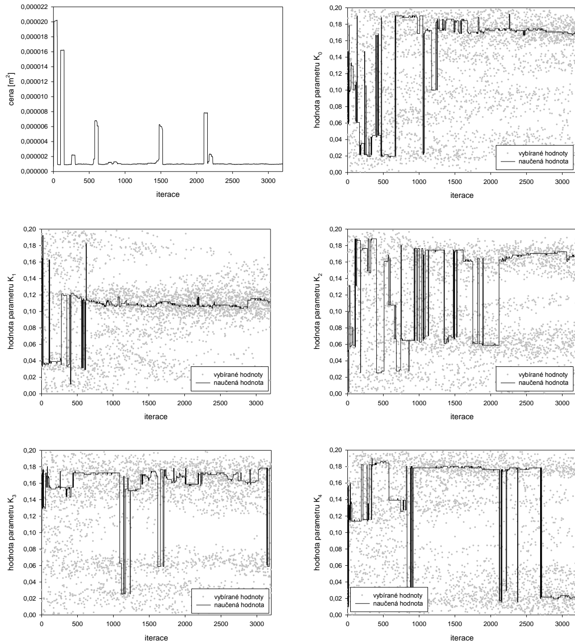
Obrázek 34: Průběh učení
