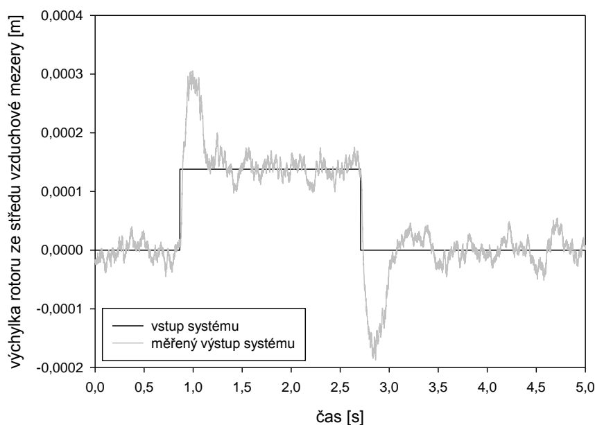
Obrázek 27: Data použitá pro identifikaci
