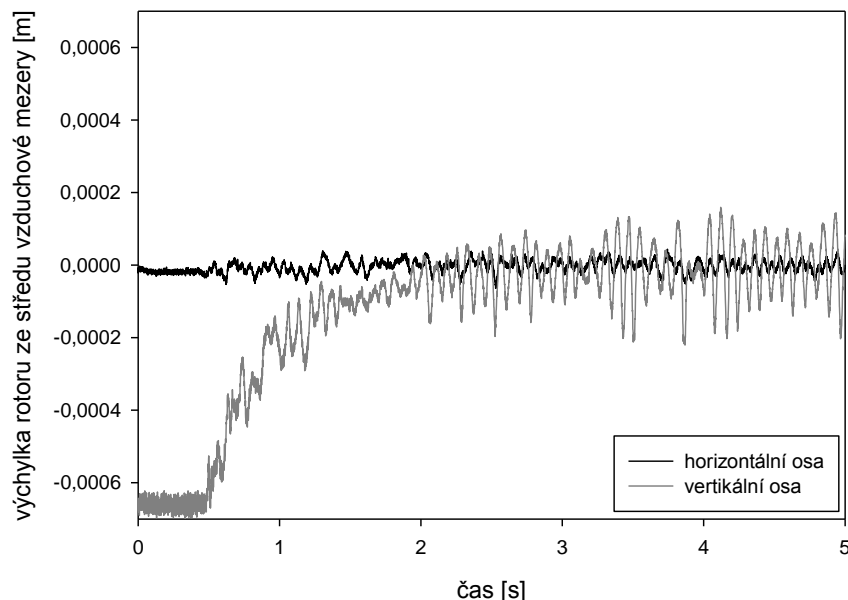
Obrázek 47: Chování aktivního magnetického ložiska řízeného LQ regulátorem
