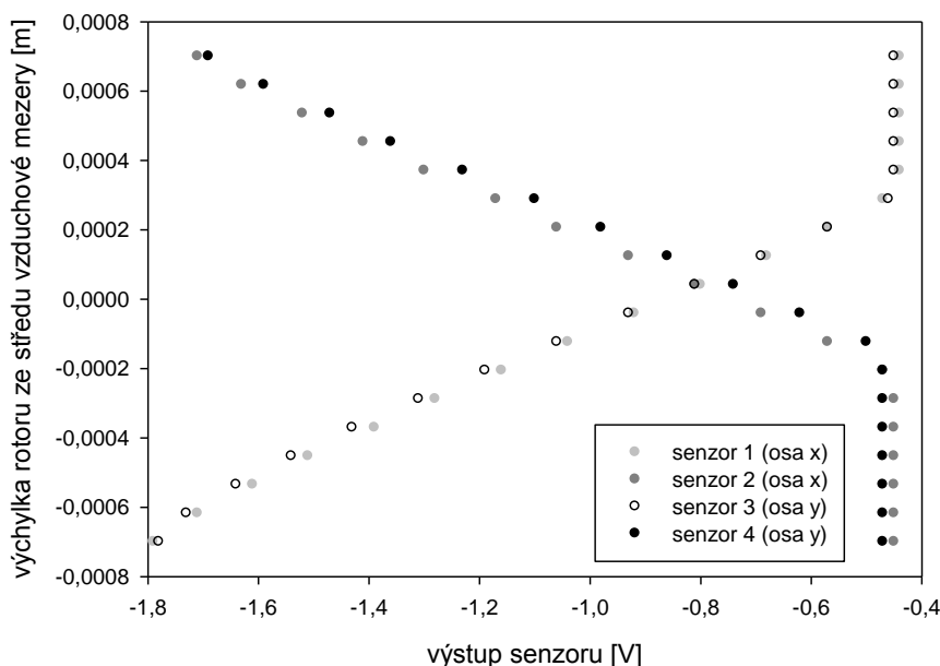
Obrázek 17: Závislost výstupu senzorů na poloze rotoru
