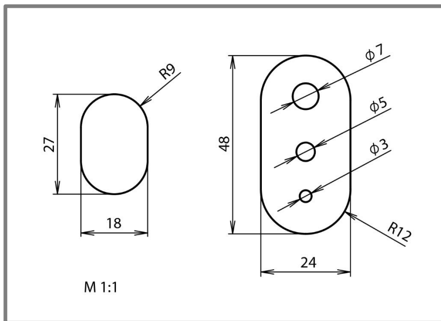
Obr. 6-11 Rozměry tlačítek
