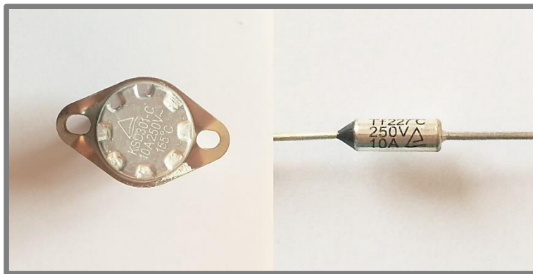
Obr. 2-12 Bimetalový spínač a tepelná nevratná pojistka
