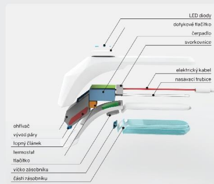
VNITŘNÍ SCHEMA
