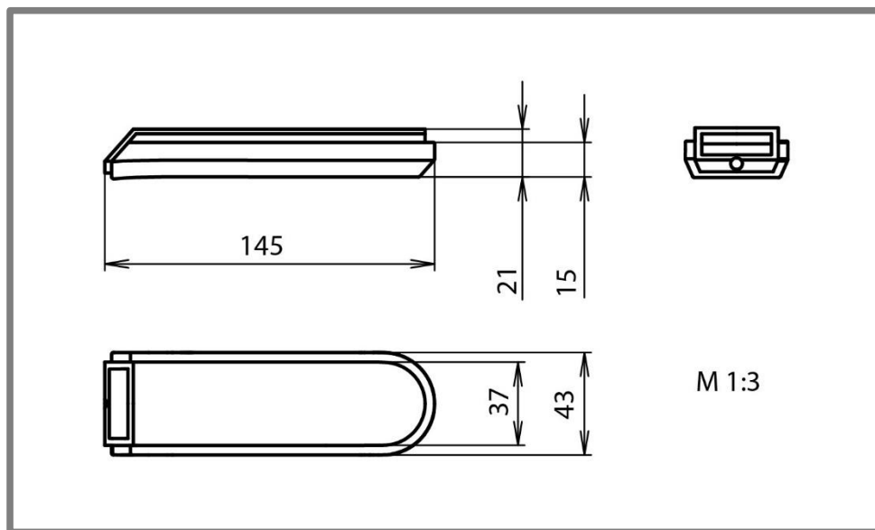
Obr. 6-8 Rozměry zásobníku
