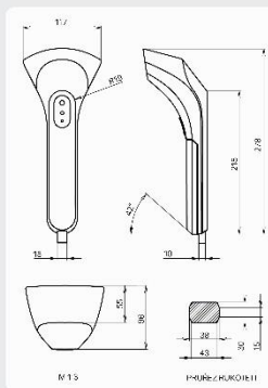
ROZMĚROVÉ ŘEŠENÍ
