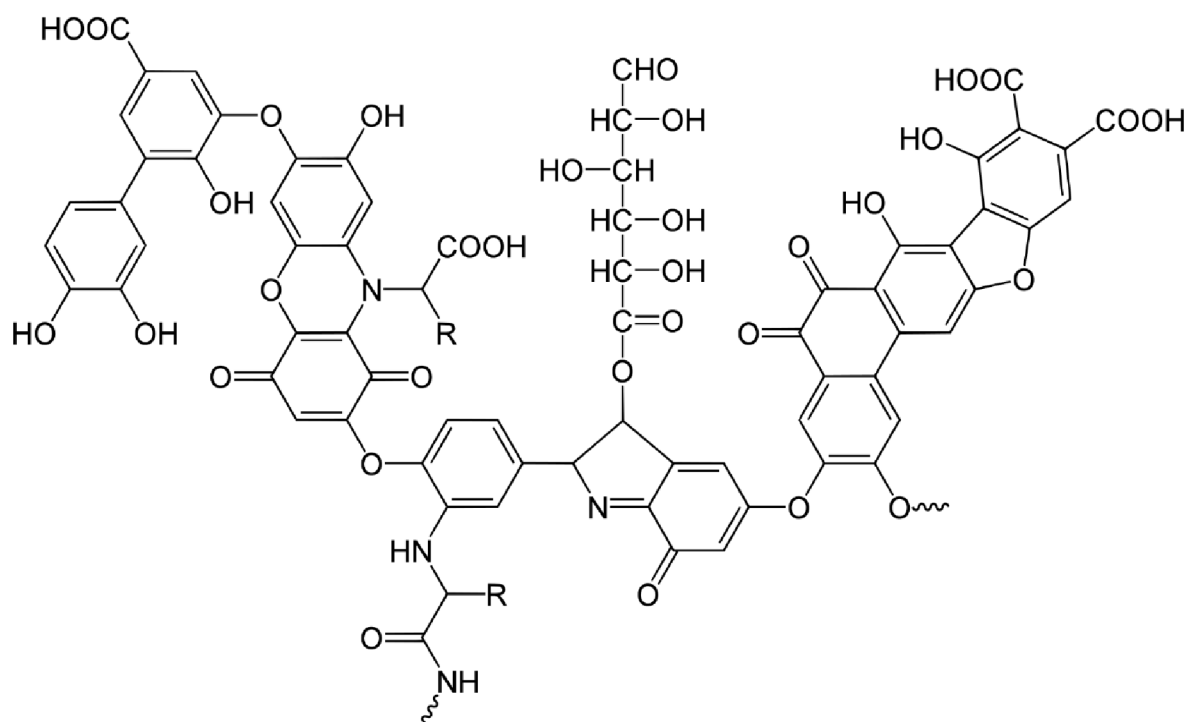
Obrázek 5 modelová struktura huminové kyseliny [32]
