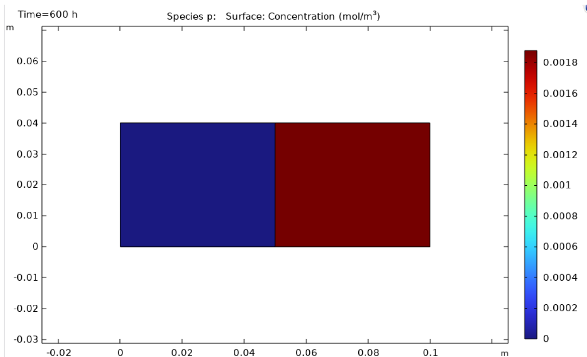
Výsledná koncentrace \xi koncentrace produktu v rovnováze při původní koncentraci barviva 0,08 g/l
