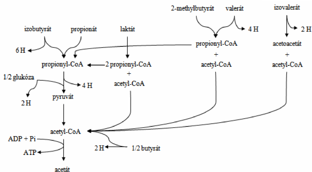
Obr. 11 Metabolismus organických kyselin za aerobních podmínek [32]
