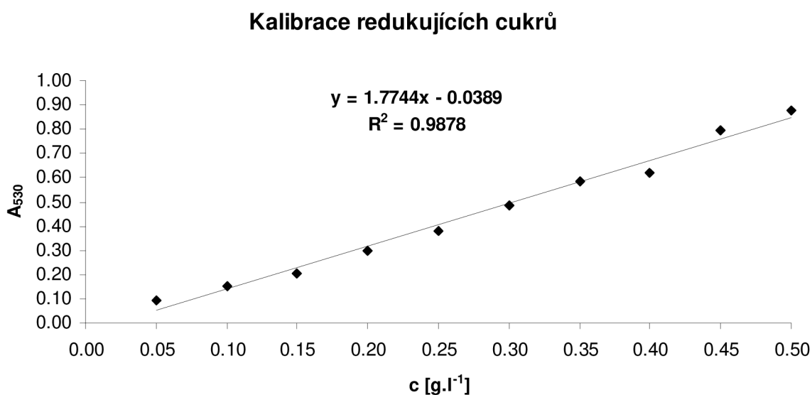
Graf 1 Závislost absorbance na koncentraci redukujících cukrů
