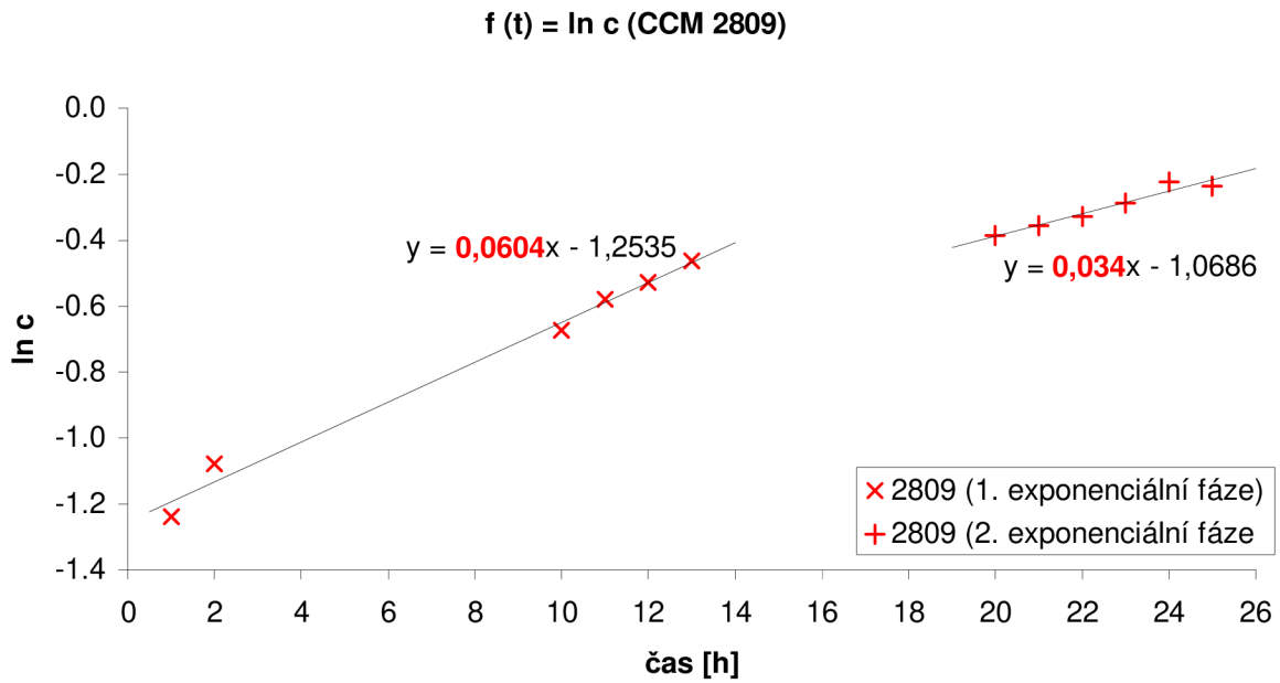
Graf 18 Linearizace koncentrace biomasy v exponenciálních fázích a výpočet měrné růstové rychlosti pro CCM 2809
