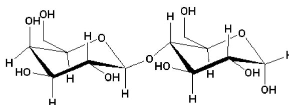
Obr. 2 Strukturní vzorec laktosy [15]
