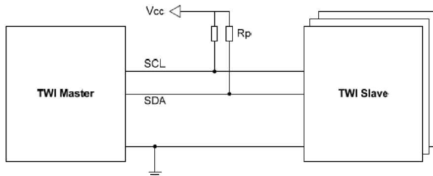
Obr. 2.3: Zapojenie dvojvodičovej zbernice [1]
