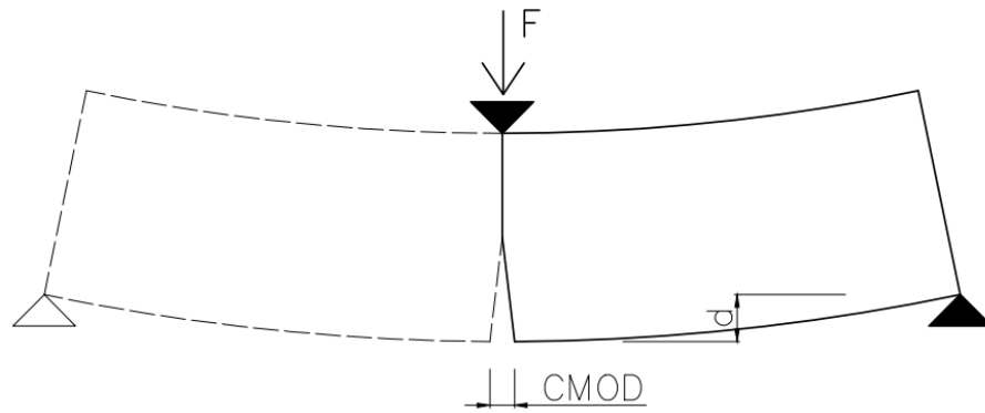
Obr. 2.6: Výstupní parametry
