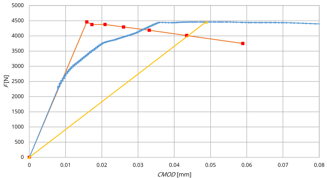
Obr. A.17: Betonové těleso P4_B45C45
