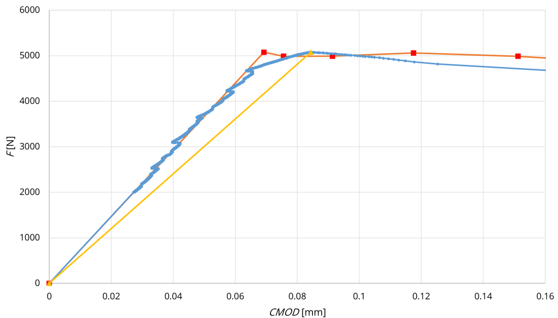
Obr. A.19: Betonové těleso P4_D62_X1
