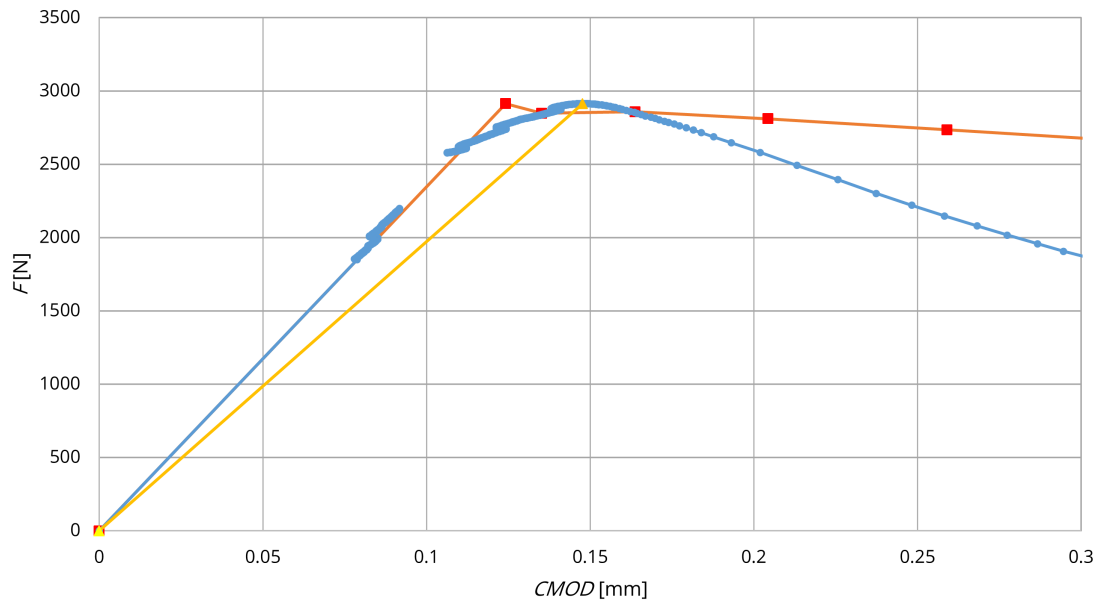
Obr. A.25: Betonové těleso P7_4EF
