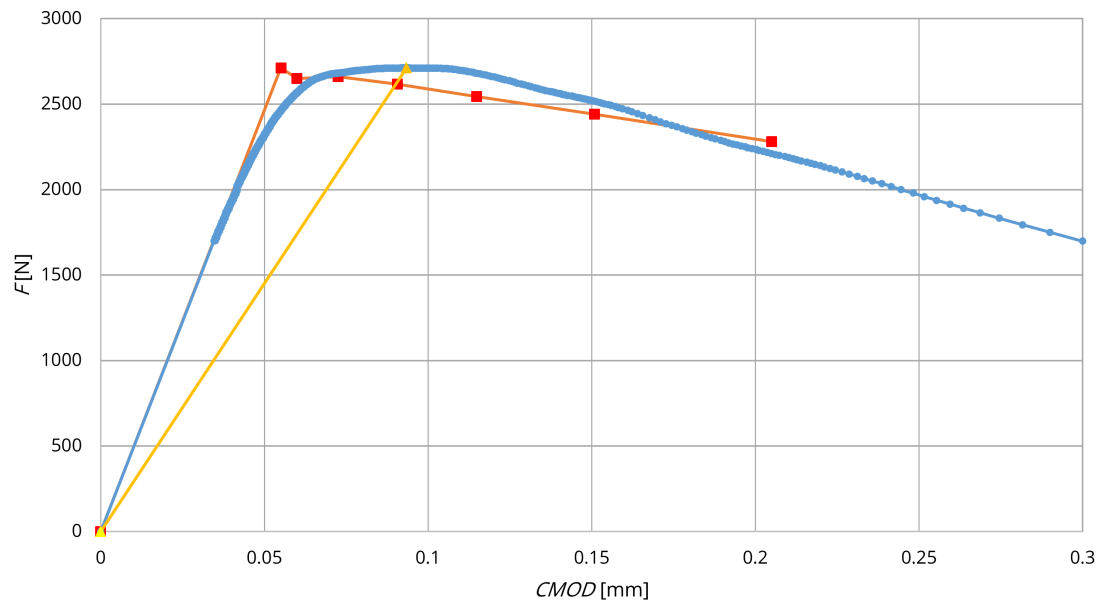
Obr. A.23: Betonové těleso P7_4BC
