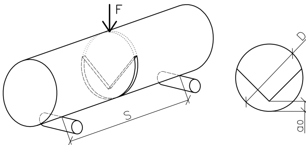
Obr. 1.5: Schéma testu válce se šípkovým vrubem v tříbodovém ohybu
