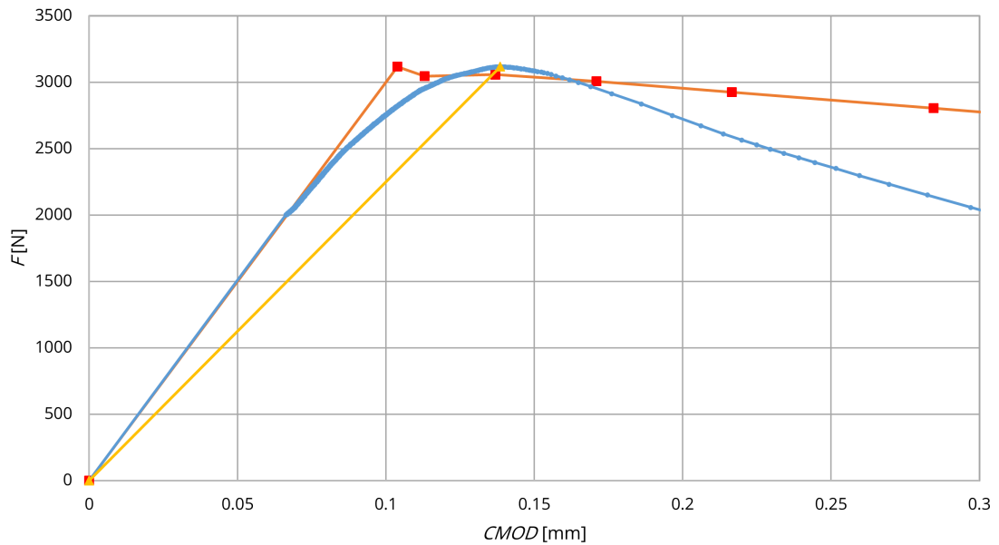
Obr. A.21: Betonové těleso P7_4FEE
