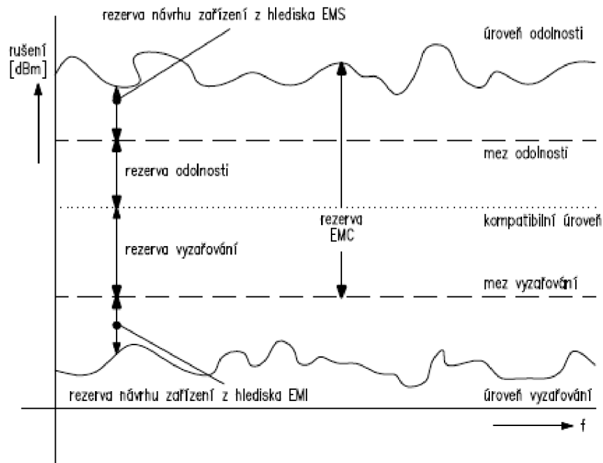
Obr. 3: Definice úrovní a mezí vyzařování a odolnosti
