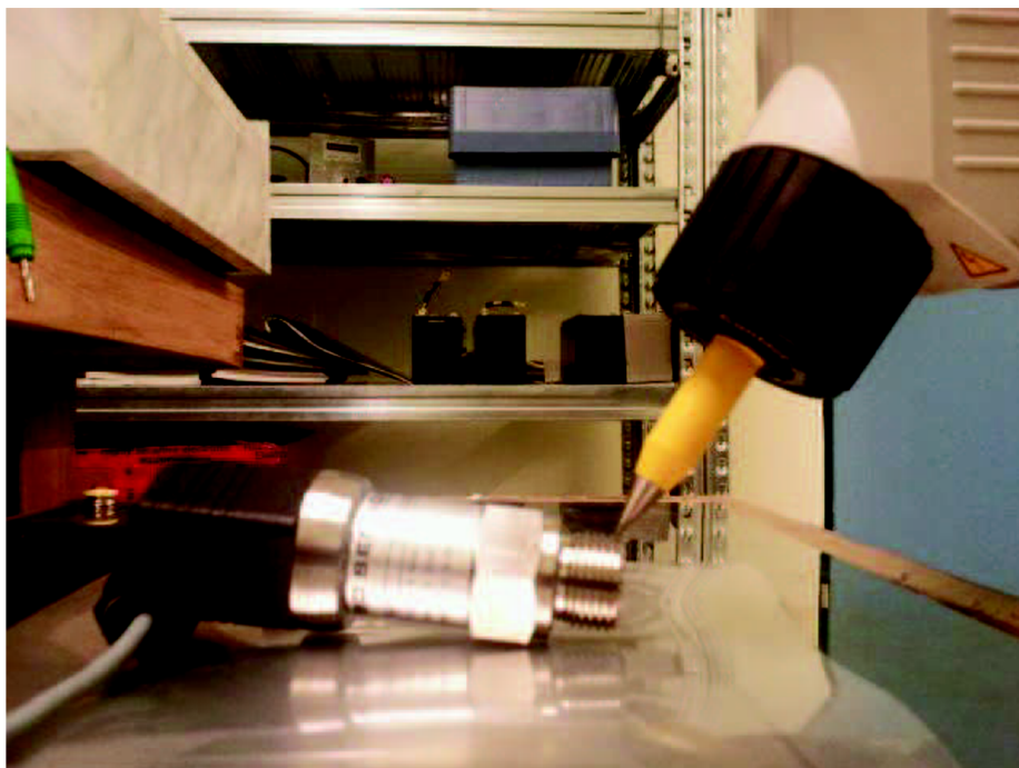
Obr. 24: Zkouška odolnosti proti elektrostatickému výboji na snímači DMP 331 (kontaktní výboj)
