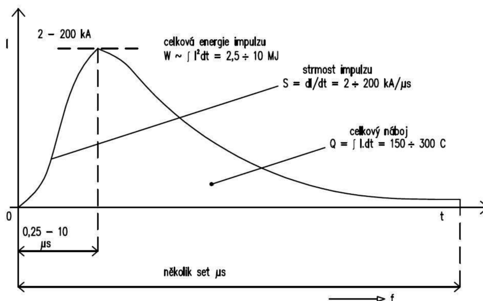
Obr. 6: Proudový impuls při výboji blesku a jeho parametry
