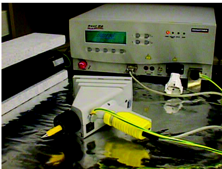
Obr. 7: Simulátor rušení BEST-EMC (Schaffner) se sondu pro elektrostatický výboj (ESD)
