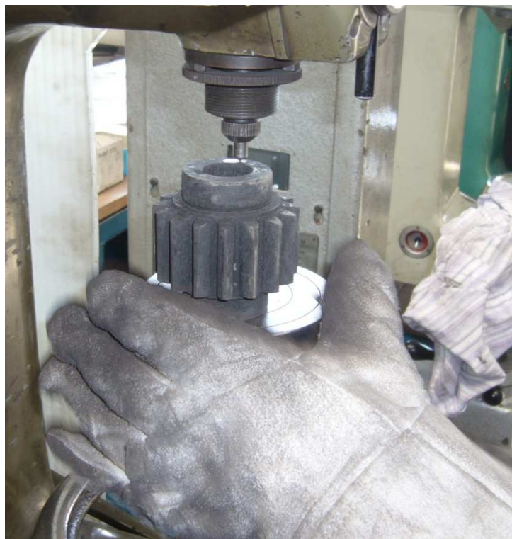
Obr. 3.3 Měření tvrdosti ozubeného kola
