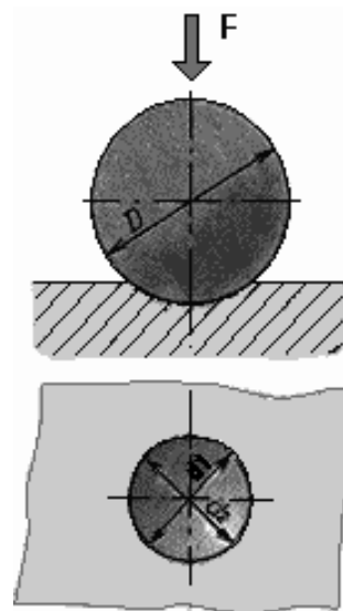
Obr. 1.1 Zkouška tvrdosti podle Brinella 8
