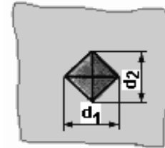
Obr. 1.2 Zkouška tvrdosti podle Vickerse 9
