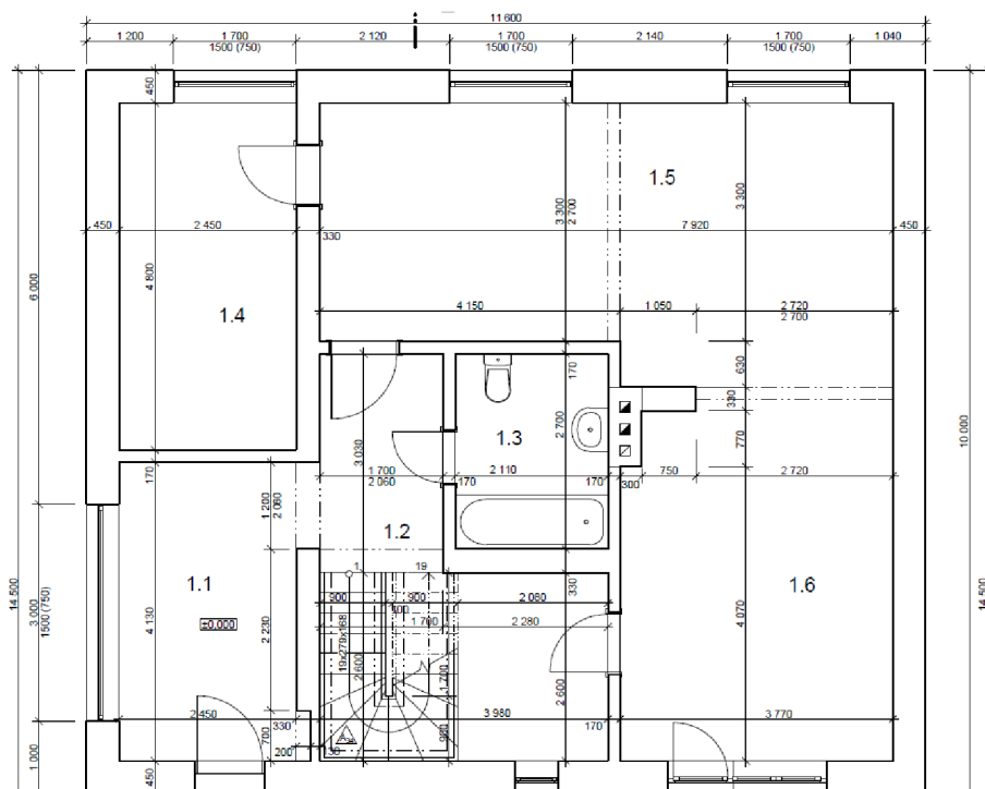
Obrázek 5.5 Půdorys [27]
