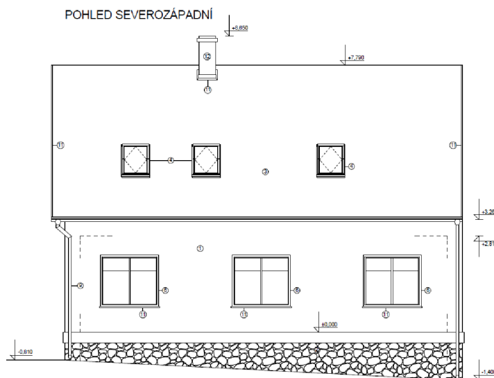
Obrázek 5.3 Severozápadní pohled [27]
