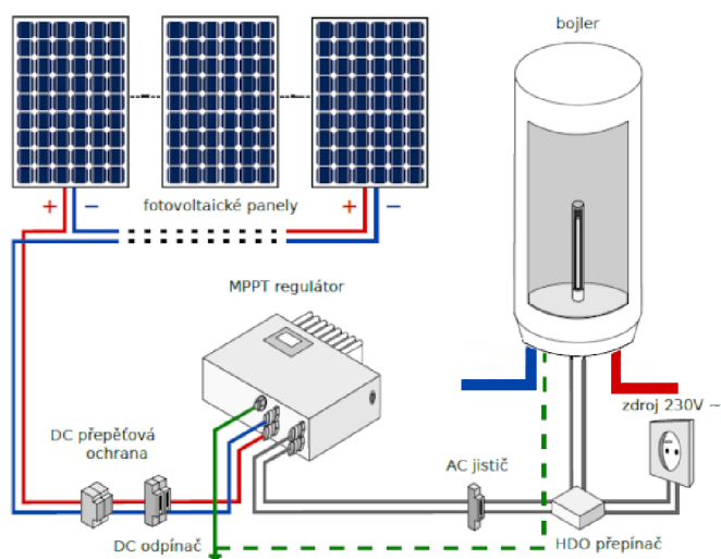
Obrázek 7.3 Kombinovaný systém s jednou spirálou a HDO [31]
