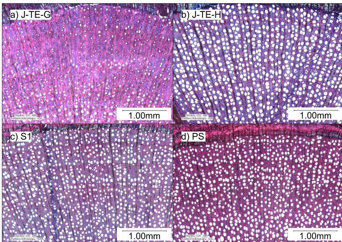
Obrázek 5: Detail xylému kořenů slabě (J-TE-G, S1) a silně (J-TE-H, PS) rostoucích podnožových kombinací jabloní a hrušní (kat.C1; Z: 26x), zdroj: autor
