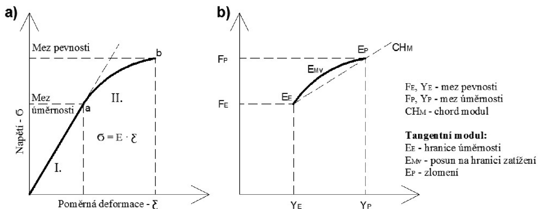
Obrázek 11 a) Napěťový deformační diagram; b) Plastická oblast (Gaff et al. , 2017a)
