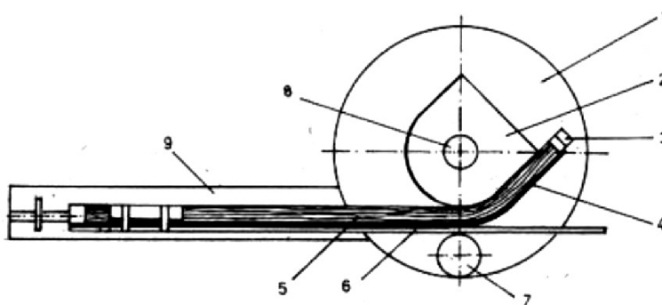
Obrázek 7 Schéma ohýbacího stroje s otočnou tvárnicí (Vinter, 2014)
