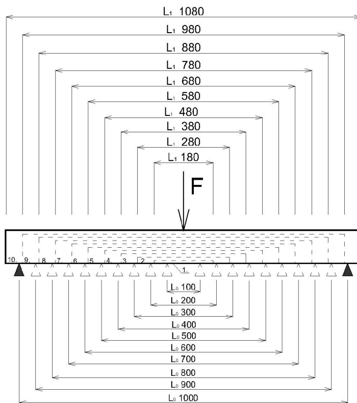
Obrázek 21 Schématické zobrazení třibodového ohybu (Autor)
