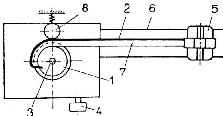
Obrázek 9 Ohýbací stroj k vytvoření uzavřených ohybů (Hlásková, 2018)
