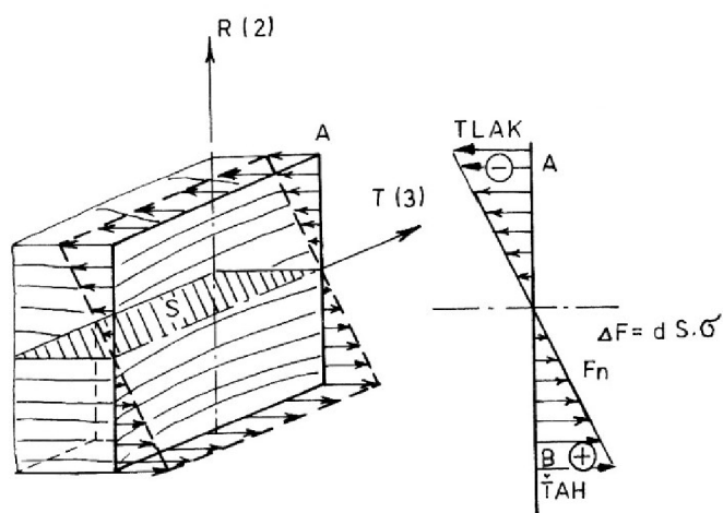
Obrázek 17 Napětí na výšku tělesa (Požgaj et al. , 1997).
