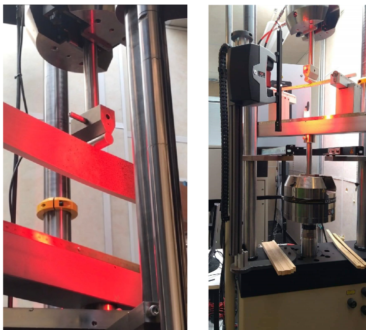
Obrázek 26 Trhací stroj Instron v procesu zkoušky (Autor)
