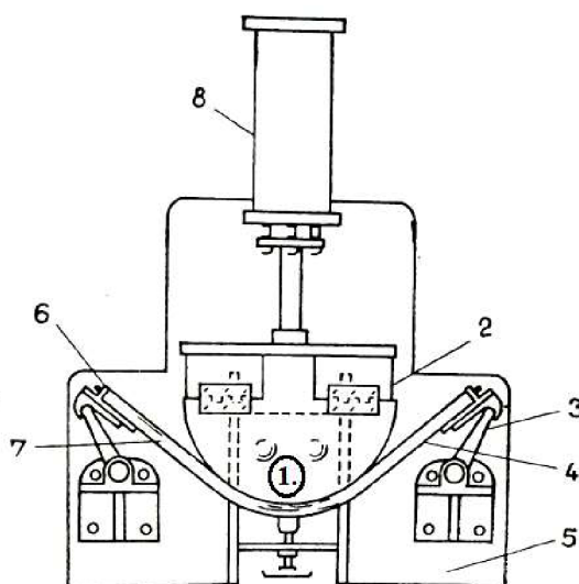
Obrázek 8 Rámová ohýbačka (Hlásková, 2018)
