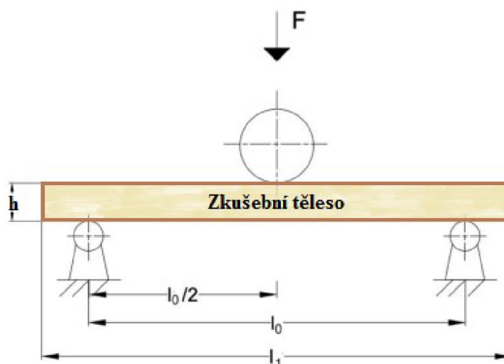
Obrázek 25 Schéma třibodového ohybu podle EN 310
