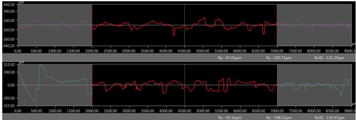
Obr. 4-8 Príklad vyhodnotenia drsnosti povrchu dvoch priamok na jednom prúte, pričom vyšedivená časť priebehu je spôsobená korekčným súčiniteľom \lambda_c
