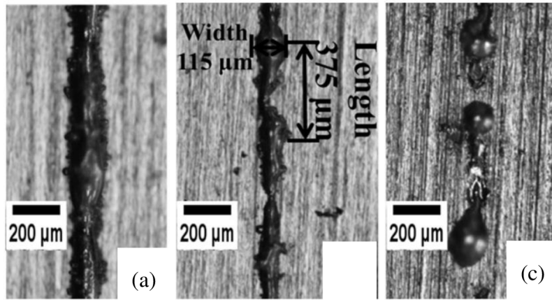
Obr. 2-6 Jednotlivé dráhy vyrobené pri výkone 170 W a rôznych skenovacích rýchlostiach: (a) Konzistentná, spojitá dráha (1100 mm/s), (b) Nekonzistentná, rozpadajúca sa dráha (2700 mm/s), (c) Dráha rozpadnutá na guľôčky (5500 mm/s) [10]
