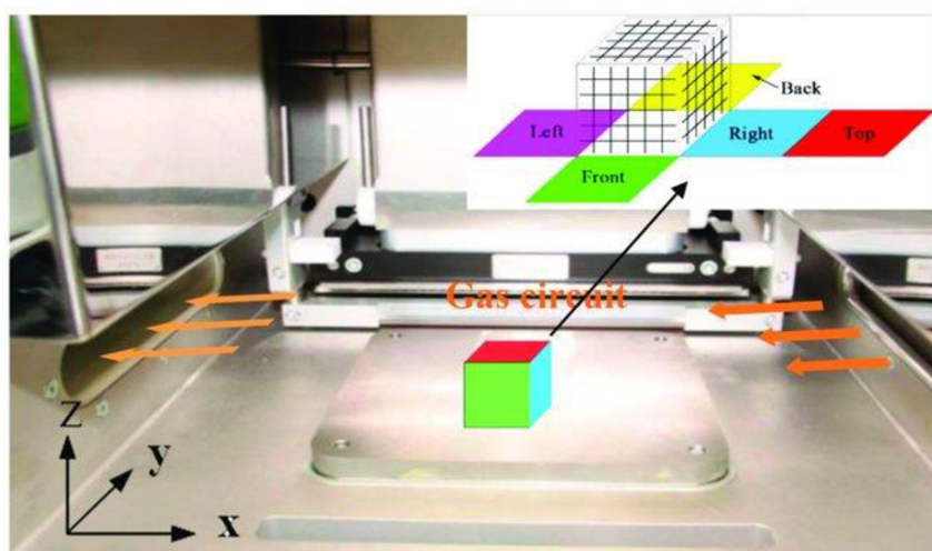
Obr. 2-14 Orientácia kocky vo výrobnéj komore a zvýraznenie smeru prúdenia atmosféry [11]
