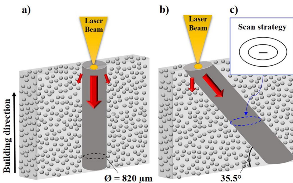
Obr. 2-19 Schematický nákres odvodu tepla prútov pod rôznymi uhlami sklonu: (a) Vertikálny prút (uhol sklonu 90°), (b) Prút s uhlom sklonu 35,5°, (c) Skenovacia stratégia použitá na výrobu prútov [13]
