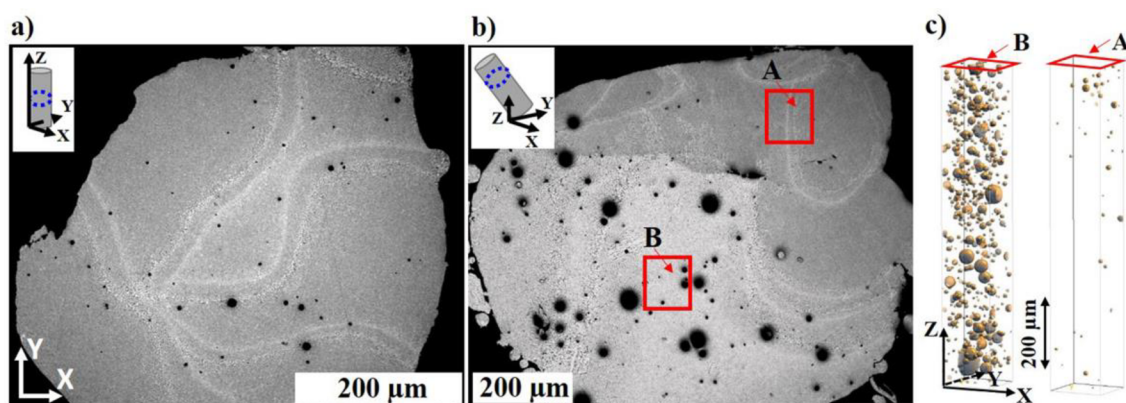
Obr. 2-20 Porovnanie mikroštruktúry a porozity v reze pre prúty s rôznymi uhlami sklonu: (a) Vertikálny prút (uhol sklonu 90^\circ ), (b) Prút s uhlom sklonu 35,5^\circ , (c) Porovnanie porozity dvoch rôznych zón v prúte so sklonom 35,5^\circ [13]
