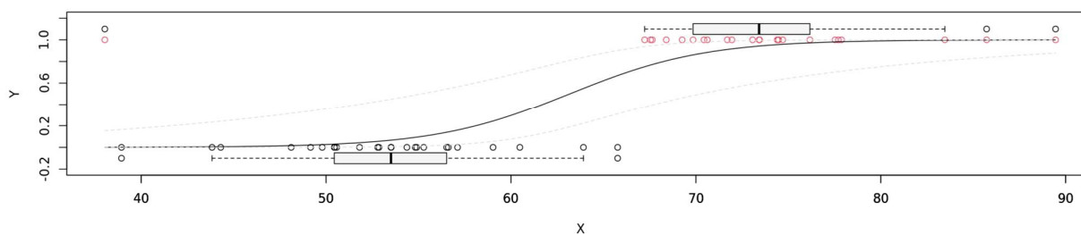
Graf č. 2: Ilustrativní graf výsledků logistické regrese
