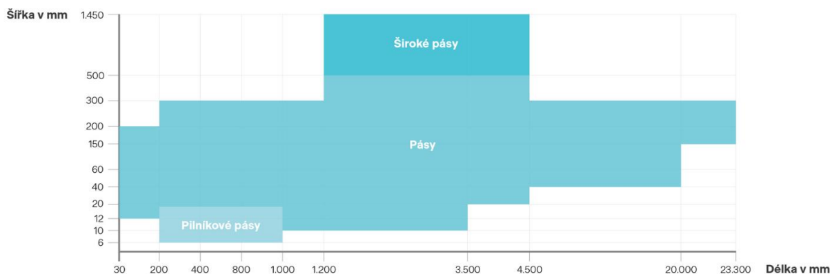
Obr. 16 Klasifikace brusných pásů [11]
