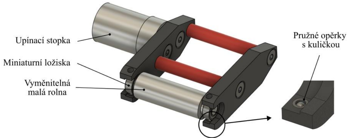
Obr. 43 Konstrukční řešení sady malých broušicích roln s držákem
