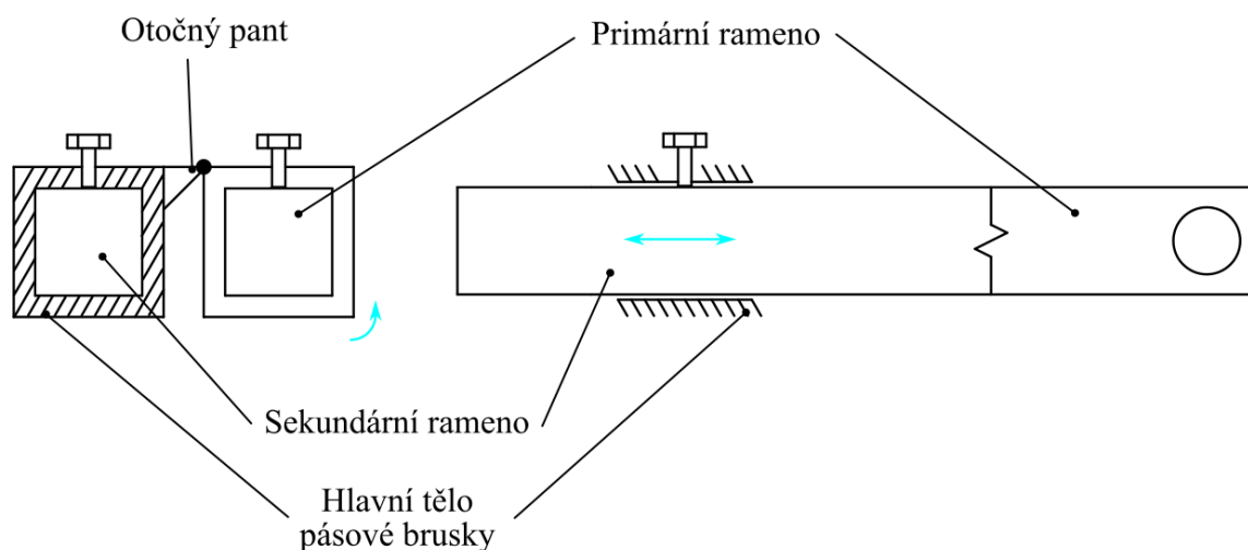
Obr. 19 Uspořádání výsuvných ramen – varianta 3
