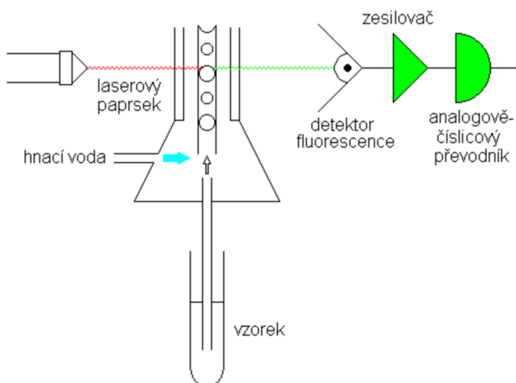
Obr. č. 11: Průtoková cytometrie
