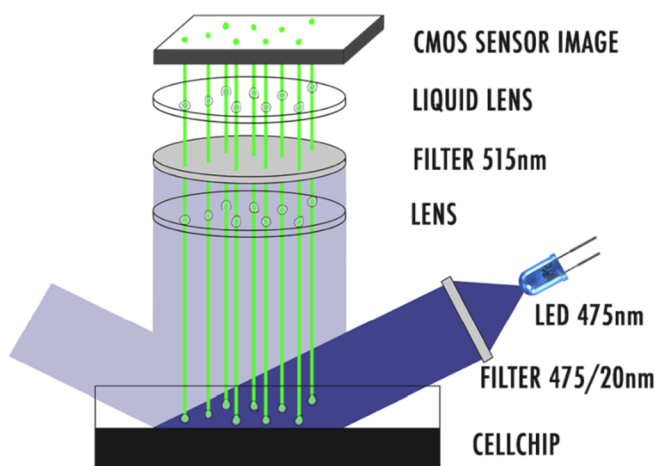
Obr. č. 14: Princip fluorescenční obrazové cytometrie Zdroj: online obrázek č. 14
