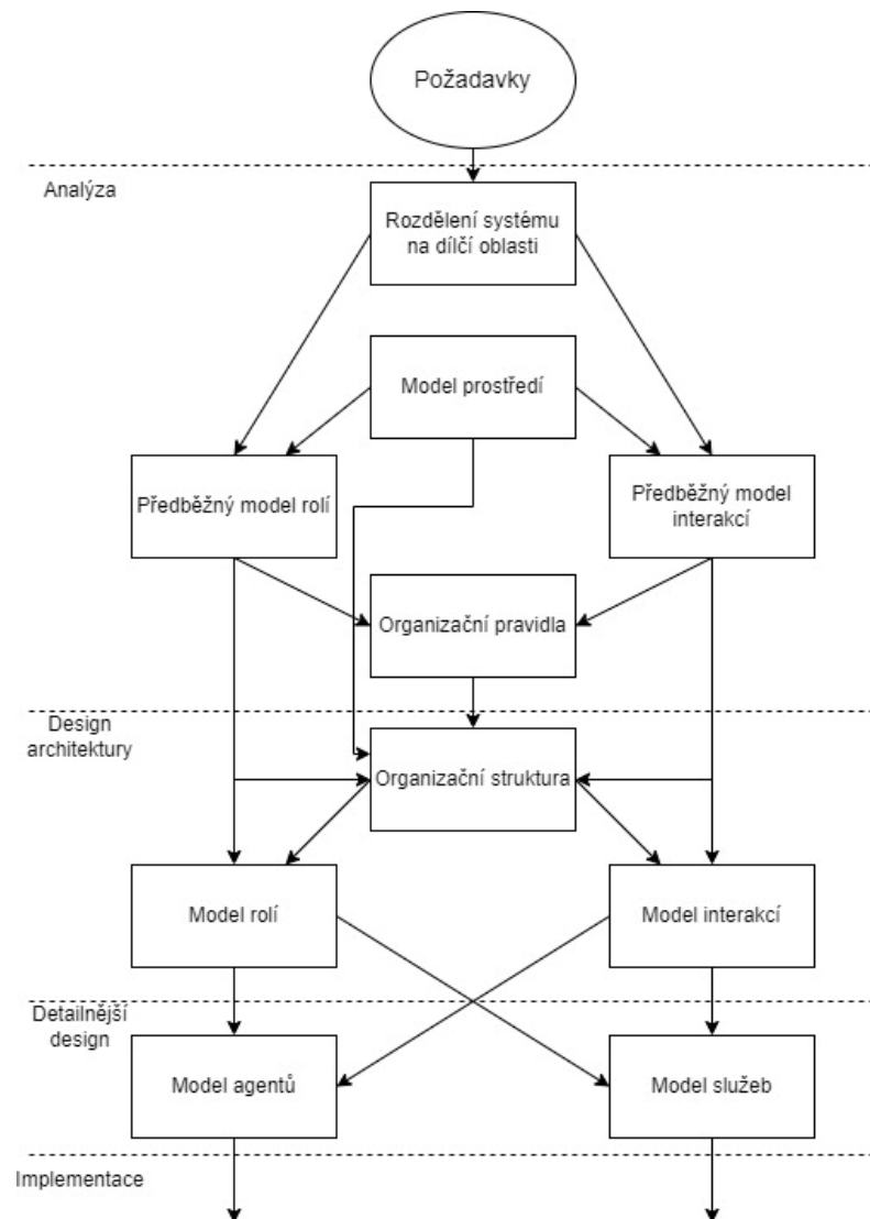
Obrázek 4: Struktura GAIA, volné zpracování autorky dle (Wooldridge, 2000)
