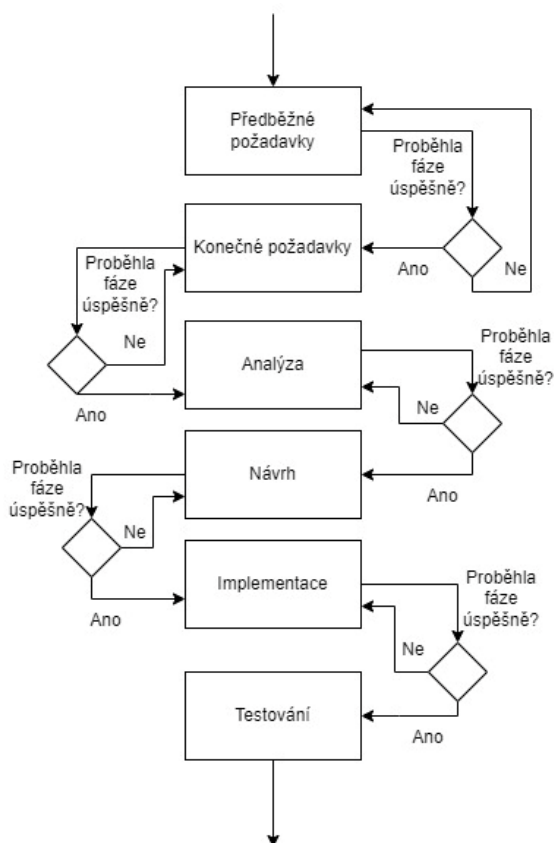
Obrázek 3: Struktura ADELFE, volné zpracování autorky dle (Mefteh, 2015)
