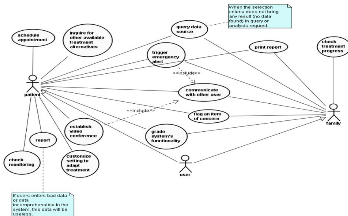
Obrázek 17: Kooperace entit v ADELFE v rámci případové studie (Yu, 2002)
