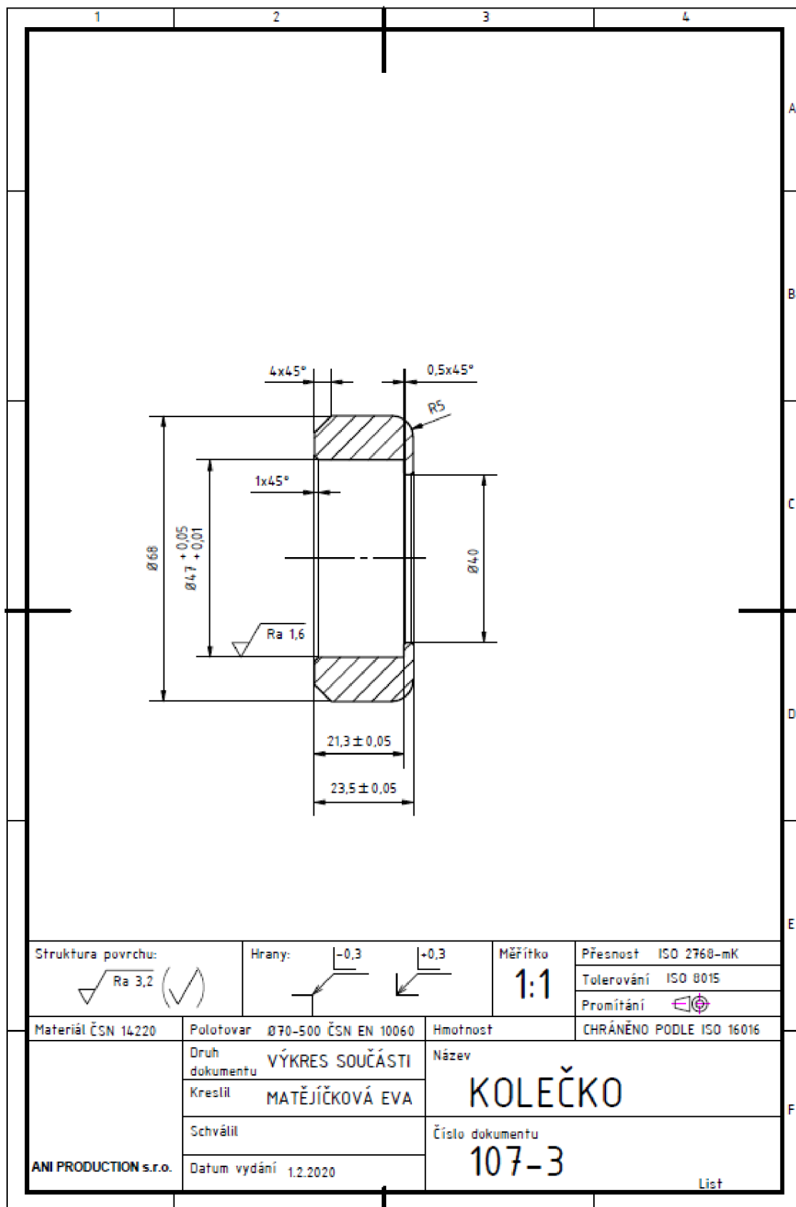
Výkres 1073 – kolečko
