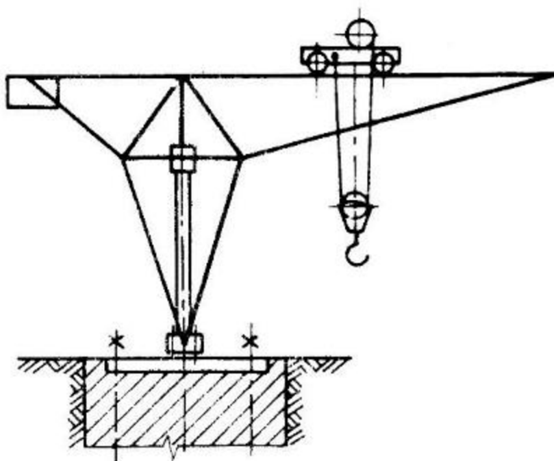
Obr. 9 Věžový jeřáb. [7]
