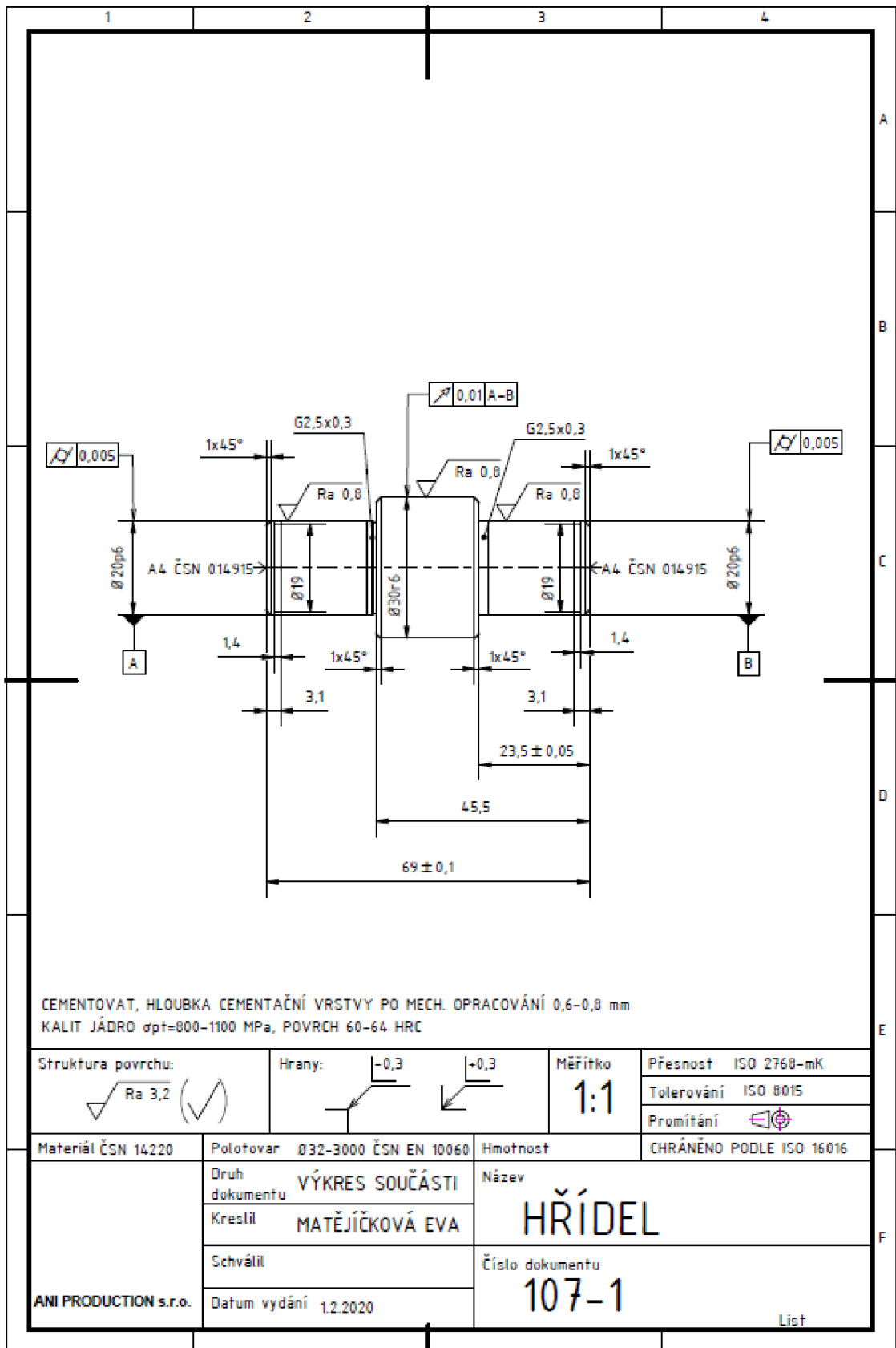
Výkres 1071 – hřídel
