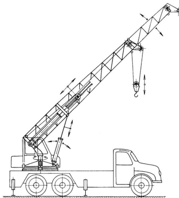
Obr. 11 Automobilový jeřáb.
