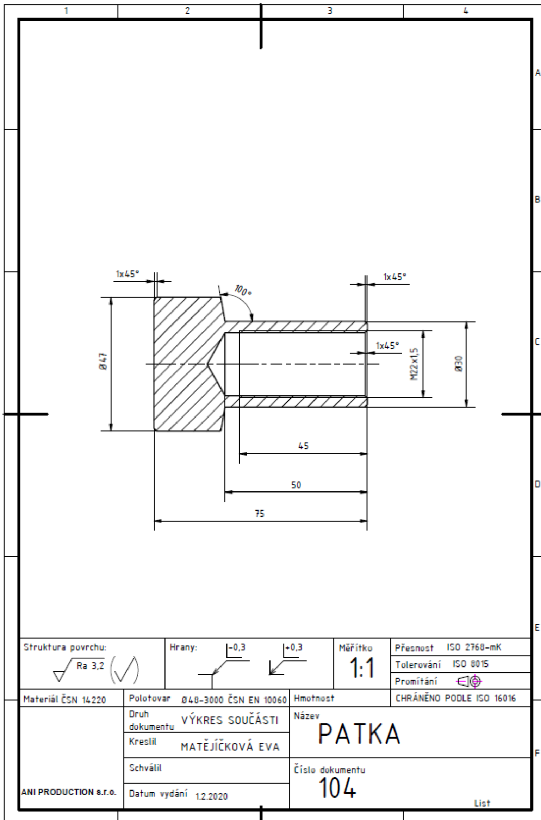
Výkres 104 – patka
