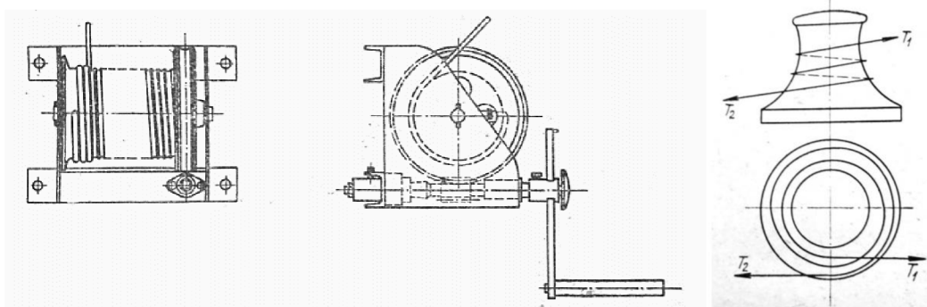
Obr. 4 Klikový naviják a posunové vrátka. [2]
