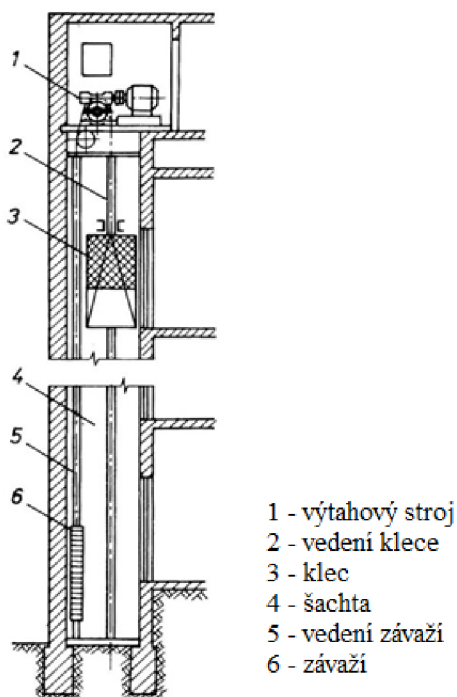
Obr. 13 Výtah. [8]
