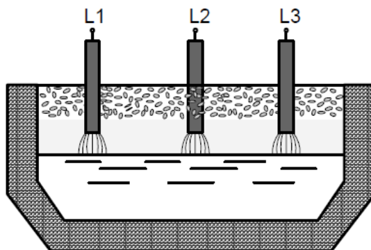
Obr. 4) Pec se zakrytým obloukem [7]
