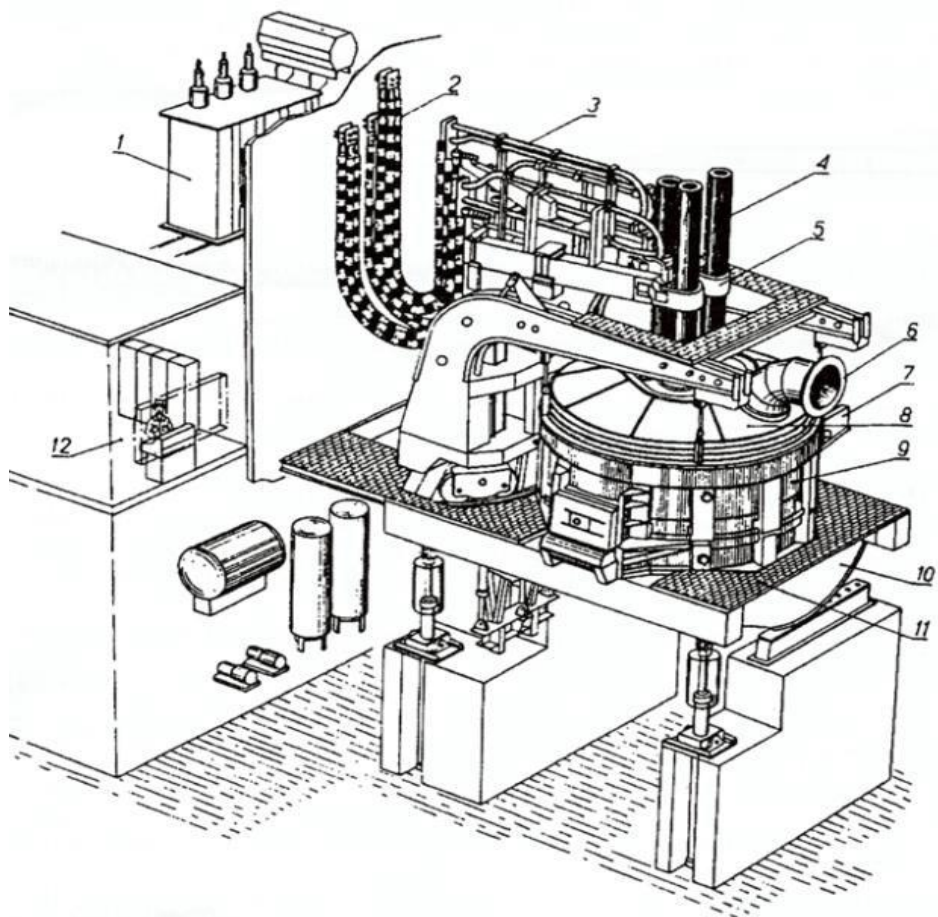
Obr. 1) Schematické zobrazení třífázové EOP [3]
