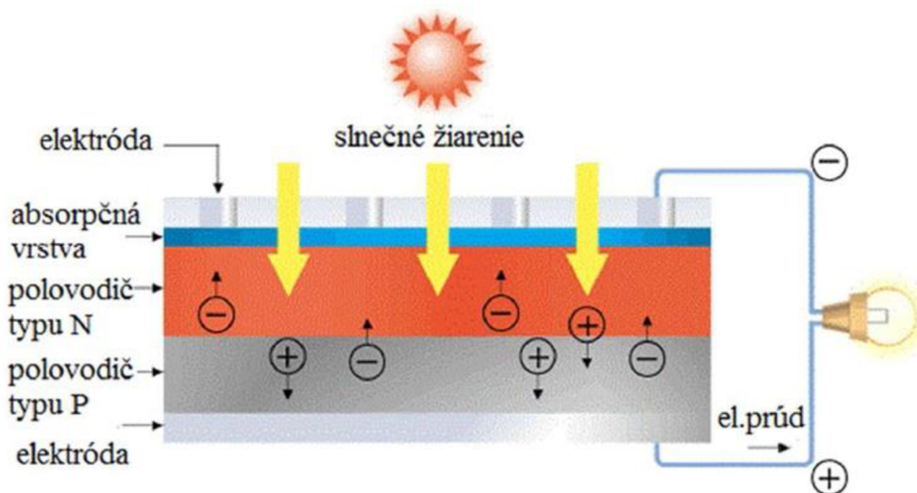
Obr. 10.4 Schéma principu fotovoltaických systémů (33)
