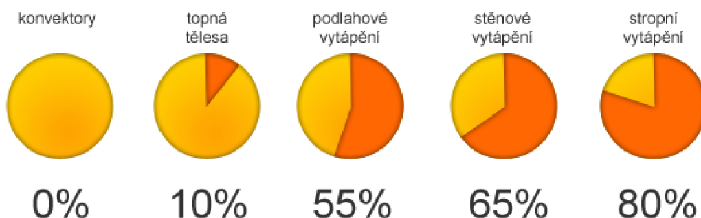
Obr. 8.4 Podíl tepelného toku sáláním pro různé druhy vytápění (24)
