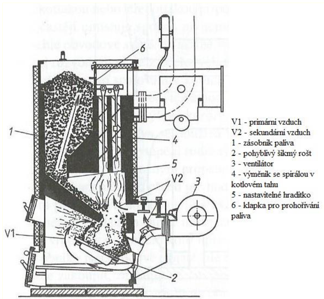
Obr. 6.7 Kotel s přetlakovým spalováním (16)
