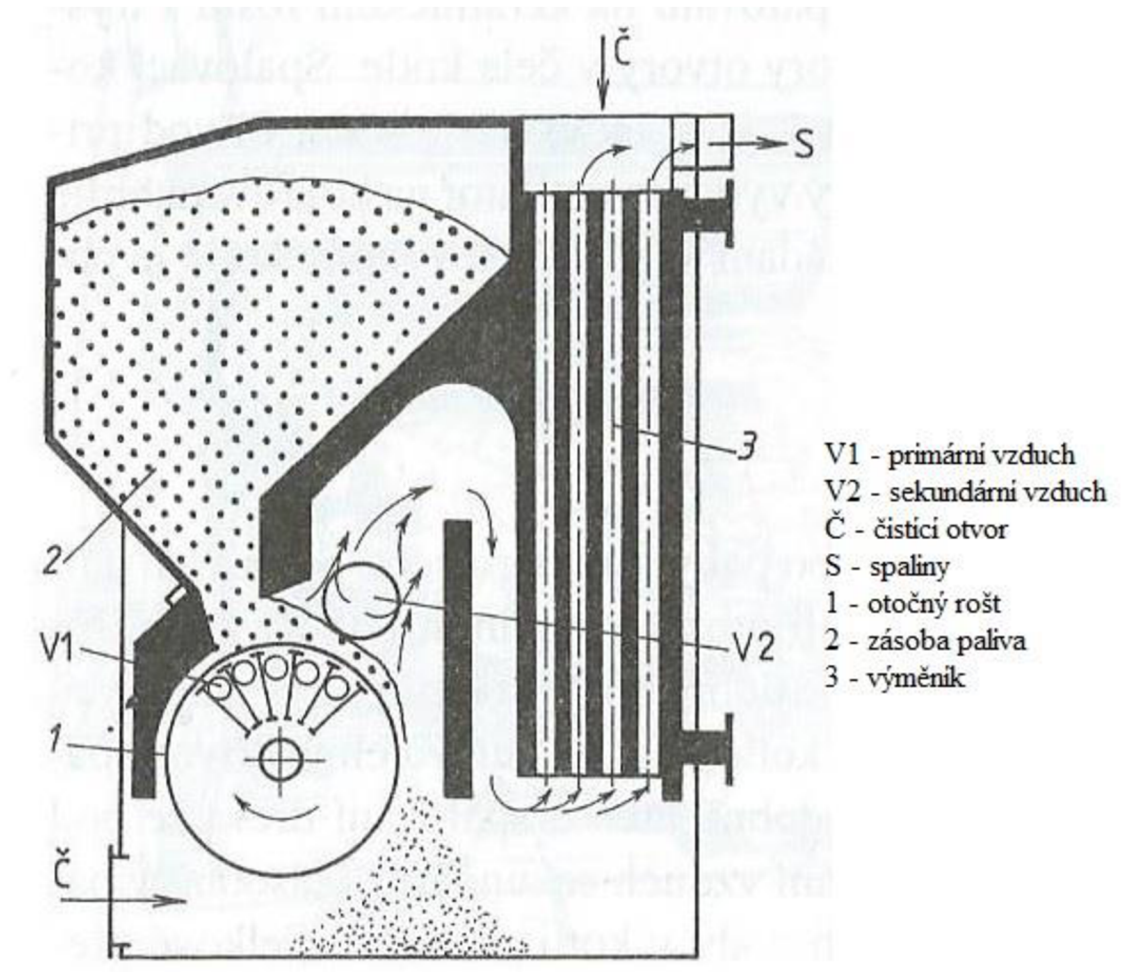
Obr. 6.6 oteel s pohyblivým roštem (15)
