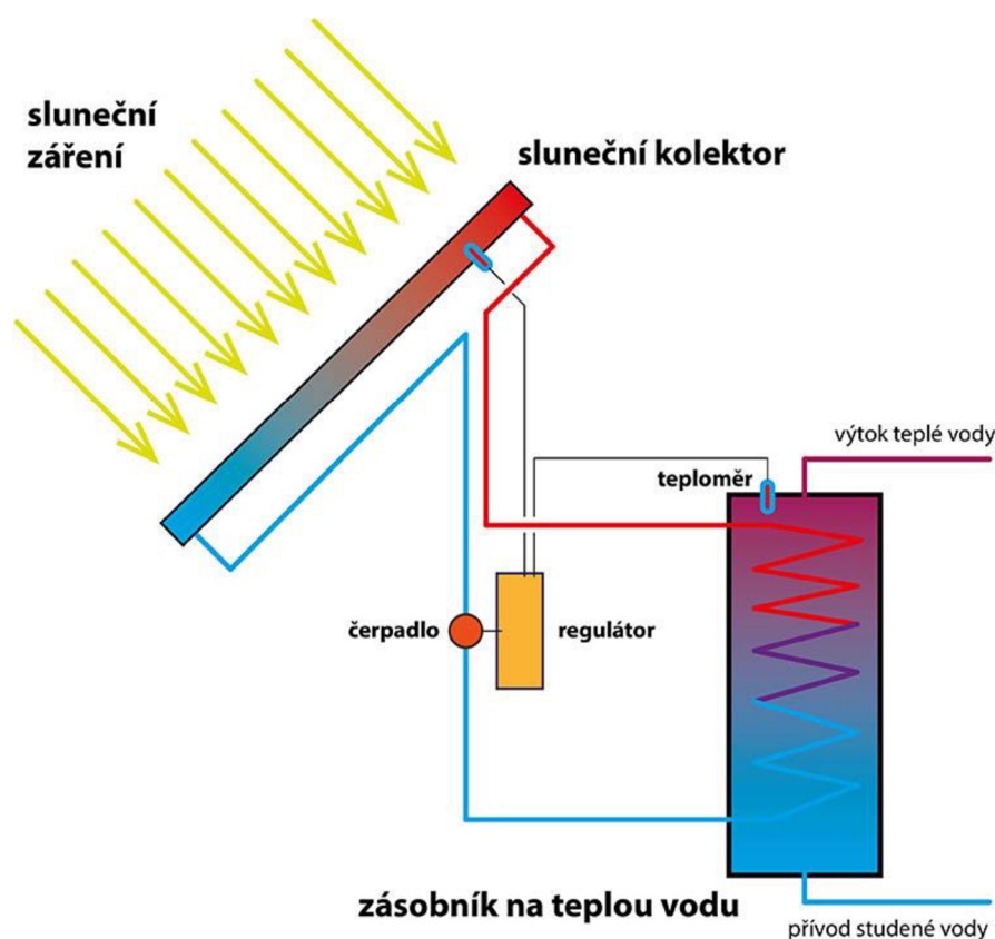
Obr. 10.1 Schéma principu fototermického systému (30)
