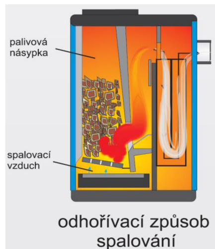
Obr. 5.6 Odhořivací kotel (7)
