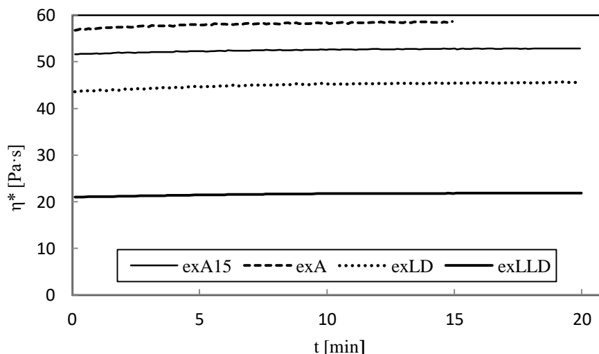
Obr. 23 Křivka testu stability vybraných vzorků směsí exA a exA15 a obou referenčních složek
