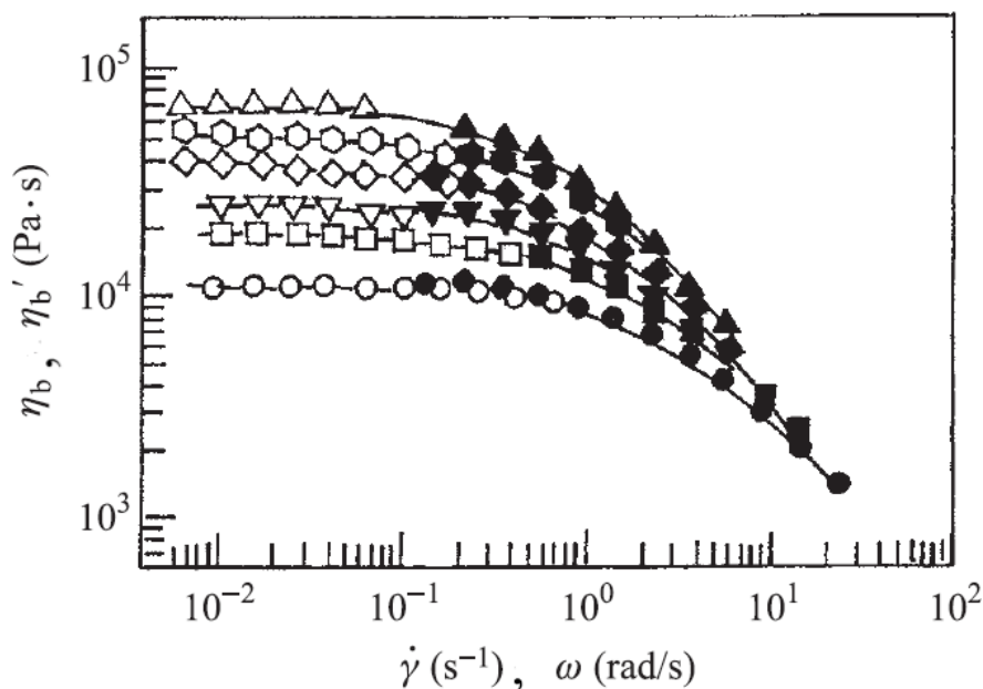
Obr. 16 Graf sestavený dle Cox-Merzova pravidla pro taveniny směsí PMMA/PVDF (vyplněné symboly značí data z oscilačního měření, prázdné symboly značí data ze smykového měření) [9]
