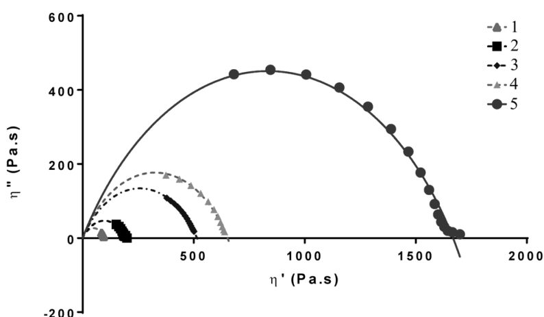
Obr. 12 Cole-Cole grafy pro vzorky PLA, které byly vystaveny působení UV záření po různě dlouhou dobu [17]
