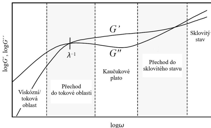
Obr. 11 Průběh závislostí G' a G'' na \omega (logaritmické měřítko) [4]
