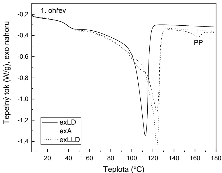
Obr. 19 Křivky prvního ohřevu vzorků filmů vylisovaných z extrudovaného granulátu LD, A a LLD; PP značí pík tání polypropylénu u vz. exA
