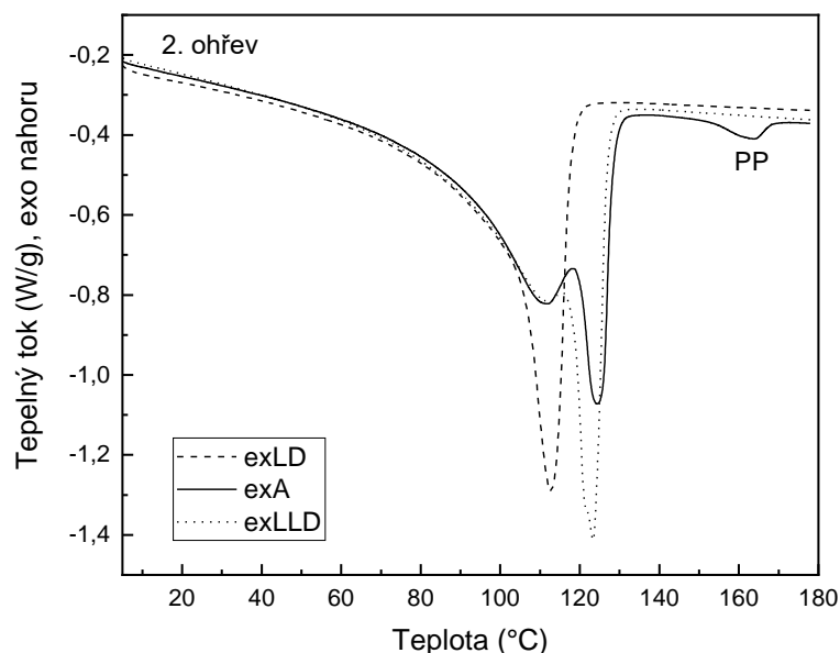
Obr. 21 Křivky druhého ohřevu vzorků filmů vylisovaných z extrudovaného granulátu LD, A a LLD; PP značí pík tání polypropylénu u vz. exA
