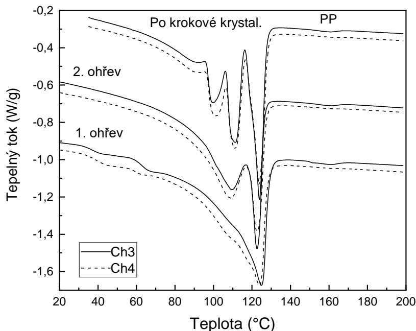
Obr. 18: Křivky prvního a druhého ohřevu vzorků regranulátu Ch3 a Ch4 a křivky ohřevu po izotermické krokové krystalizaci; PP značí pík tání polypropylénu (intenzivnější pík a tudíž větší množství je ve vz. Ch3)
