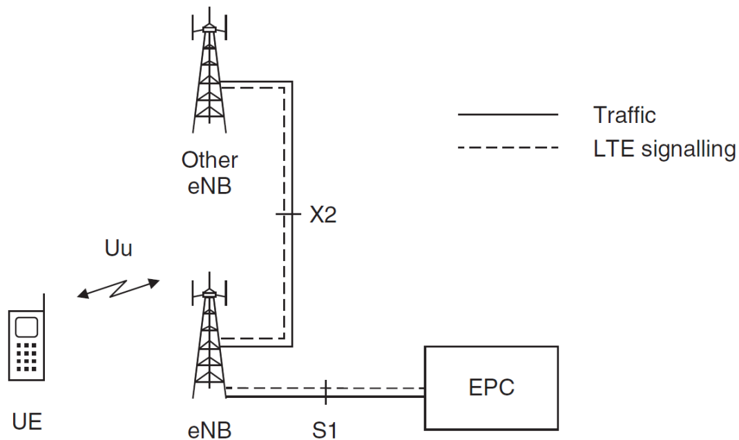
Obr. 1.2: Architektúra E-UTRAN [1]
