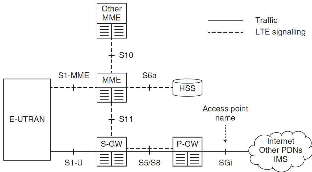
Obr. 1.3: Architektúra EPC [1]
