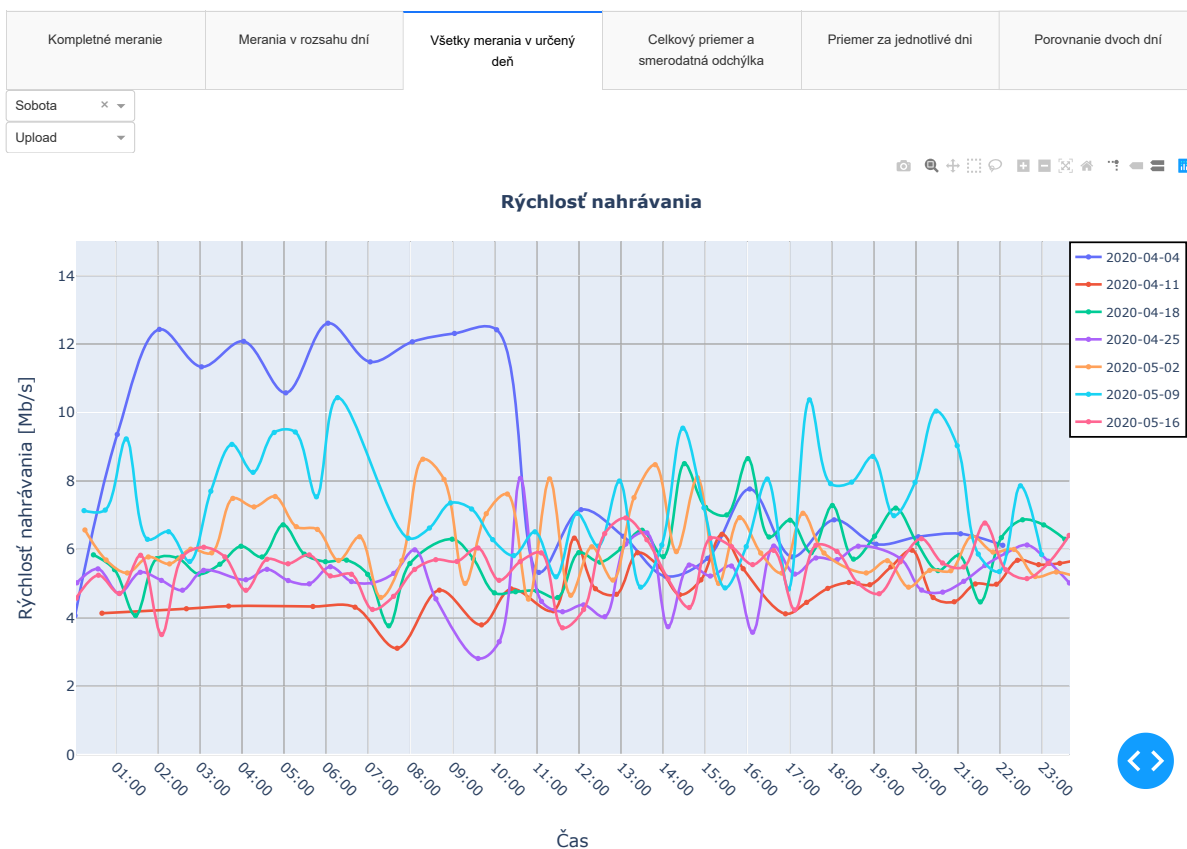
Obr. 5.1: Grafické prostredie pre zobrazovanie grafov
