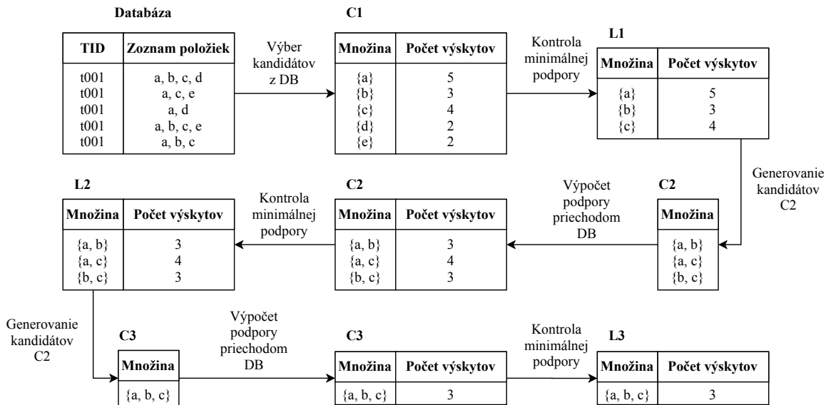
Obr. 3.1: Algoritmus Apriori
