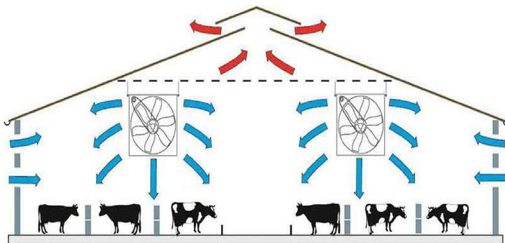
Obrázek č. 3. Proudění vzduchu
