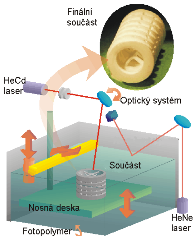
Obr. 1.2 Schéma stereolitografie [5]
