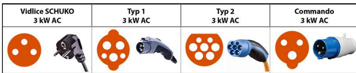
Obrázok 4 Typy konektorov pre pomalé nabíjanie [15]
