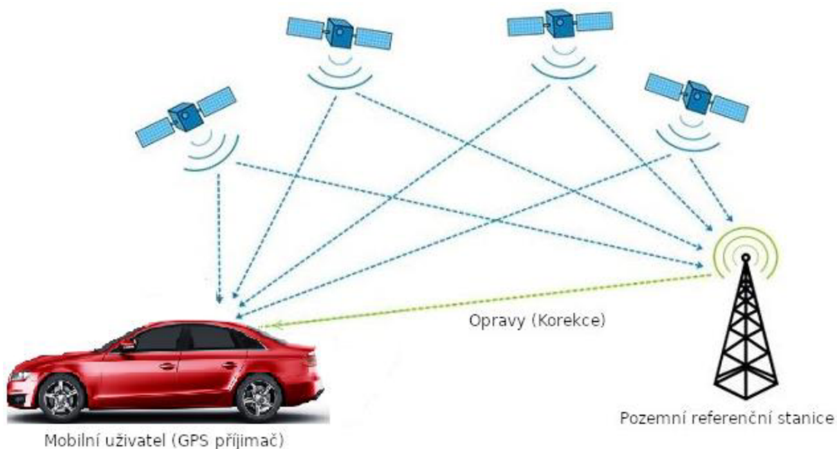
Obr. 23 Princip fungování diferenciální GPS (upraveno) [64]
