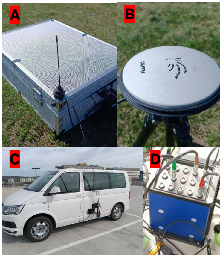
Obr. 35 A) Anténa, B) Satelit, C) Experimentální vozidlo, D) ADMA ve vozidle
