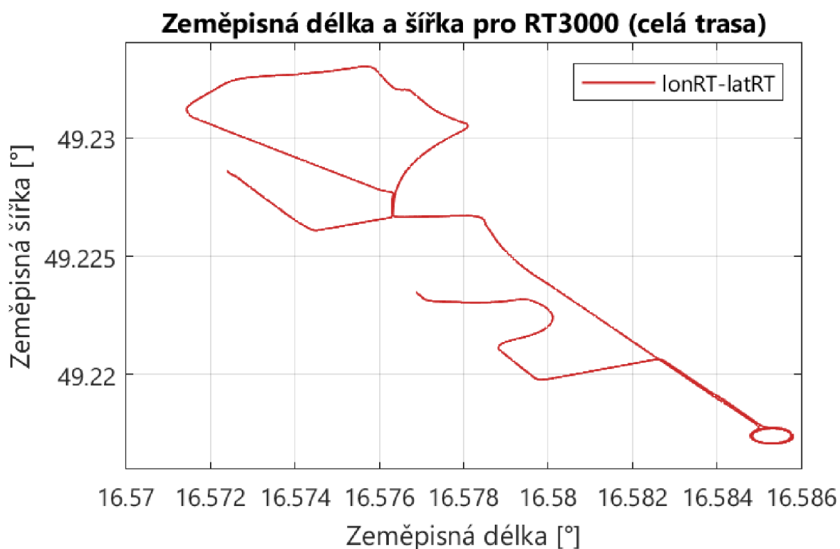
Obr. 38 Graf zeměpisné délky a šířky pro RT3000 (celá trasa)
