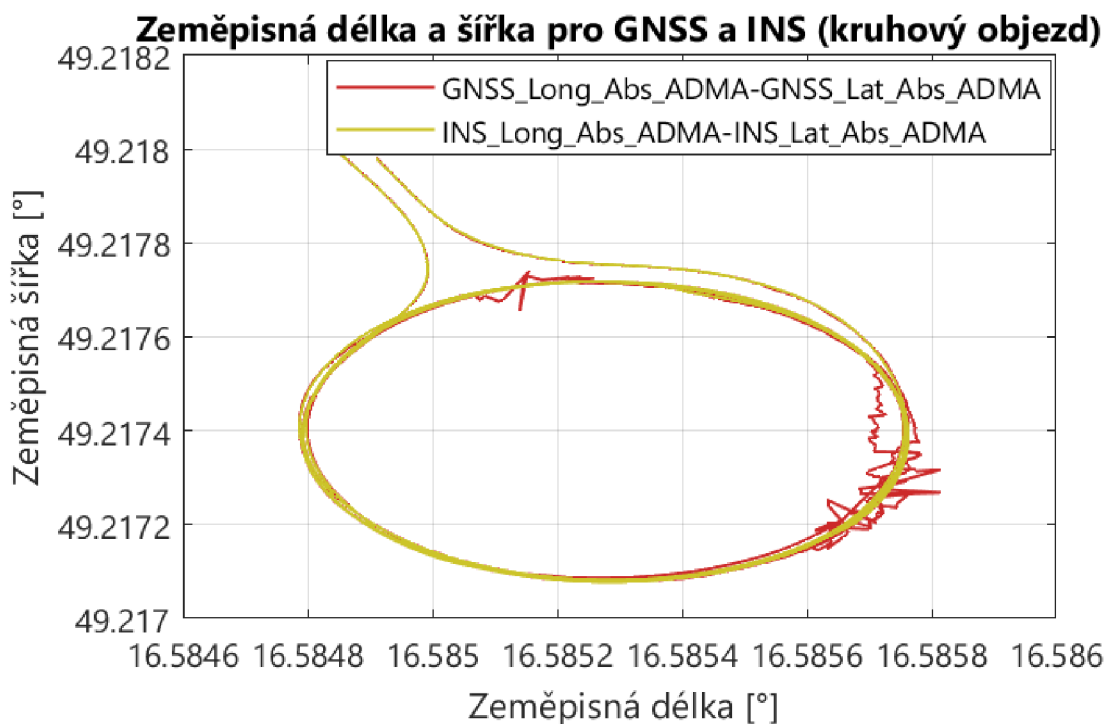
Obr. 44 Graf zeměpisné délky a šířky pro GNSS a INS (kruhový objezd)
