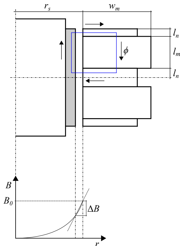
Obr. 3.6: Magnetický tok v řezu elektrodynamického ložiska
