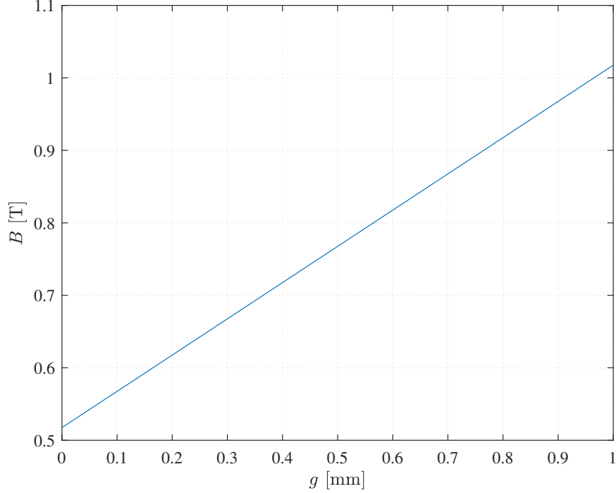
Obr. 6.2: Velikost magnetické indukce B ve vzduchové mezeře od vnějšího okraje vycentrovaného rotoru po stator
