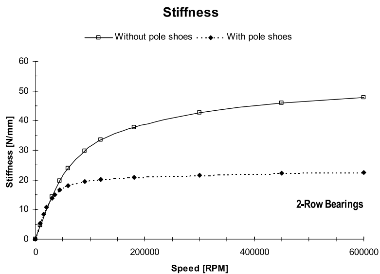
Obr. 8.8: Tuhost v závislosti na tom, zda byly použity pólové nástavce [2]
