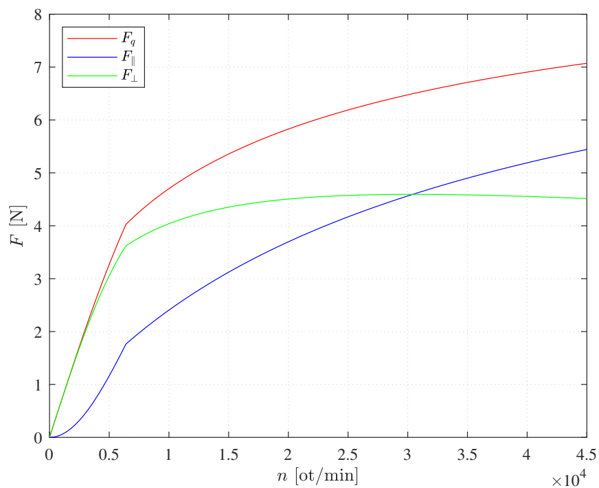
Obr. 6.4: Síla rovnoběžná F_{\parallel} a kolmá F_{\perp} na směr vychýlení a výsledná síla F_q
