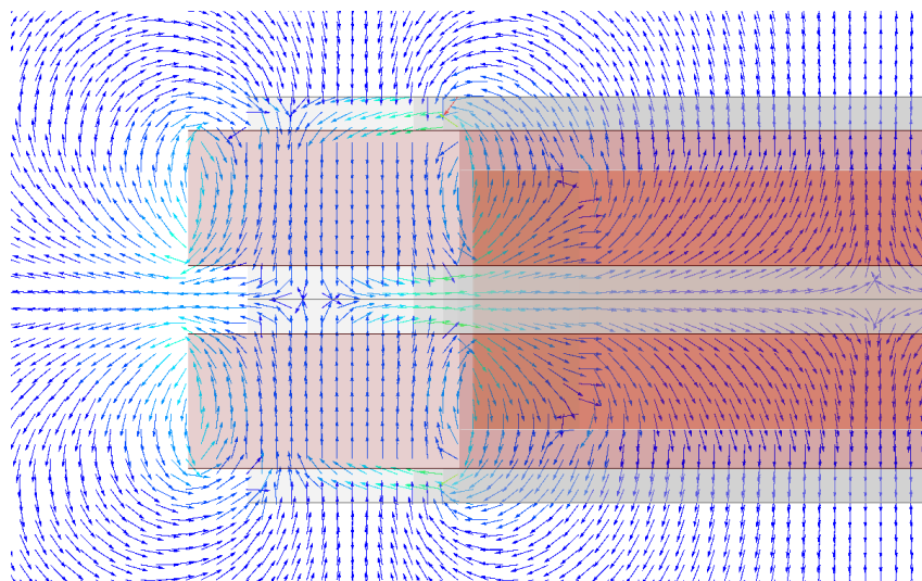
Obr. 6.14: Rozložení vektorů magnetické indukce v řezu ložiska
