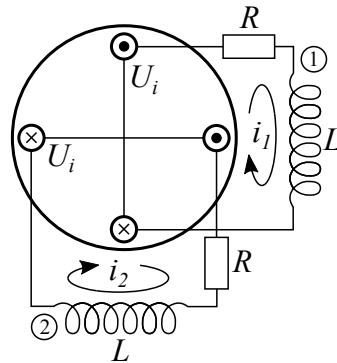
Obr. 3.2: Znázornění elektrického obvodu ve vodivém materiálu rotoru, překresleno z [20]
