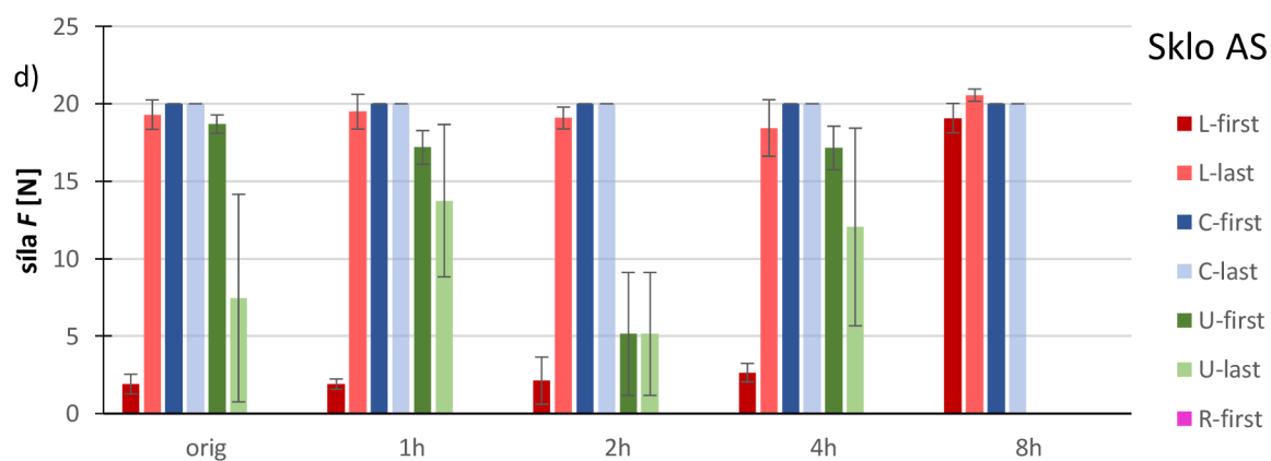
Obr. 25: Grafy pro sklo AS při indentaci 20 N. a) uvolněná energie b) počet událostí c) čas vzniku AE d) působící síla při vzniku AE.
