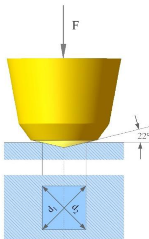
Obr. 6: Indentor pro indentační metodu podle Vickerse
