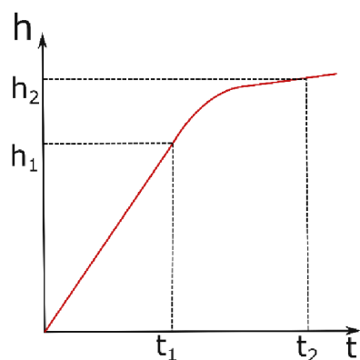
Obr. 12: Ukázka creepu.
