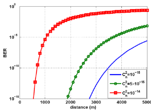
Obr. 1.4: BER podle vzdálenosti a C_n^2 [14]
