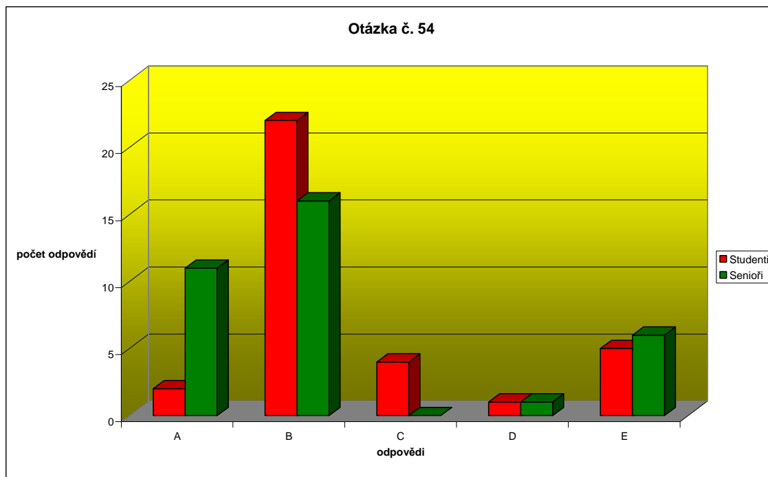
Graf 28: Vnímáte skutečnost, že vánoční a velikonoční zboží se objevuje na trhu s několikaměsíčním předstihem jako tradice?
