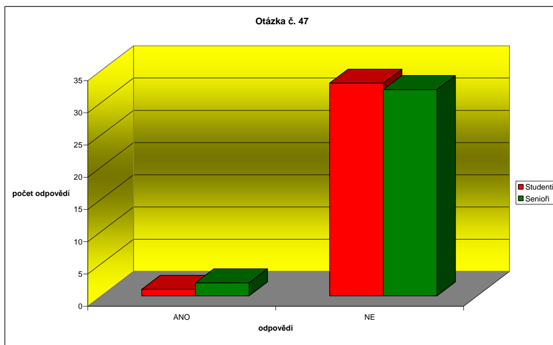
Graf 23: Chodíte o svátku sv. Štěpána koledovat?
