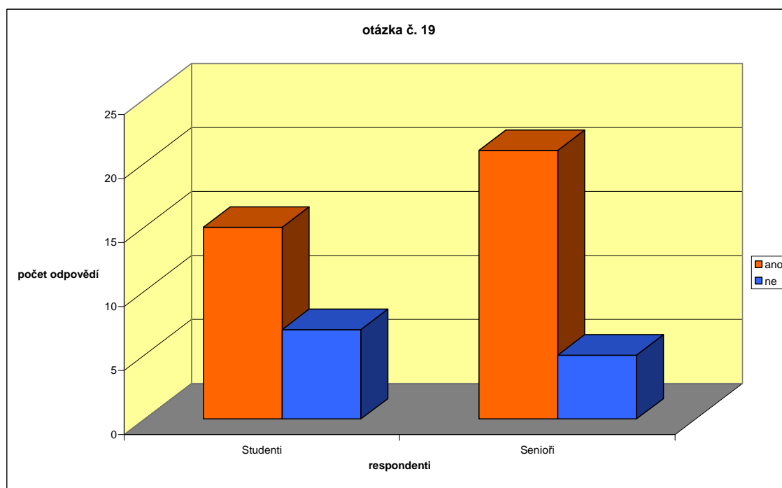
Graf 9: Jste-li žena, barvíte o Velikonocích kraslice?
