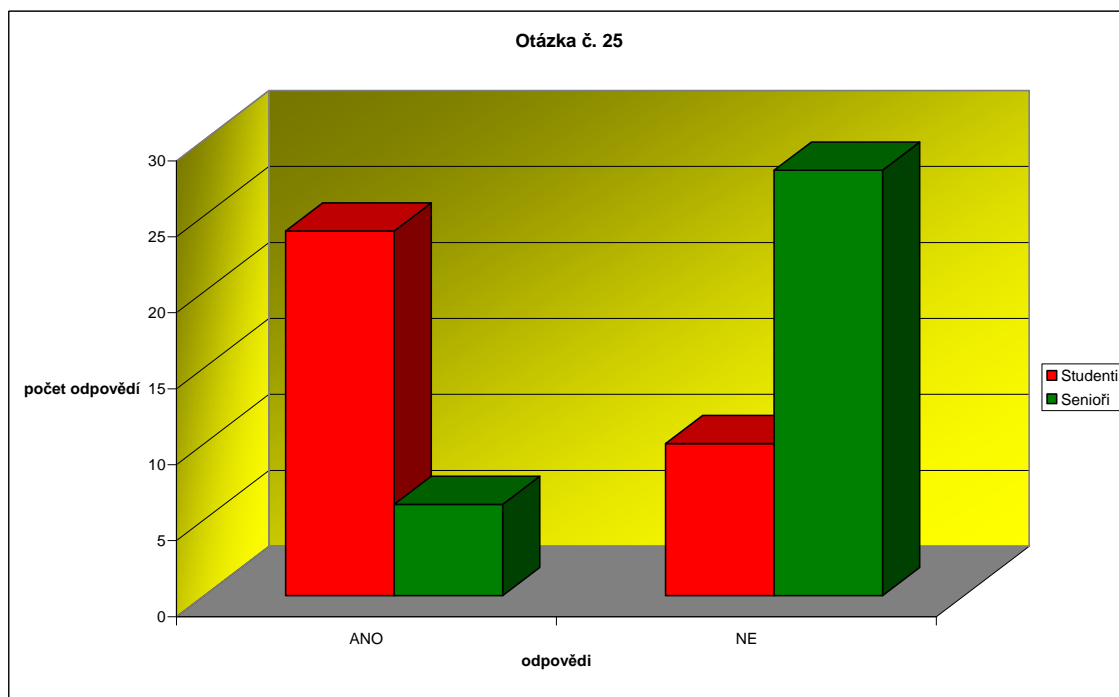
Graf 11: Účastníte se o Filipojakubské noci pálení čarodějnic?
