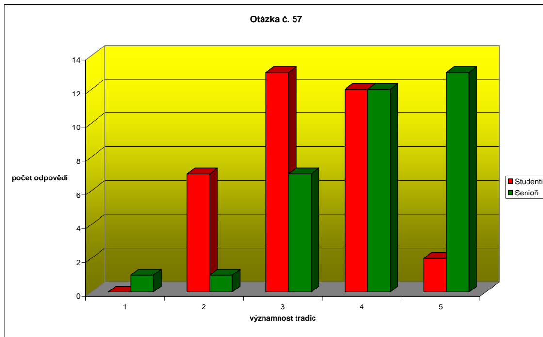
Graf 31: Domníváte se, že dodržování tradic má pro člověka význam:
