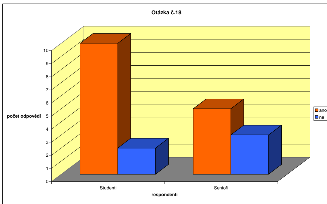
Graf 8: Jste-li muž, chodíte na Velikonoce koledovat?
