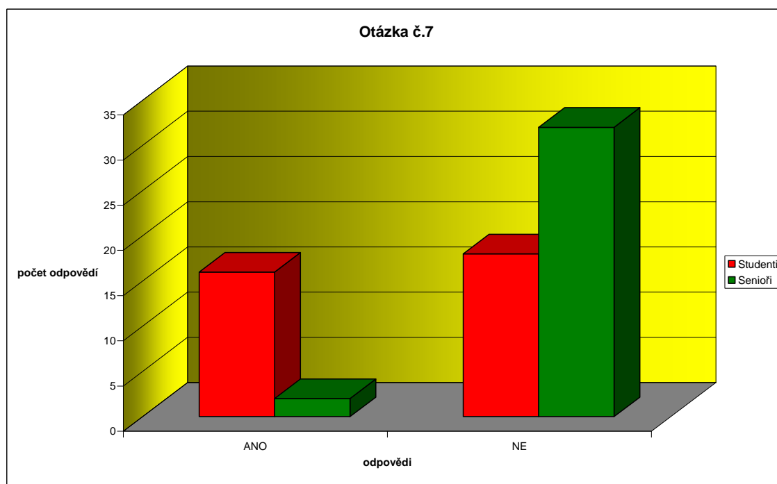
Graf 1: Dáváte si na Nový rok předsevzetí
