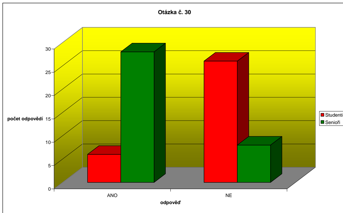
Graf 16: Víte, proč se na svátek Všech věrných zemřelých rozsvěcejí svíčky?
