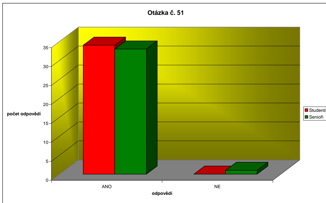
Graf 26: Myslíte si, že v dnešní době má smysl dodržovat tradice?
