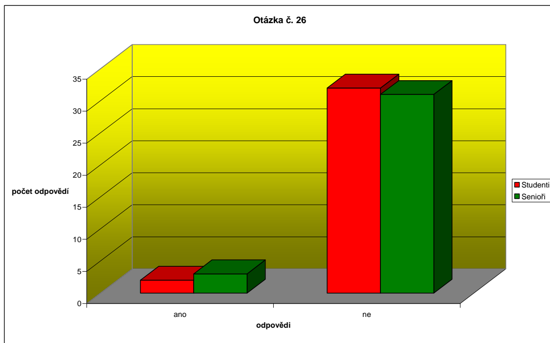
Graf 12 Účastníte se stavění májky?
