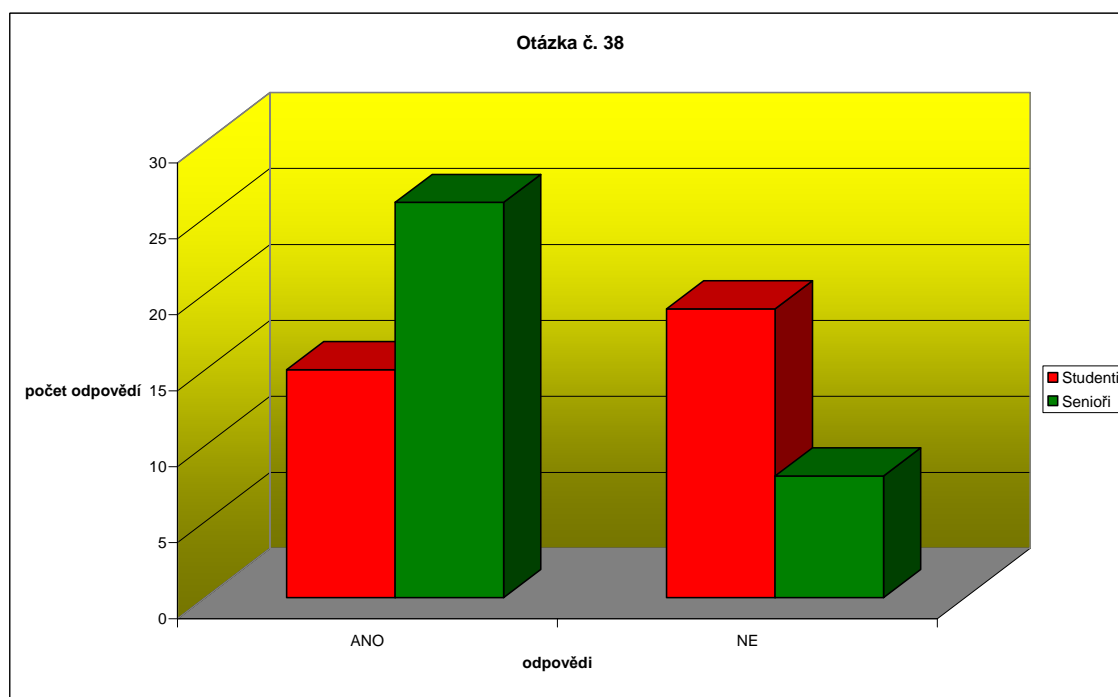
Graf 19: Slavíte svátek sv. Mikuláše?
