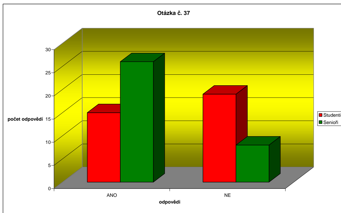
Graf 18: Dáváte si do vázy barborky?
