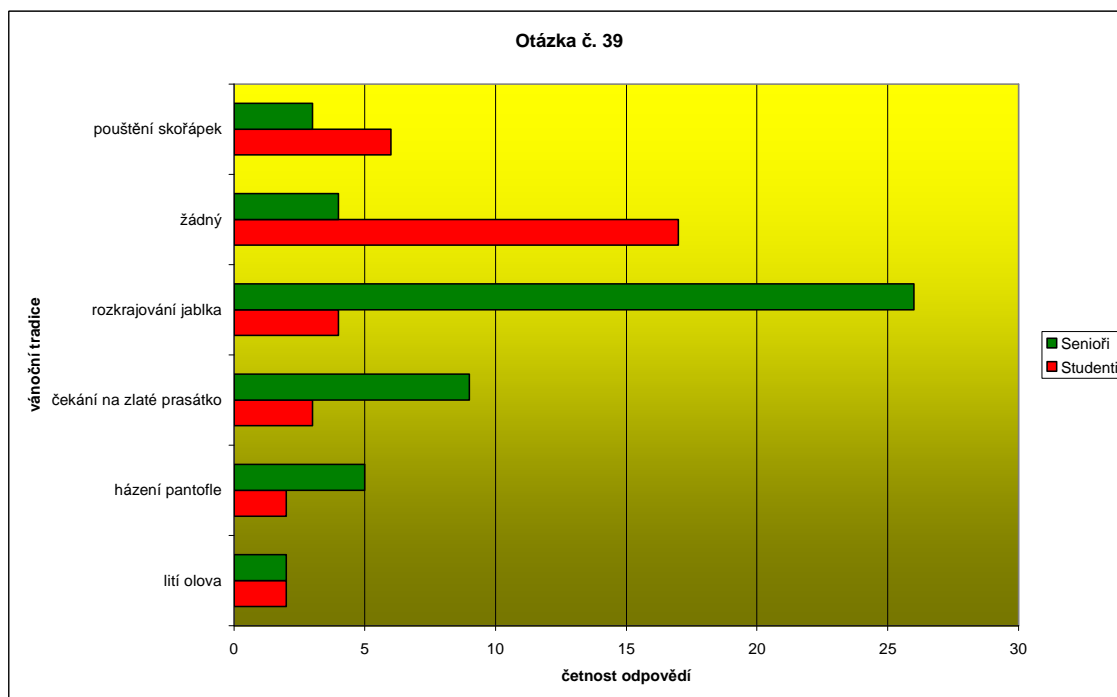
Graf 20: Dodržujete na štědrý den vždy některý ze zvyků?
