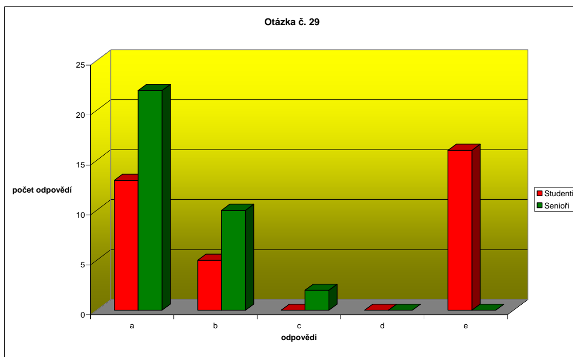
Graf 15: Jak trávíte svátek Všech věrných zemřelých?
