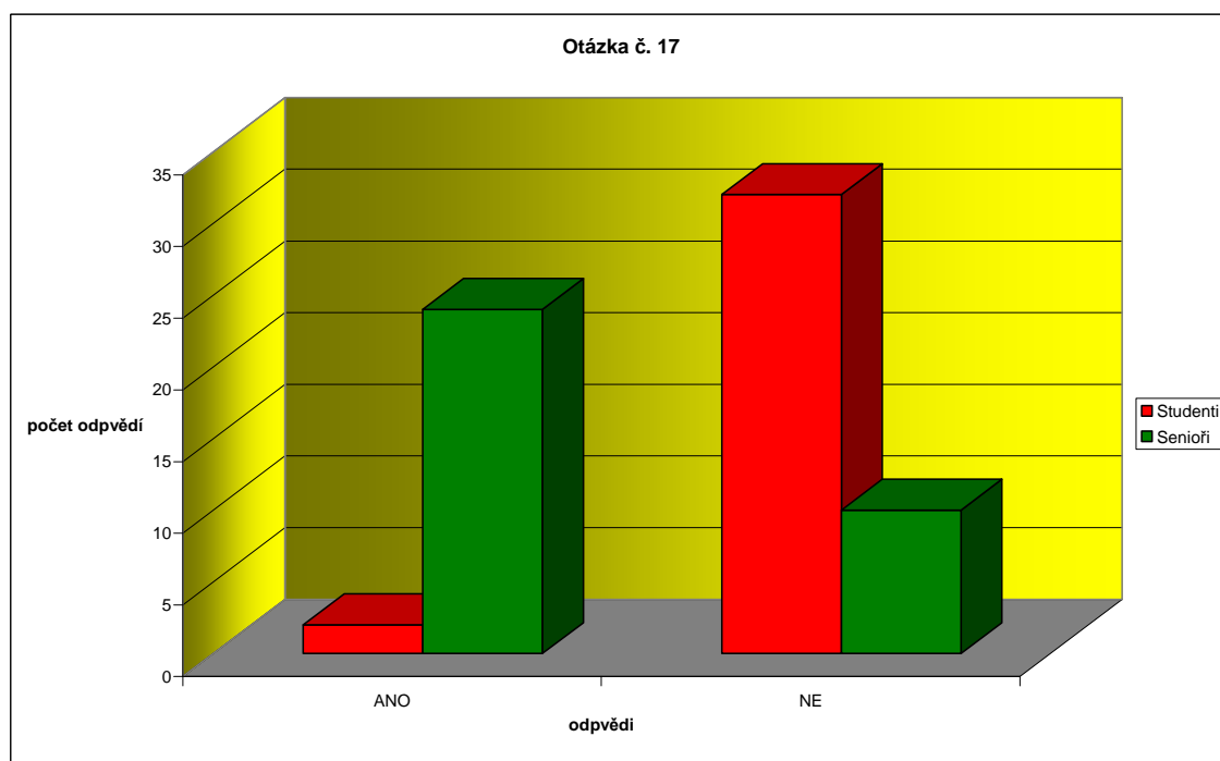
Graf 7: Jíte na Zelený čtvrtek o Velikonocích pouze zelenou stravu?
