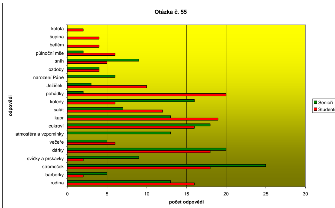
Graf 29: Napište 5 slov, která se Vám vybaví při slově Vánoce
