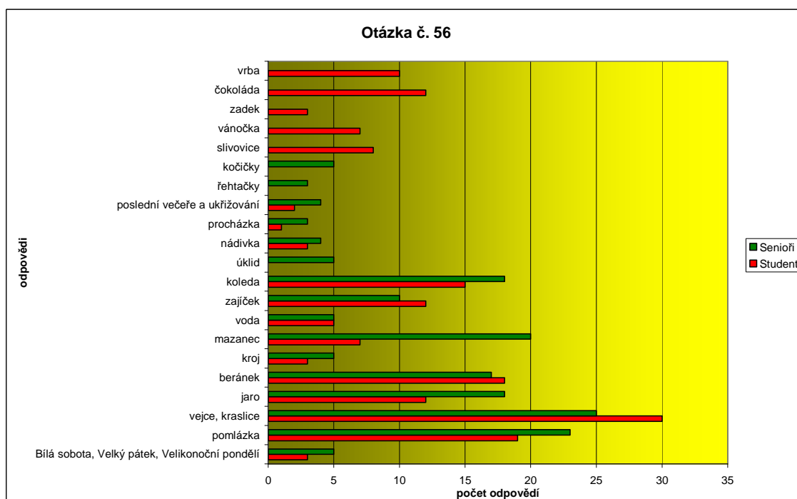
Graf 30: Napište 5 slov, která se Vám vybaví při slově Velikonoce:
