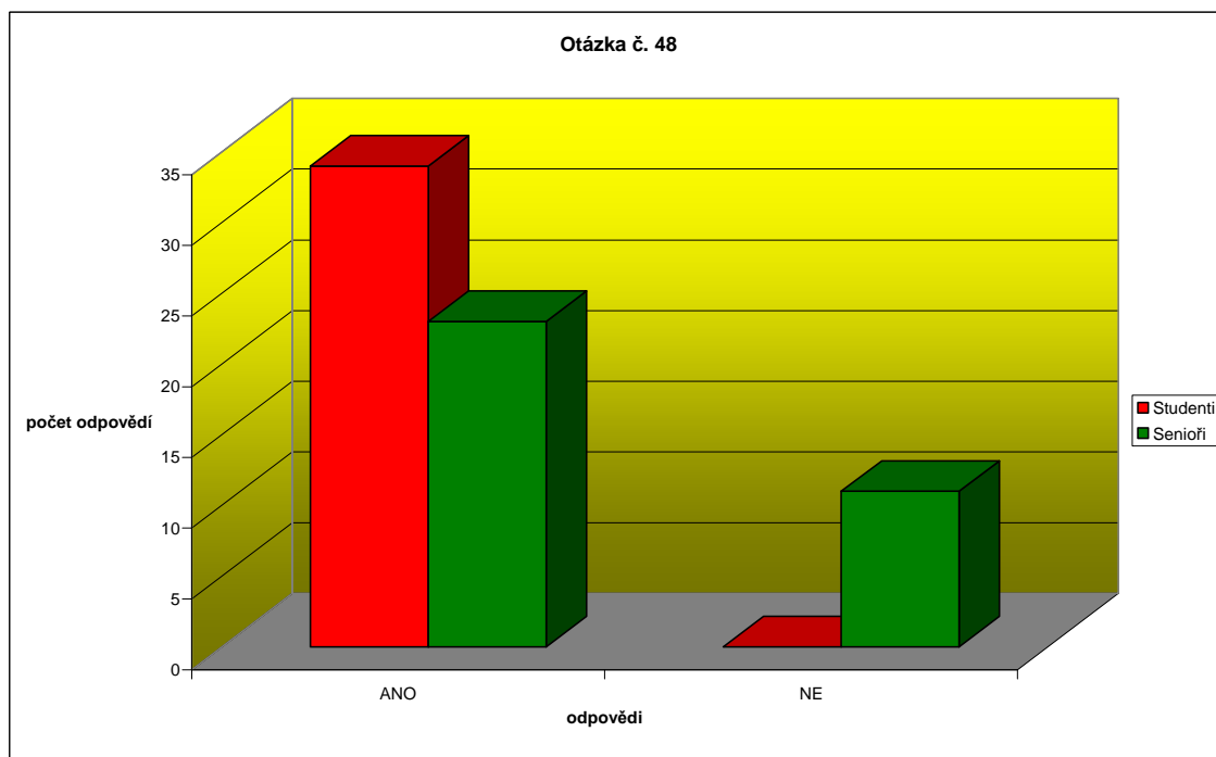
Graf 24: Slavíte Silvestra?
