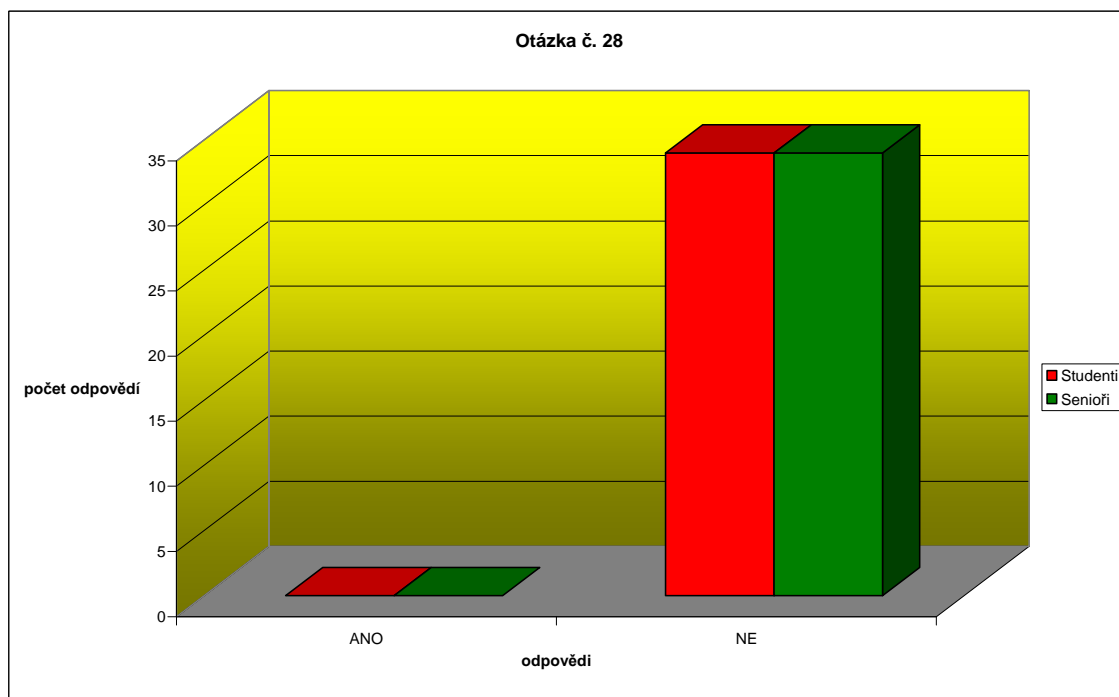
Graf 14: Účastníte se zapalování Svatojánských ohňů?
