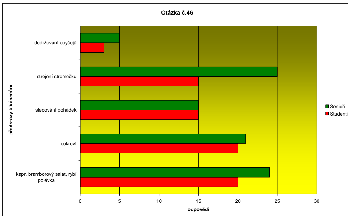
Graf 22: O Štědrém dni podle Vás nesmí chybět:
