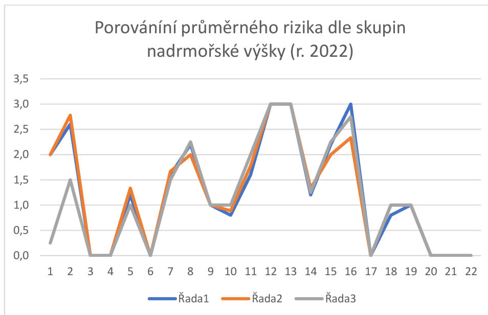
Graf 2: Porovnání průměrného rizika dle skupin nadmořské výšky (r. 2022) (zpracování autora)
