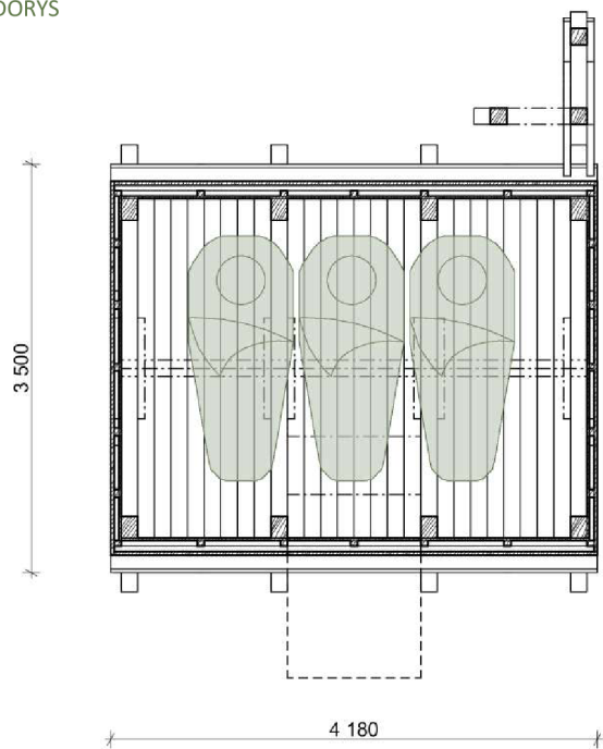
PŮDORYS
