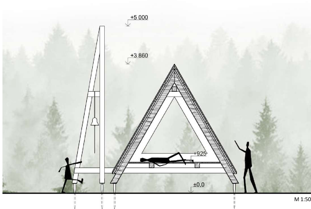
PŘÍČNÝ ŘEZ
