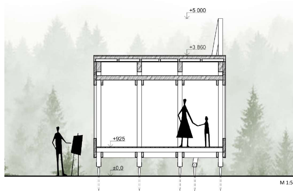
PODÉLNÝ ŘEZ
