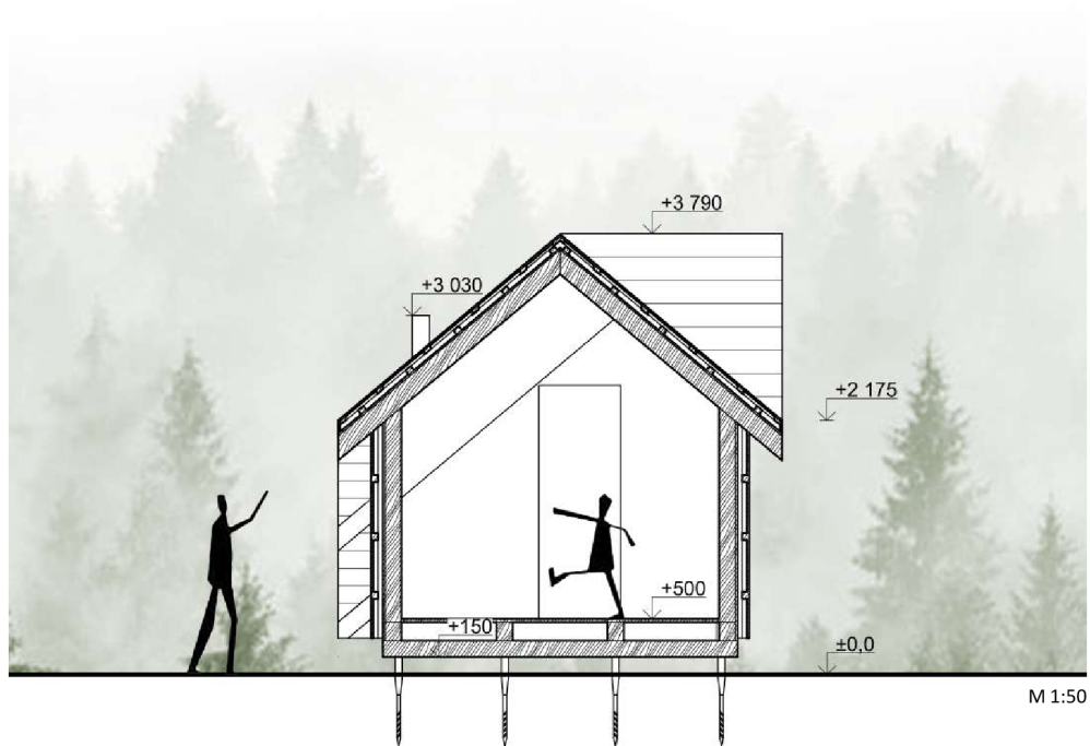
PŘÍČNÝ ŘEZ
