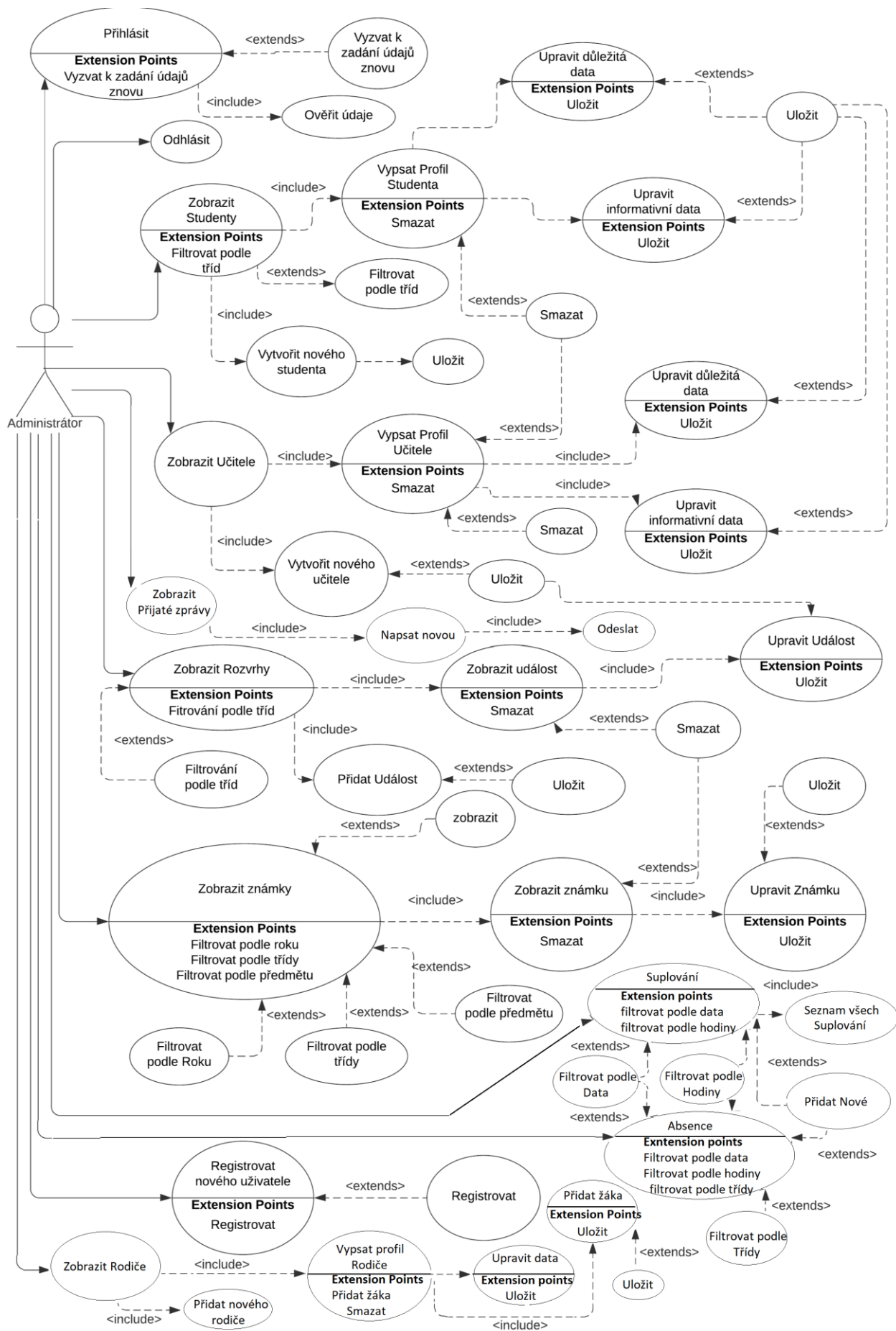
Obrázek 5 - Use Case Diagram z pohledu Administrátora
