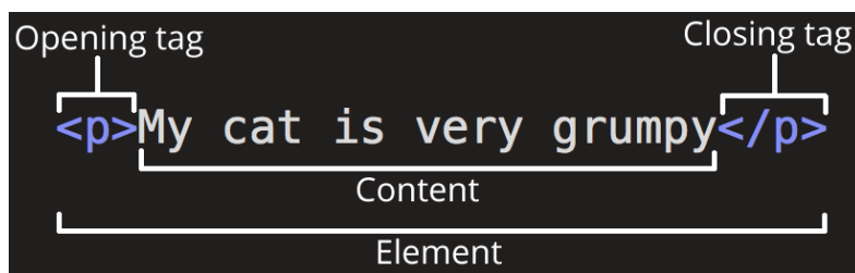
Obrázek 2 - Příklad HTML [2]
