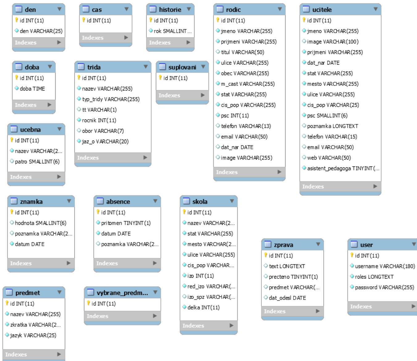
Obrázek 11 - Seznam Atributů v Entitách v Databázi
