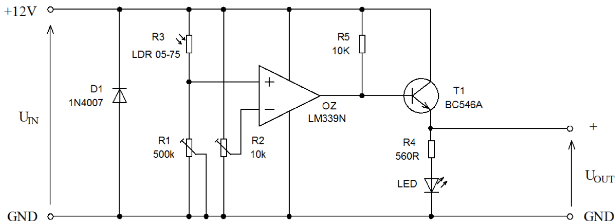
Obr. 8-1 Schéma vyrobeného optoelektronického snímače
