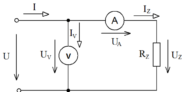
Obr. 2-3 Nepřímé měření výkonu stejnosměrného proudu v zapojení VA
