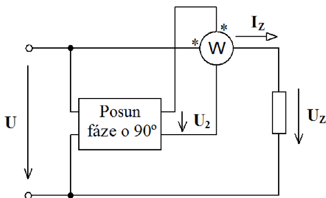
Obr. 2-8 Zapojení wattmetru pro přímé měření jalového výkonu
