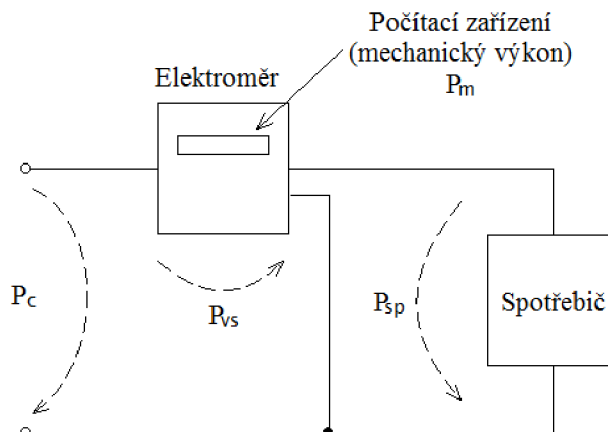
Obr. 3-1 Naznačení vlastní spotřeby elektroměru
