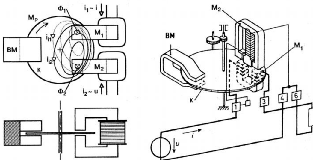
Obr. 3-2 Princip indukčního měřicího ústrojí a jeho náčrtek [1]
