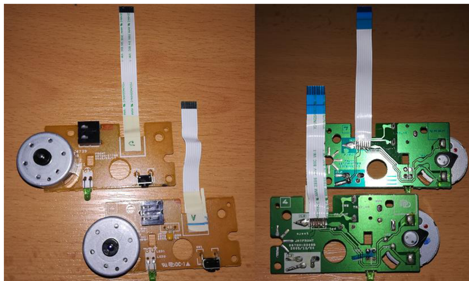
Obr. 10 Motorčky zásuvky na disk z mechanik LG, nahoře ze čtecí mechaniky, dole z vypalovací.
