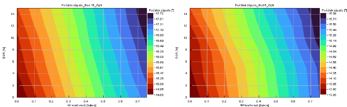
Obr. 128: EGR vs. vodní vstřikování – počátek zápalu
