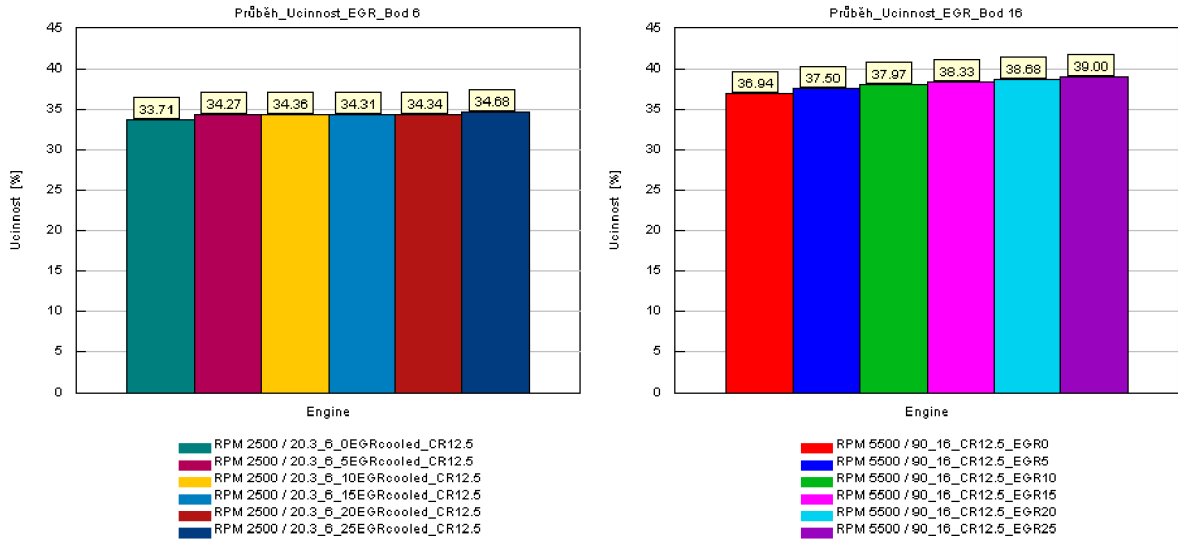
Obr. 65: Závislost množství recirkulovaných spalin na účinnosti
