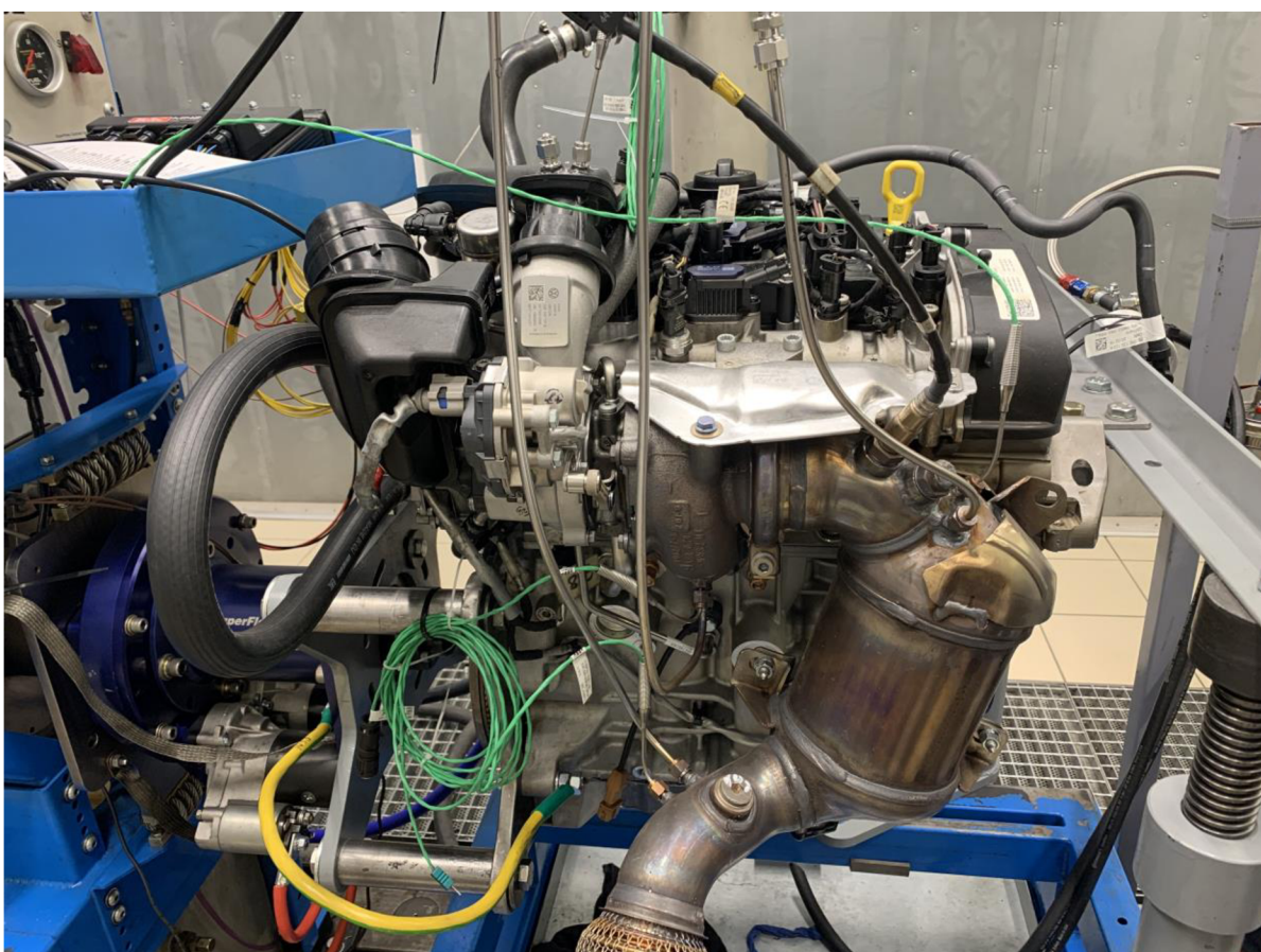
Obr. 31: Testovaný motor na měřicí stolici osazený měřicími senzory
