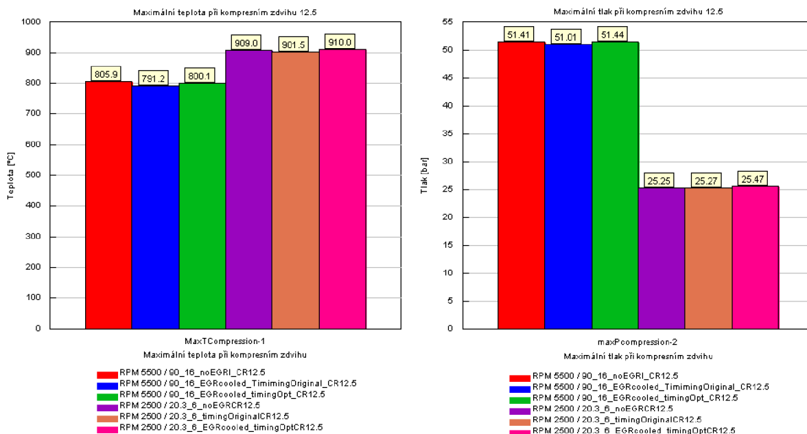
Obr. 82: Maximální teplota a tlak při kompresním zdvihu
