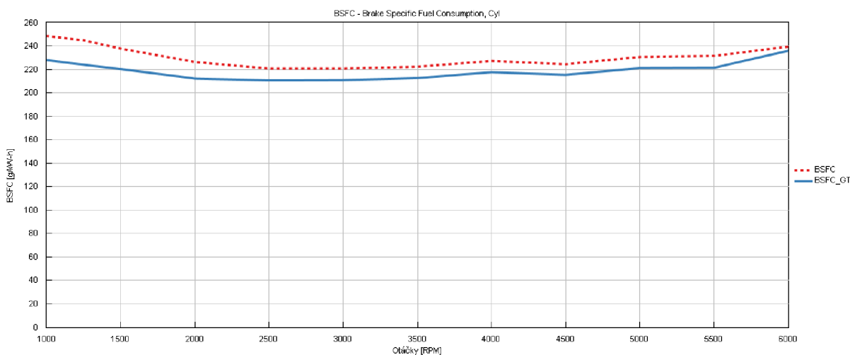
Obr. 54: Porovnání měrné spotřeby paliva u experimentu a modelu
