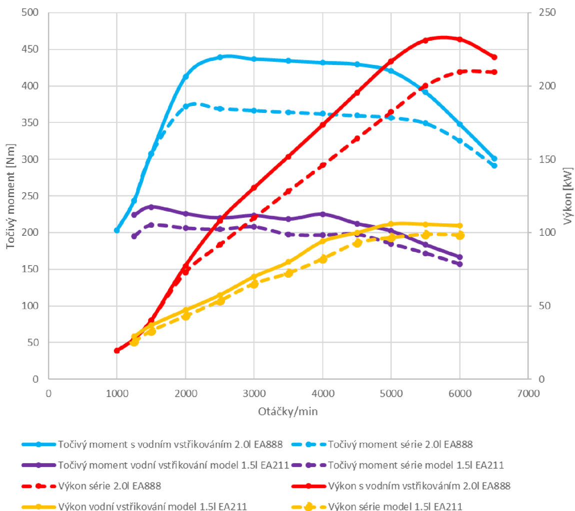
Obr. 138: Změřená data experimentálního vozidla s motorem 2.0 l EA888 a modelu 1.5 l EA211 evo
