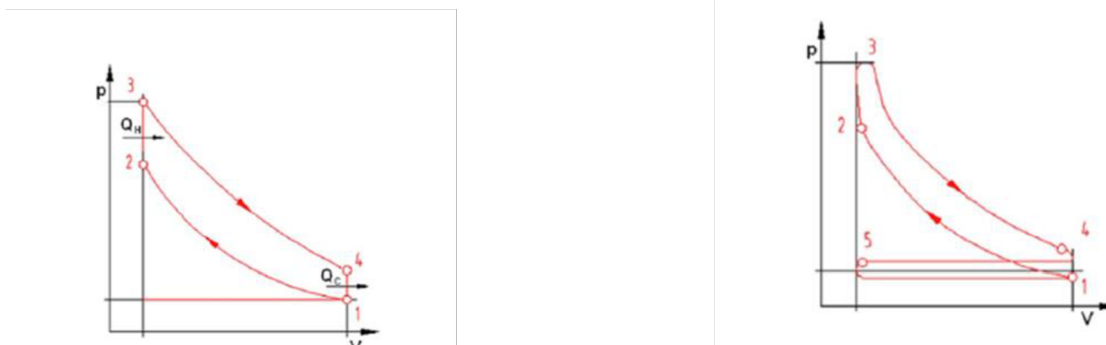
Obr. 21: Čerpací ztráty [15]
