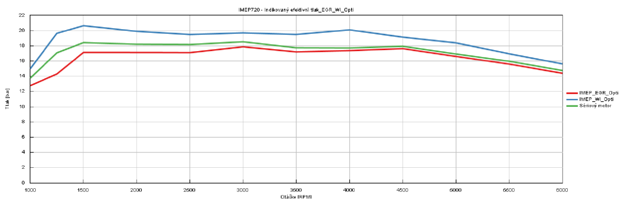
Obr. 121: Porovnání středního efektivního tlaku
