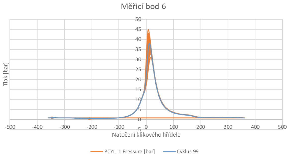
Obr. 37: Analýza indikačního tlaku u měřicího bodu 6
