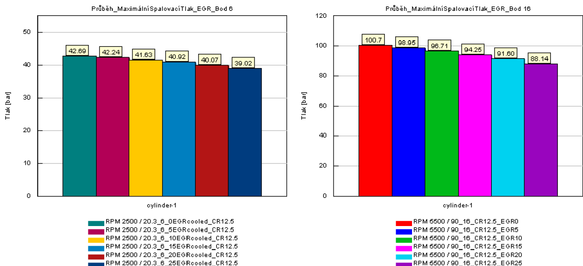
Obr. 68: Závislost množství recirkulovaných spalín na maximálním spalovacím tlaku
