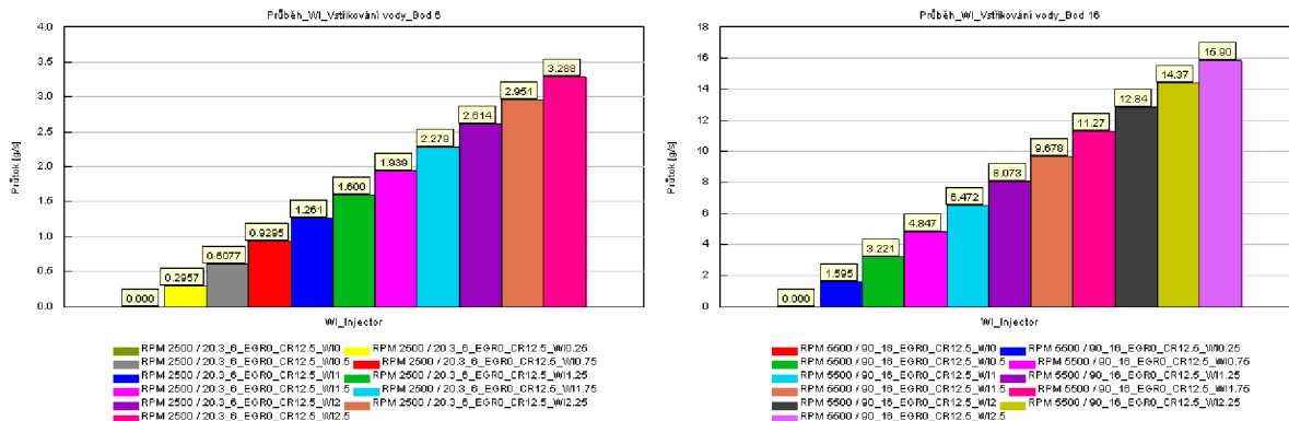
Obr. 101: Množství vstřikování vody
