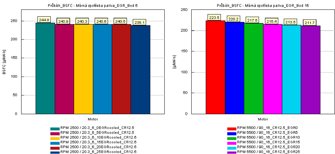
Obr. 64: Závislost množství recirkulovaných spalín na měrné spotřebě paliva
