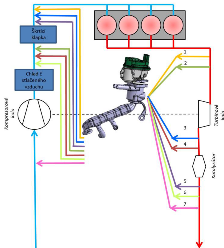
Obr. 24: Architektura pro přepřítňované motory
