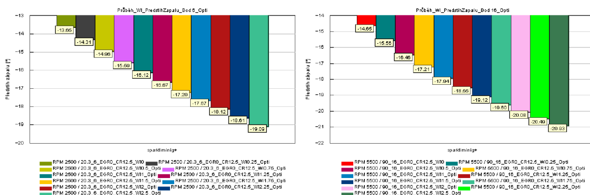
Obr. 110: Závislost předstihu zážehu na množství vstřikované vody
