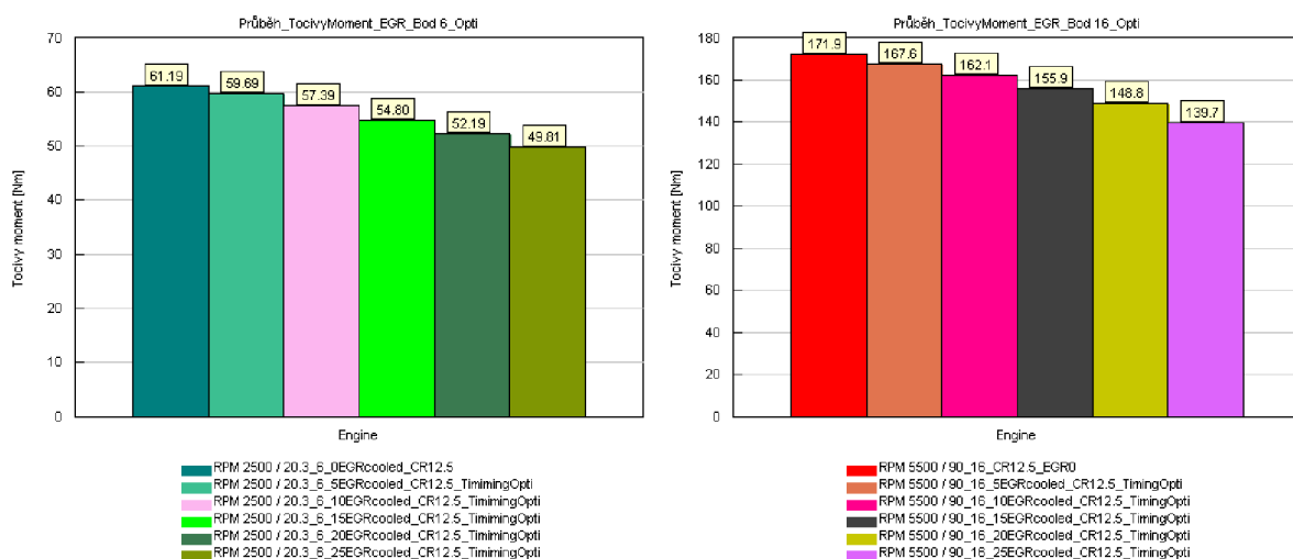
Obr. 72: Závislost množství recirkulovaných spalín na točivém momentu – optimalizovaný předstih zážehu
