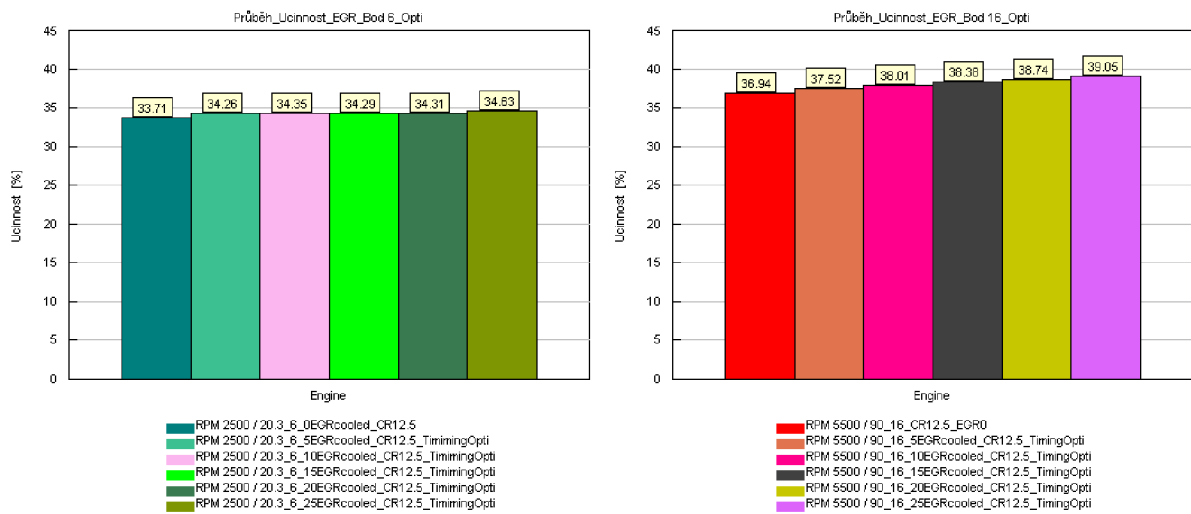
Obr. 74: Závislost množství recirkulovaných spalin na účinnosti motoru – optimalizovaný předstih zážehu
