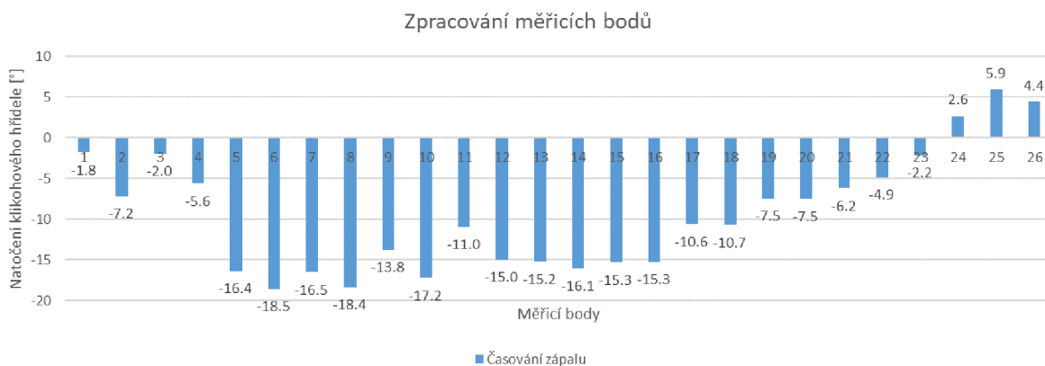
Obr. 42: Časování zápalu
