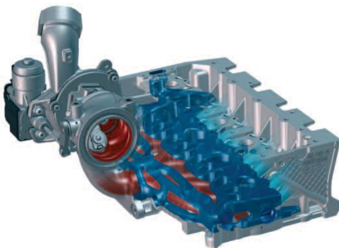
Obr. 29: Výfukové svody motoru EA 211 evo chlazené chladičím kapalinou [32]
