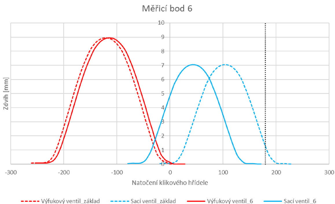
Obr. 43: Průběh zdvihu ventilů u měřicího bodu 6
