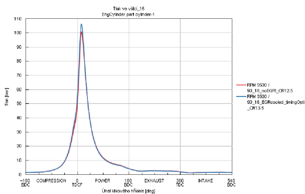
Obr. 90: Průběh tlaků ve válci
