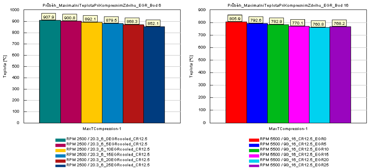
Obr. 66: Závislost množství recirkulovaných spalin na maximální kompresní teplotě
