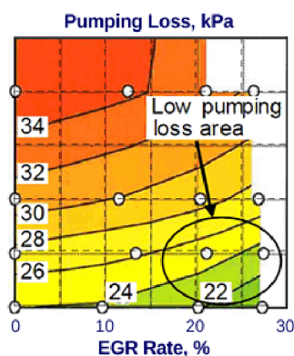
Obr. 22: Vliv EGR na tlakové (čerpací) ztráty [16]
