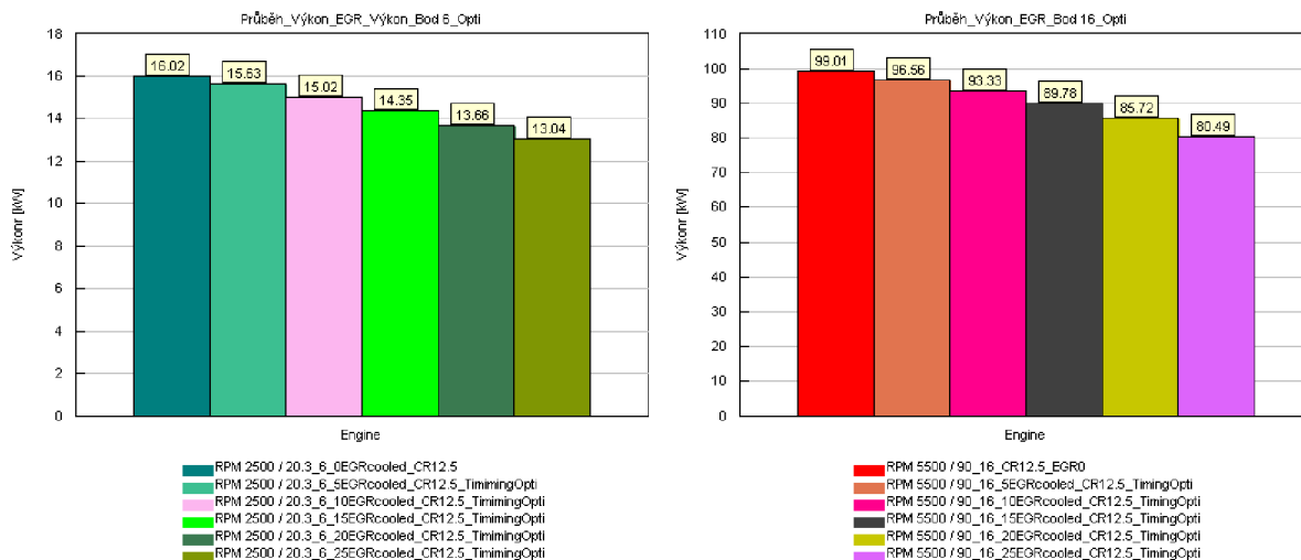
Obr. 71: Závislost množství recirkulovaných spalín na výkonu – optimalizovaný předstih zážehu
