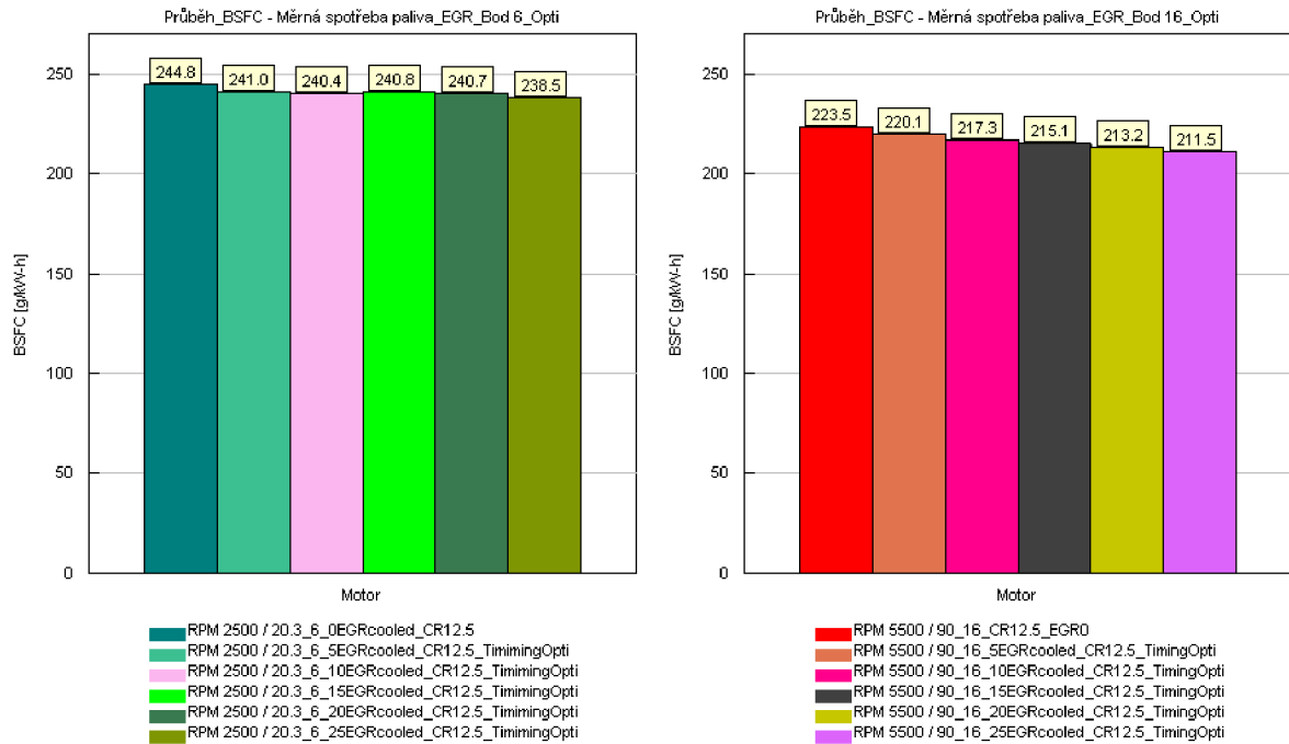
Obr. 73: Závislost množství recirkulovaných spalin na měrné spotřebě paliva – optimalizovaný předstih zážehu
