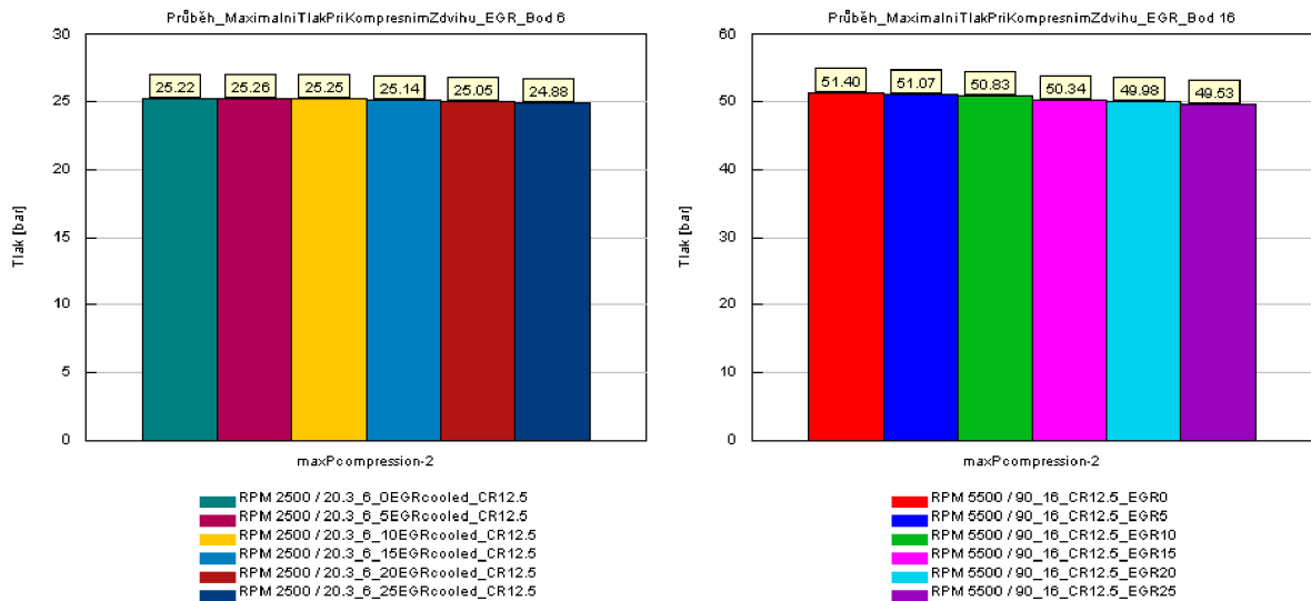
Obr. 67: Závislost množství recirkulovaných spalín na maximálním kompresním tlaku
