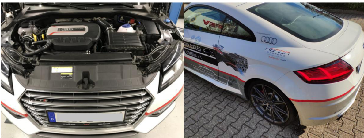
Obr. 137: Experimentální vozidlo s vodním vstřikováním
