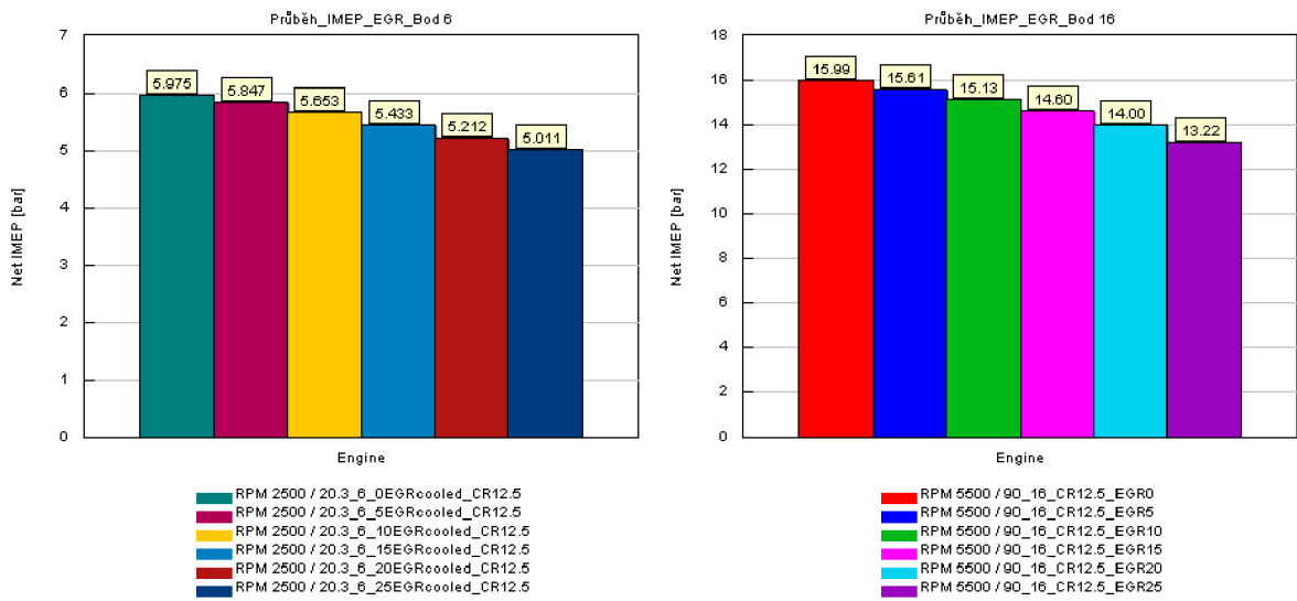
Obr. 61: Závislost množství recirkulovaných spalín na středním efektivním tlaku
