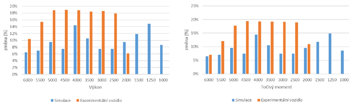
Obr. 139: Relativní srovnání simulace a experimentu (Výkon, Točivý moment)
