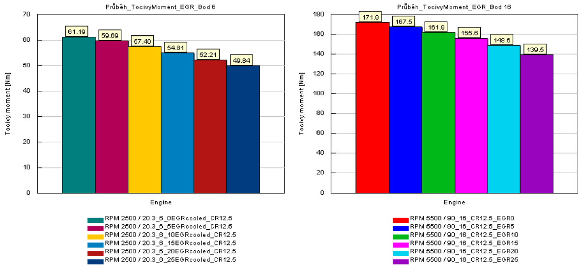
Obr. 63: Závislost množství recirkulovaných spalín na točivém momentu
