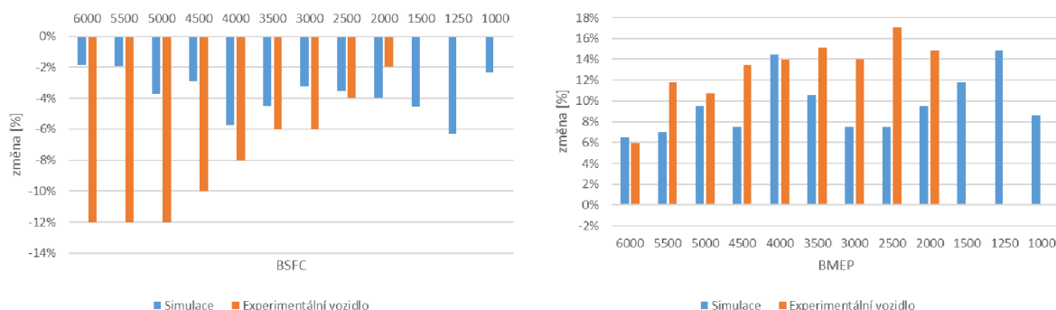
Obr. 140: Relativní srovnání simulace a experimentu (BSFC, BMEP)
