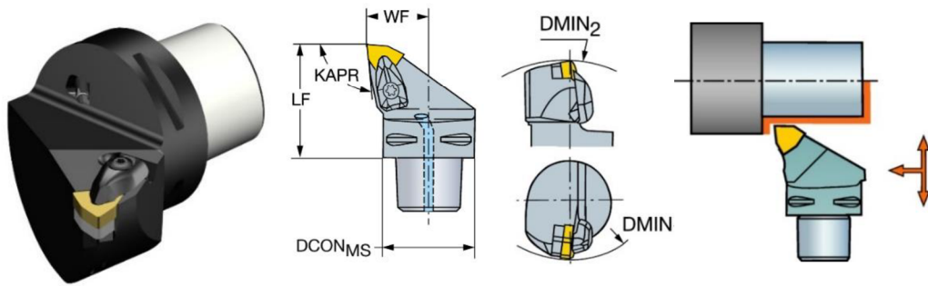
Obr. 12 Nástroj C6-DWLN-45065-08 [15].
