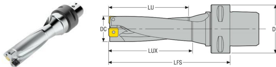
Obr. 31 Vrták SD523-40-120-C6 [16].
