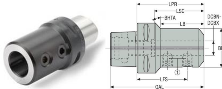
Obr. 46 Upínač C6-391.27-40085 [16].
