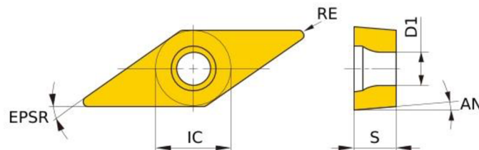
Obr. 23 Břitová destička VBGT110302L-F [17].
