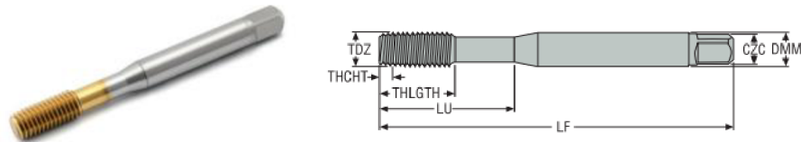
Obr. 38 Tvářecí závitník MF-M10X1.50ISO6HX-XE-V053 [16].
