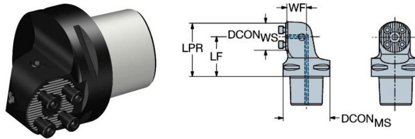
Obr. 17 Nástroj C6-570-32-RF [15].
