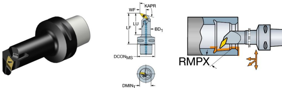
Obr. 22 Nástroj C6-SVQBR-22120-16HP [15].
