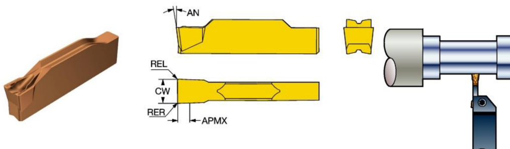
Obr. 19 Destička N123G1-0300-0003-TF 1125 [15].
