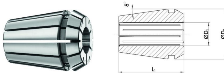
Obr. 36 Kleština CC ER 25 Ø14-15 [13].
