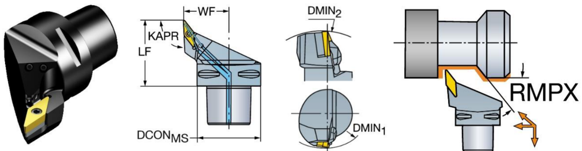
Obr. 20 Nástroj C6-SVJBR-45065-16HP [15].
