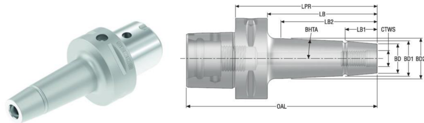
Obr. 26 Upínač C6-391.5820-10075 [16].
