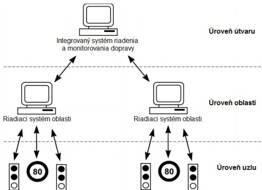
Obr. 2.2: Trojvrstvová architektúra telematického systému. [2]
