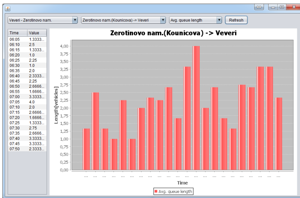
Obr. 3.3: Okno s detailnými štatistikami.
