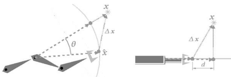
Obrázek 5: Cyclinc Coordinate Descent metoda pro a) rotační kloub b) translační kloub[16]
