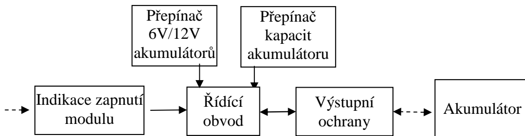
Obr. 4.13: Blokové schéma modulu nabíjecího gelové olověné baterie
