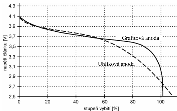
Obr. 2.10: Vybíjecí charakteristika Li-Ion článku; převzato z [11]
