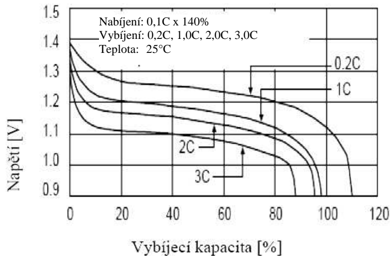
Obr. 2.4: Vybíjecí charakteristika NiMH článku; převzato z [4]
