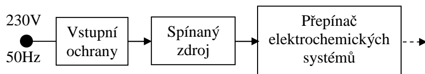
Obr. 4.2: Blokové schéma modulu zdroje
