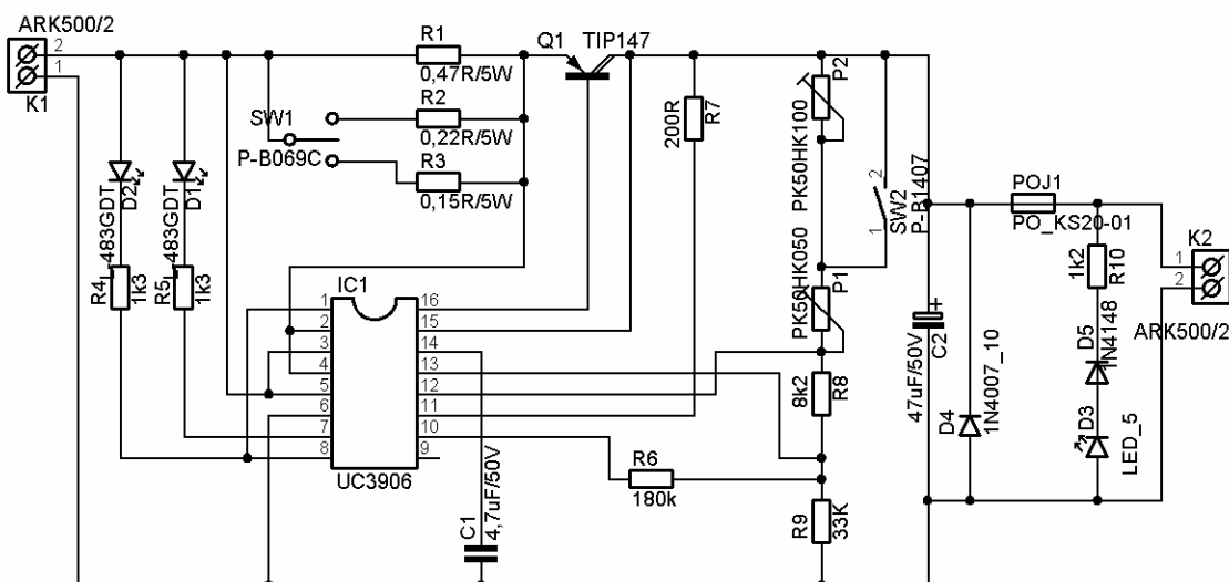
Obr. 4.15: Schéma modulu, který nabíjí gelové olověné baterie
