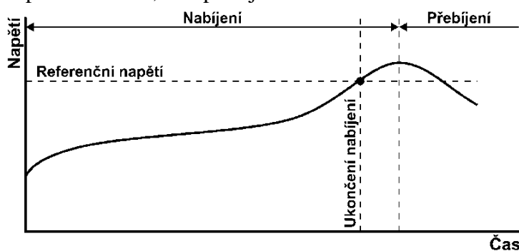
Obr. 3.1: Ukončení nabíjení při dosažení stanoveného napětí; převzato z [9]
