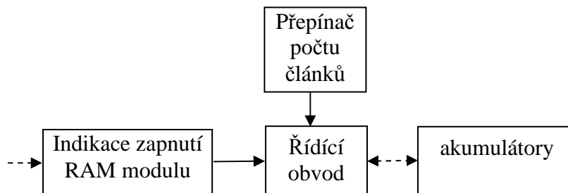
Obr. 4.10: Blokové schéma modulu nabíječického RAM akumulátory
