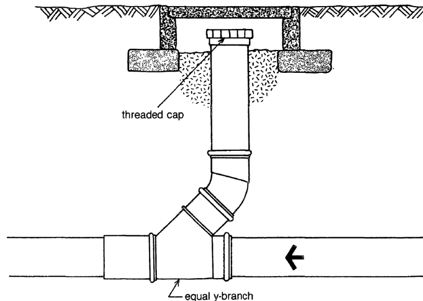
Obr.14-Šachtička (čistící kus) [12]
