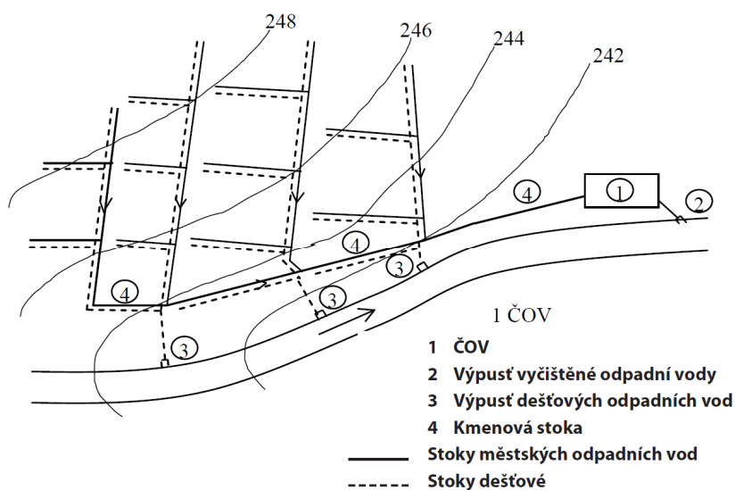
Obr.2-Oddílná kanalizace [7]
