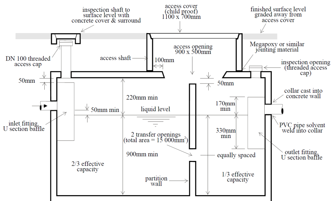
Obr.13-Schéma dvoukomorového septiku [16]
