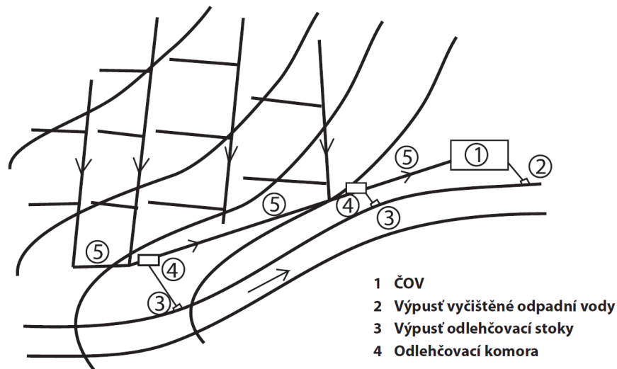
Obr.1-Jednotná kanalizace [7]
