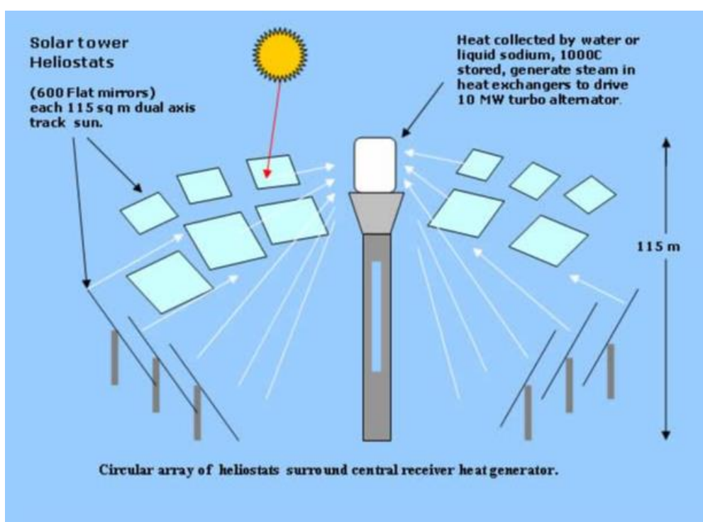
Obr. 11 Princip koncentrování sluneční paprsků (11)
