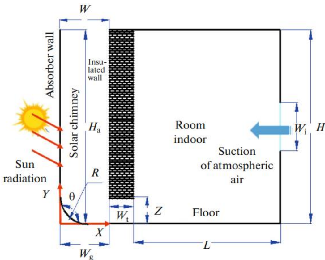
Obr. 8 Větrání pomocí Trombeho stěny (11)
