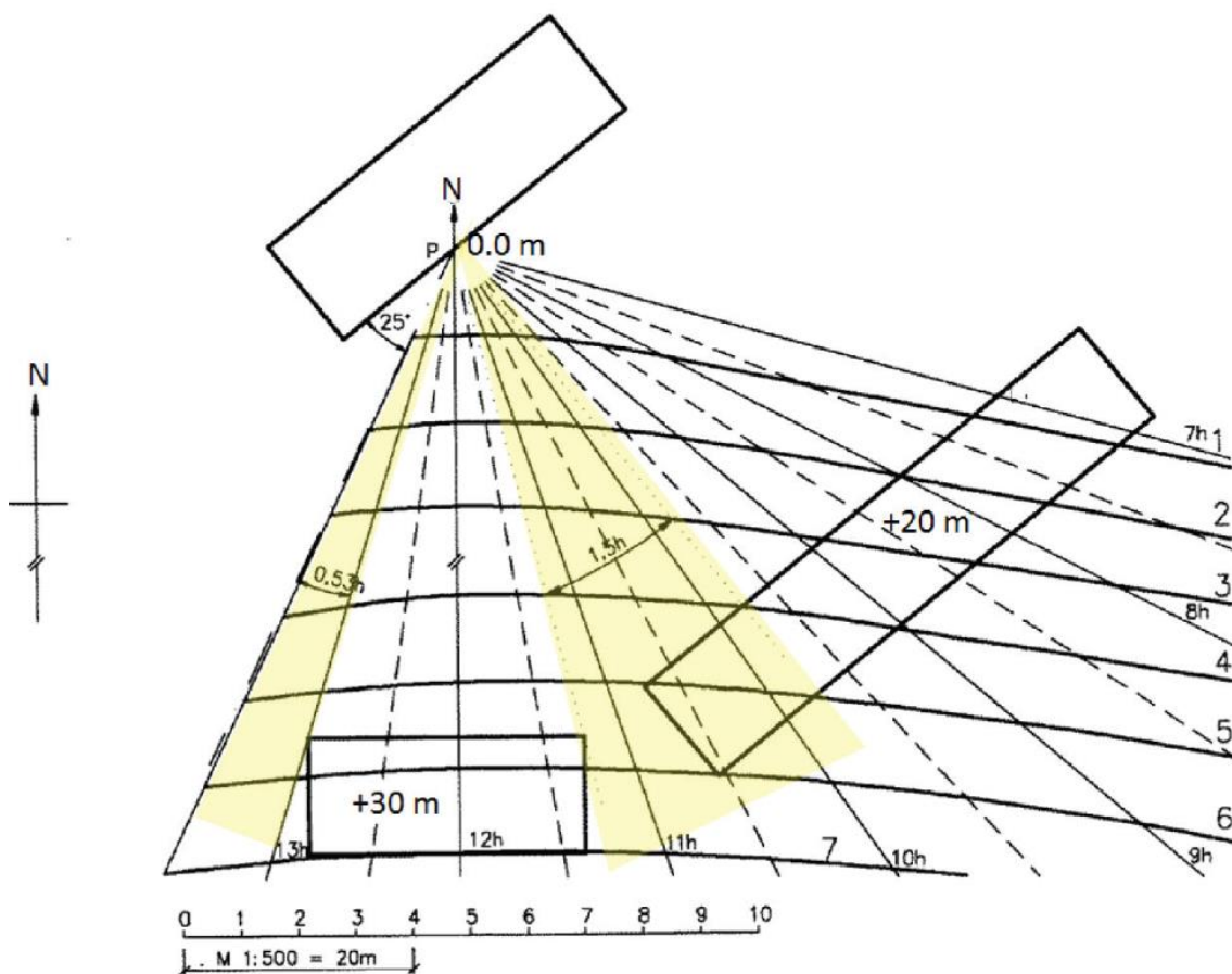
Obr. 4 Model osvětlení budu P se zastíněním budovami 20m a 30m vysokými (6)
