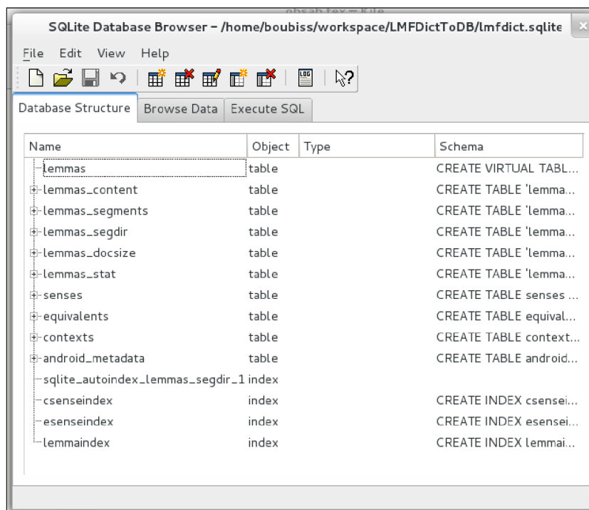
Obr. 5.1: SQLite3 browser
