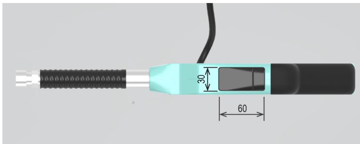
obr. 6-19 Rozměry displeje
