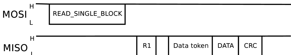
Obr. 3.2: Čtení dat z karty (jednoblokové)
