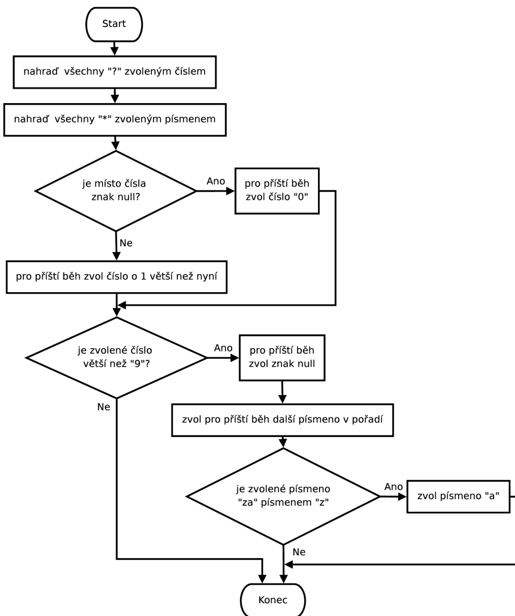
Obr. 7.4: Funkce wildtranslate
