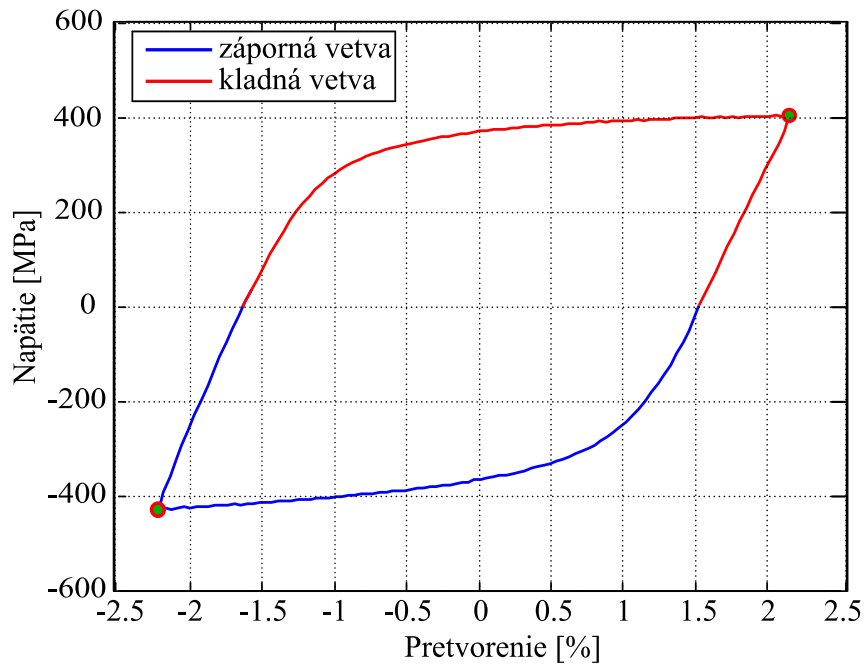
Obrázok 5.16: Rozdelenie hysteréznej slučky na kladnú a zápornú vetvu.
