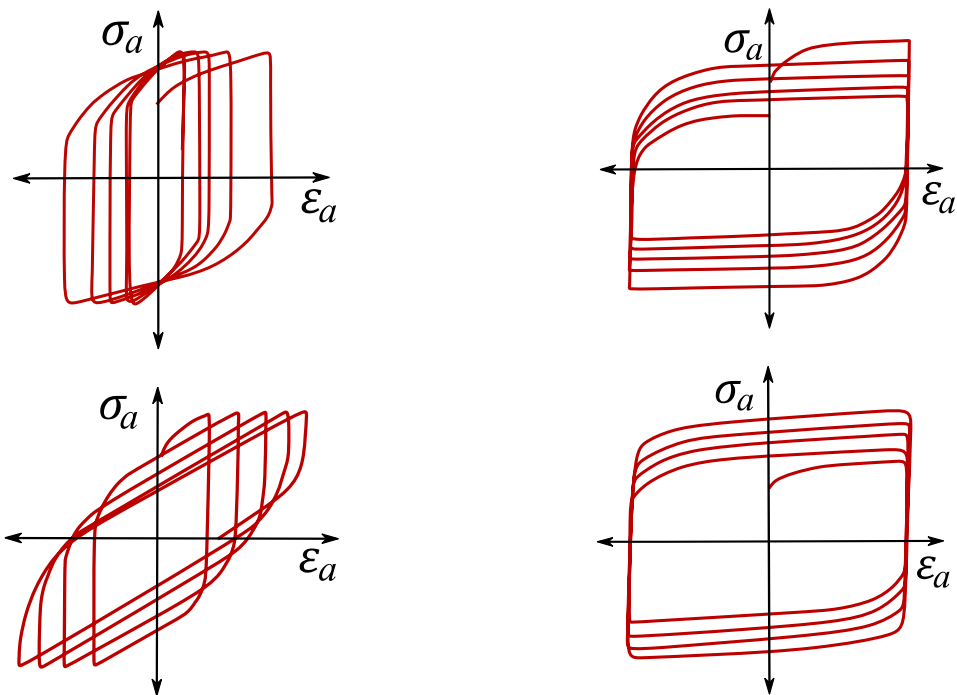
Obrázok 5.14: Tvar hysteréznej slučky pri zaťažovaní s konštantnou amplitúdou napätia pre materiál, ktorý sa cyklicky spevňuje (hore) a materiál, ktorý sa cyklicky zmäkčuje (dole) [12].
