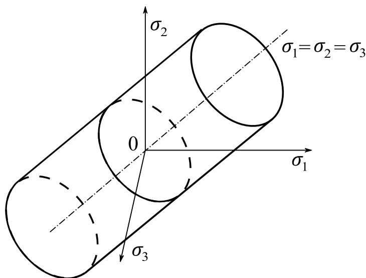
Obrázok 4.2: Plocha plasticity von Misesovej podmienky plasticity v priestore hlavných napätí [11].
