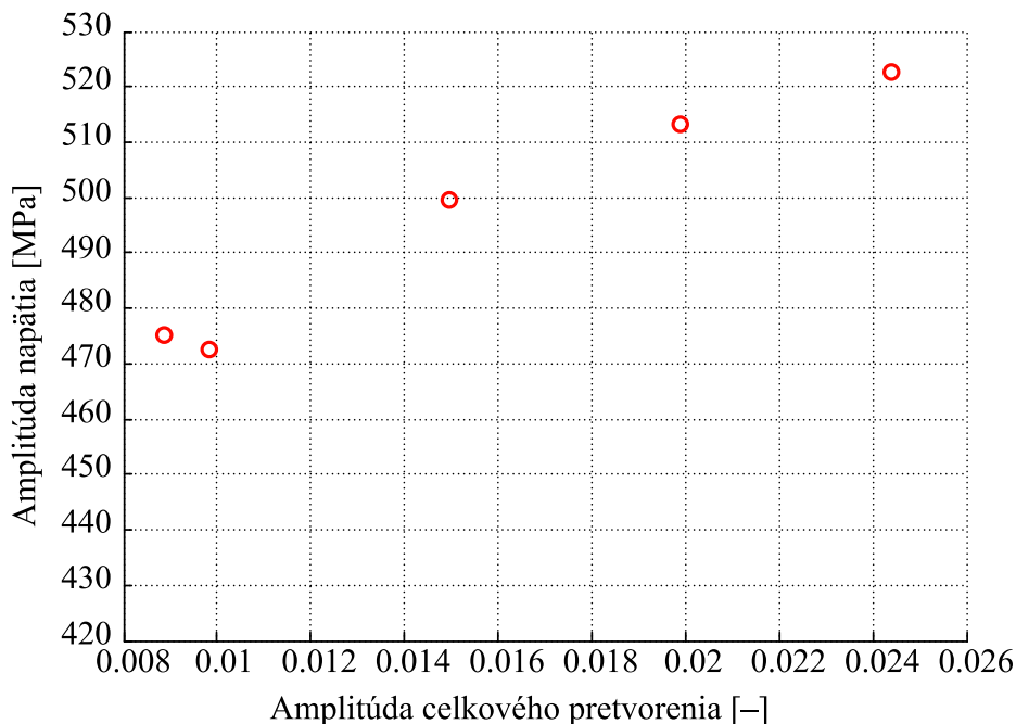
Obrázok 6.12: Vrcholové body saturovaných slučiek pre jednotlivé amplitúdy.
