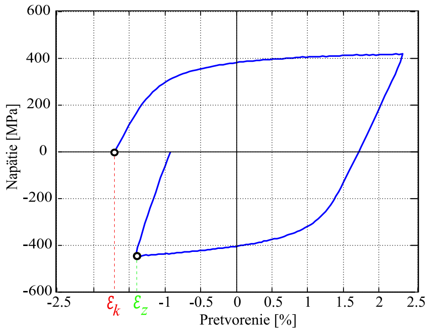
Obrázok 6.5: Znáznorenie polohy hodnôt pretvorenia \varepsilon_z a \varepsilon_k .
