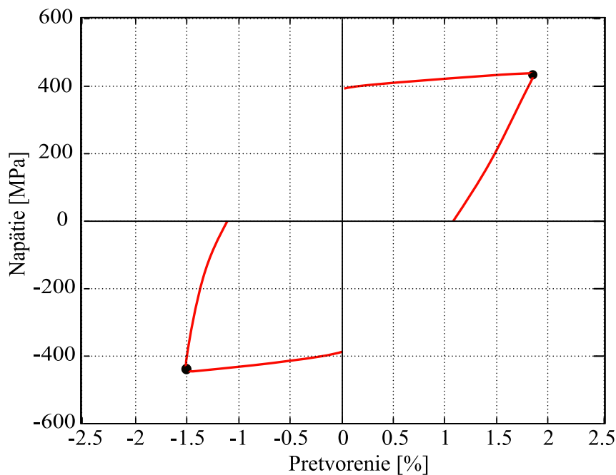
Obrázok 6.6: Oblasť hysteréznej slučky prehľadávaná nasledujúcou časťou algoritmu.
