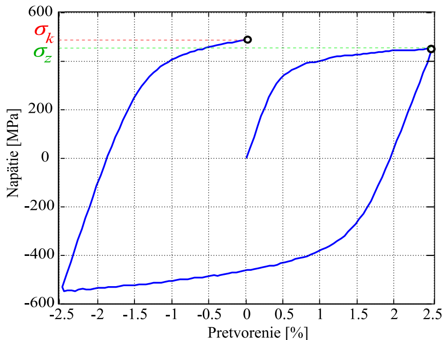
Obrázok 6.4: Znáznorenie polohy hodnôt napätia \sigma_k a \sigma_z .
