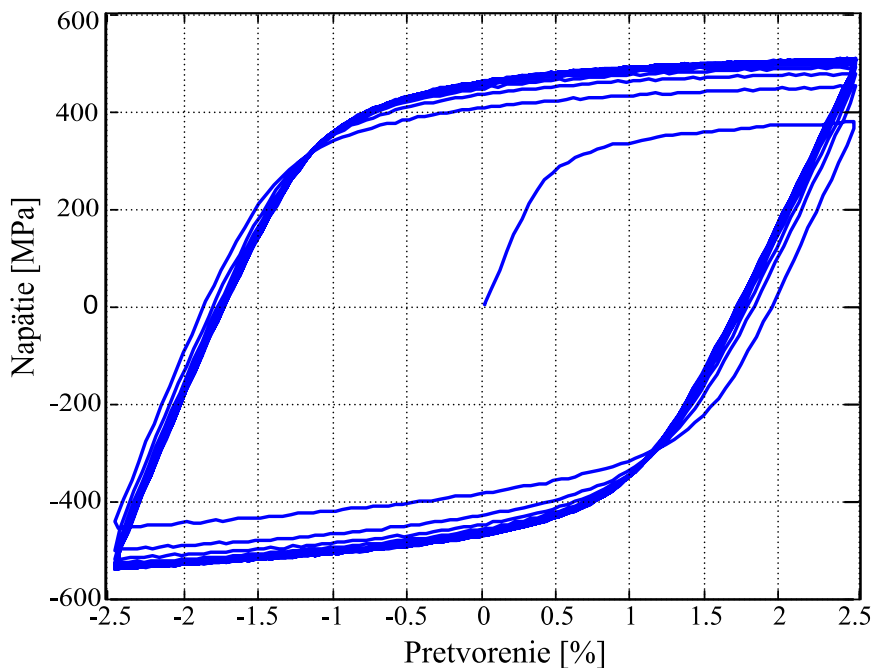
Obrázok 5.12: Postupná saturácia hysteréznej slučky.
