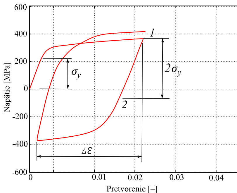
Obrázok 3.3: Znáročenie Bauschingerovho efektu [8].
