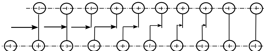
Obrázok 3.1: Posunutie vrstvy hranovou dislokáciou [5].
