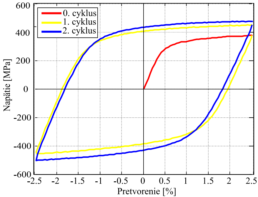
Obrázok 5.8: Číslovanie zaťažovacích cyklov začínajúce nulovým cyklom.
