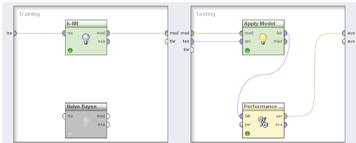
Obrázok 6.3 – Schéma krížovej validácie v programe RapidMiner
