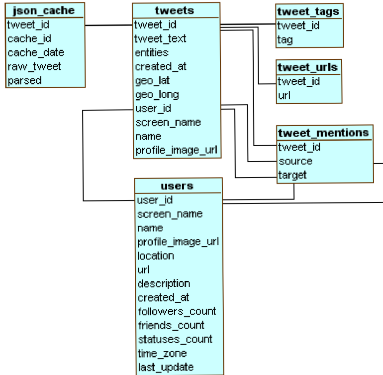
Obrázok 5.3 – databázova schéma frameworku 140dev [38]
