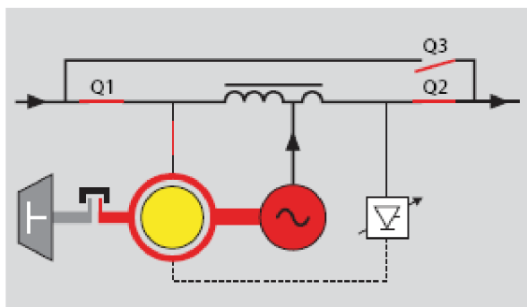
Obr. 4-3 Dynamický rotační zdroj - normální režim
