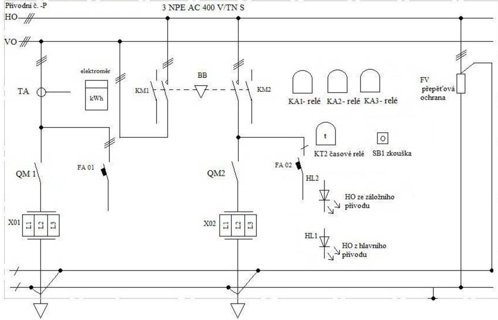
Obr. F-4 Sílový obvod přepínání napájení z hlavního obvodu
