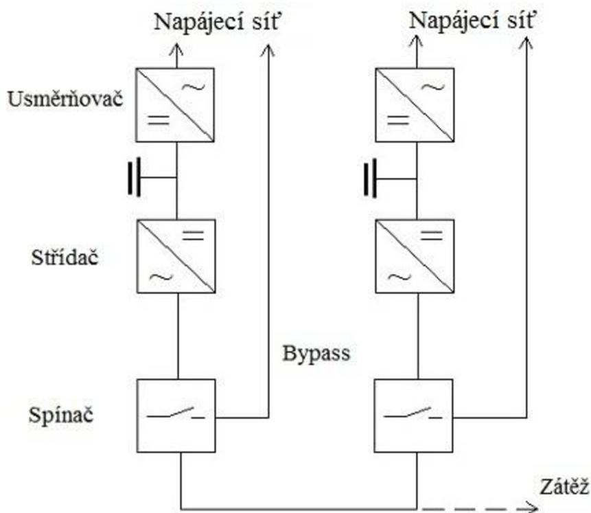
Obr. 3-2 Schéma paralelního zapojení UPS
