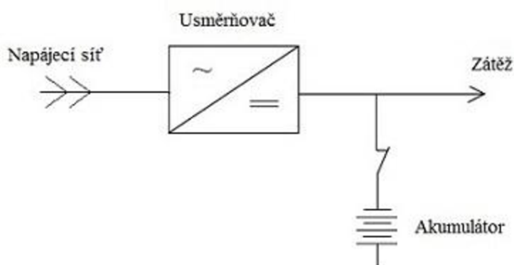
Obr. 3-1 Principiální schéma stejnosměrného náhradního zdroje
