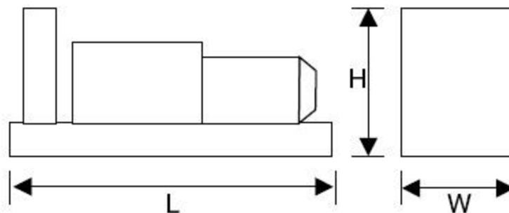
Obr. 6-4 Rozměry motorgenerátoru
