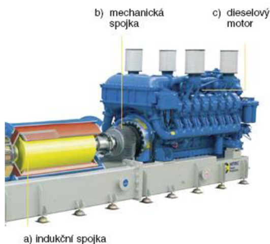
Obr. 4-2 Diesellový motor s mechanickou a indukční spojkou
