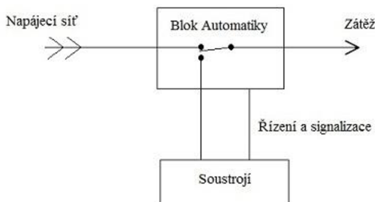
Obr. 4-1 Principiální schéma motorgenerátoru s blokem automatiky
