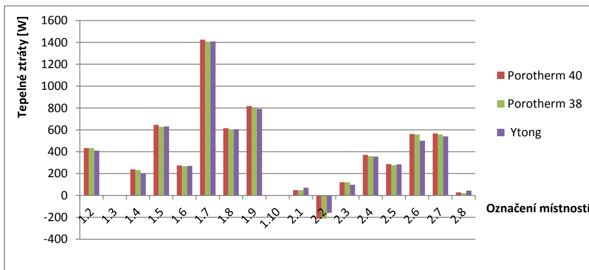
Obr. č. 15. Graf tepelné ztráty jednotlivých místností
