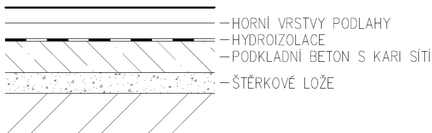
Obr. č. 11. Řez podlahou v přízemí
